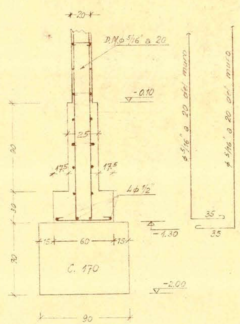
Sección 17÷17
