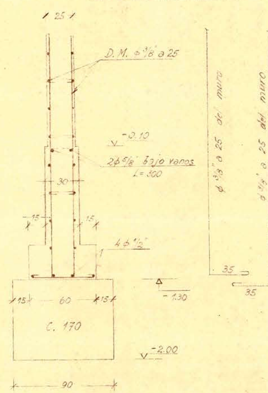
Sección 10÷10
