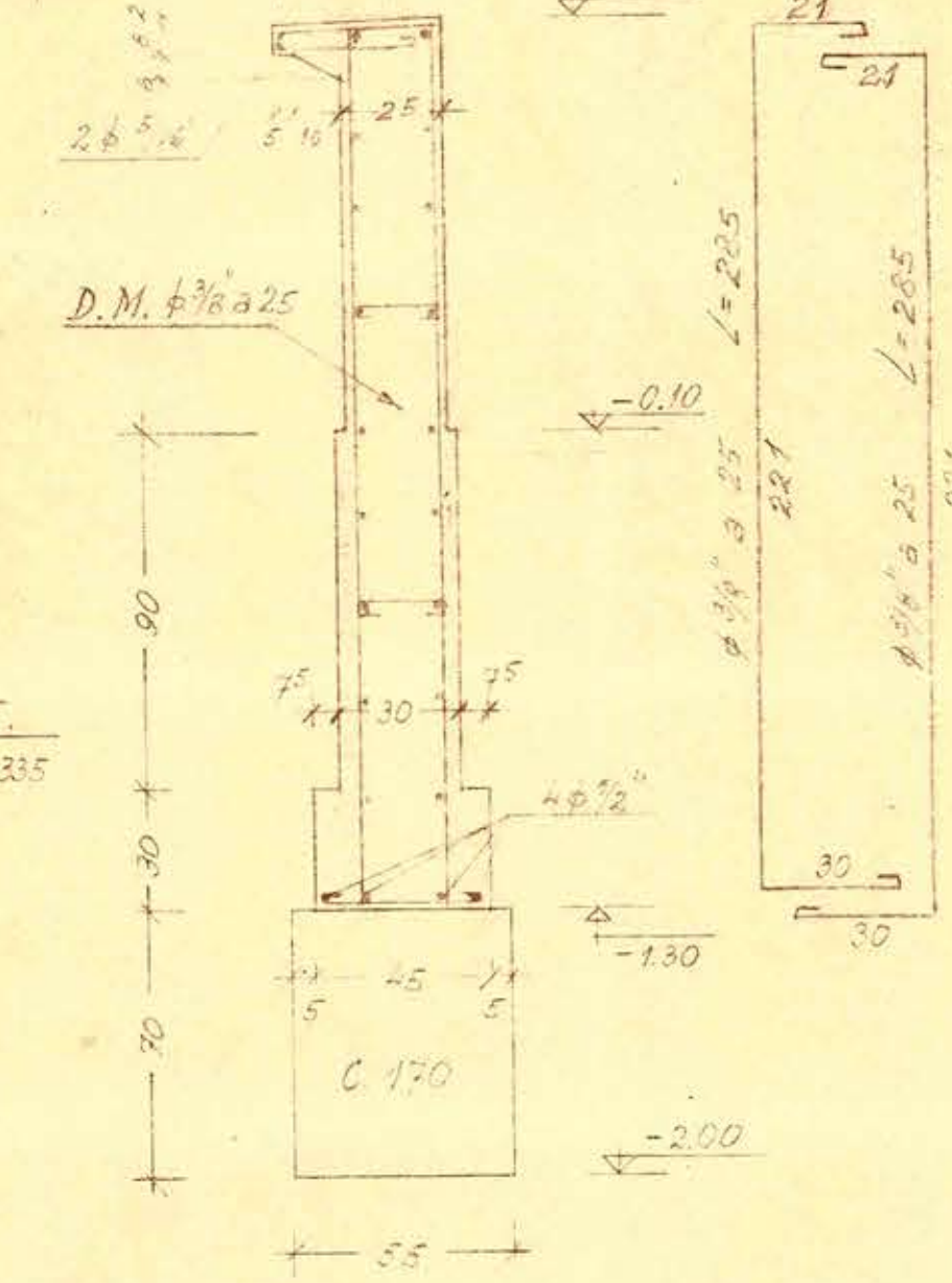
Sección 16÷16
