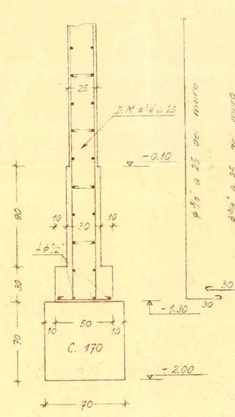
Sección 12÷12
