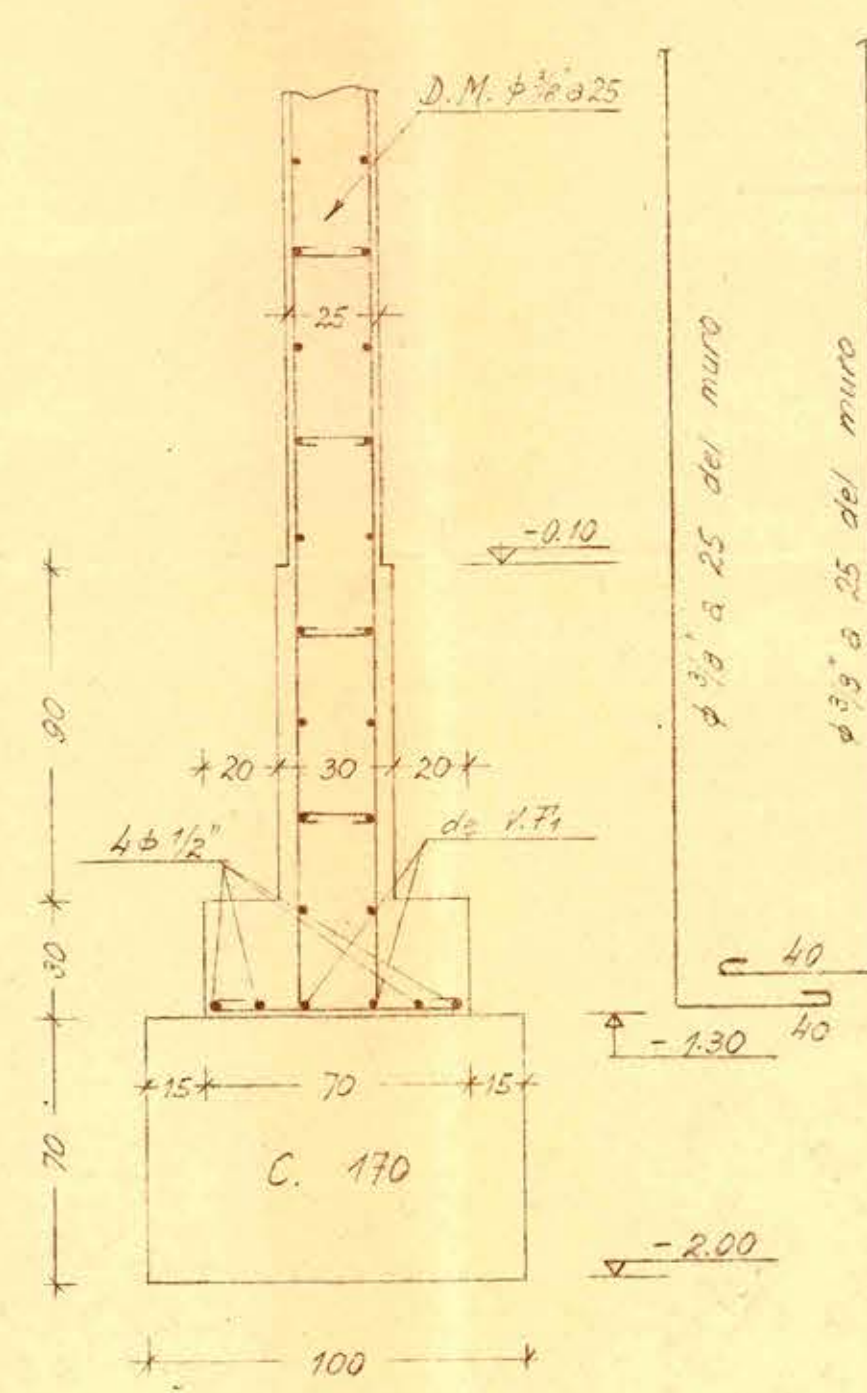
Sección 11÷11
