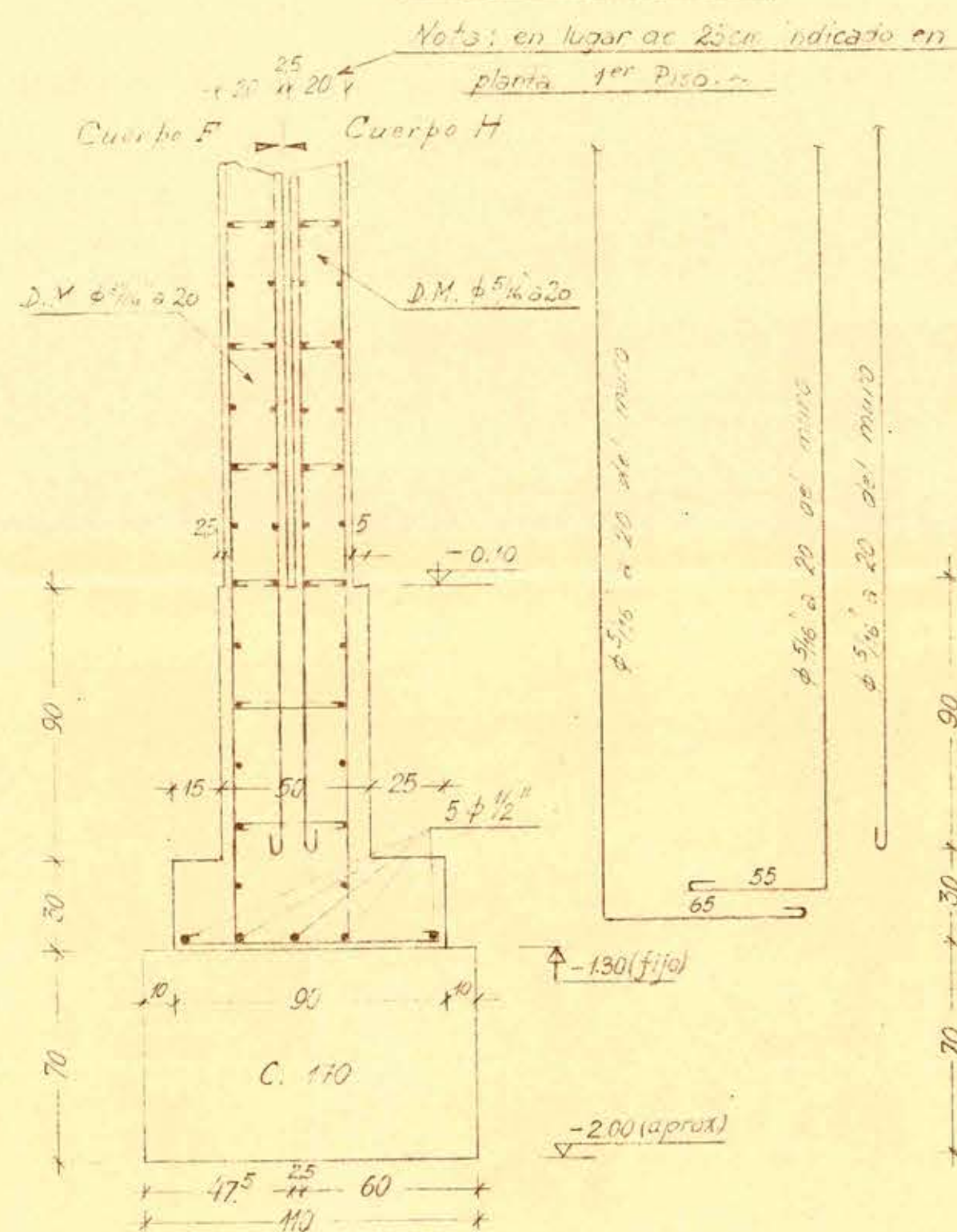
Sección 8÷8
