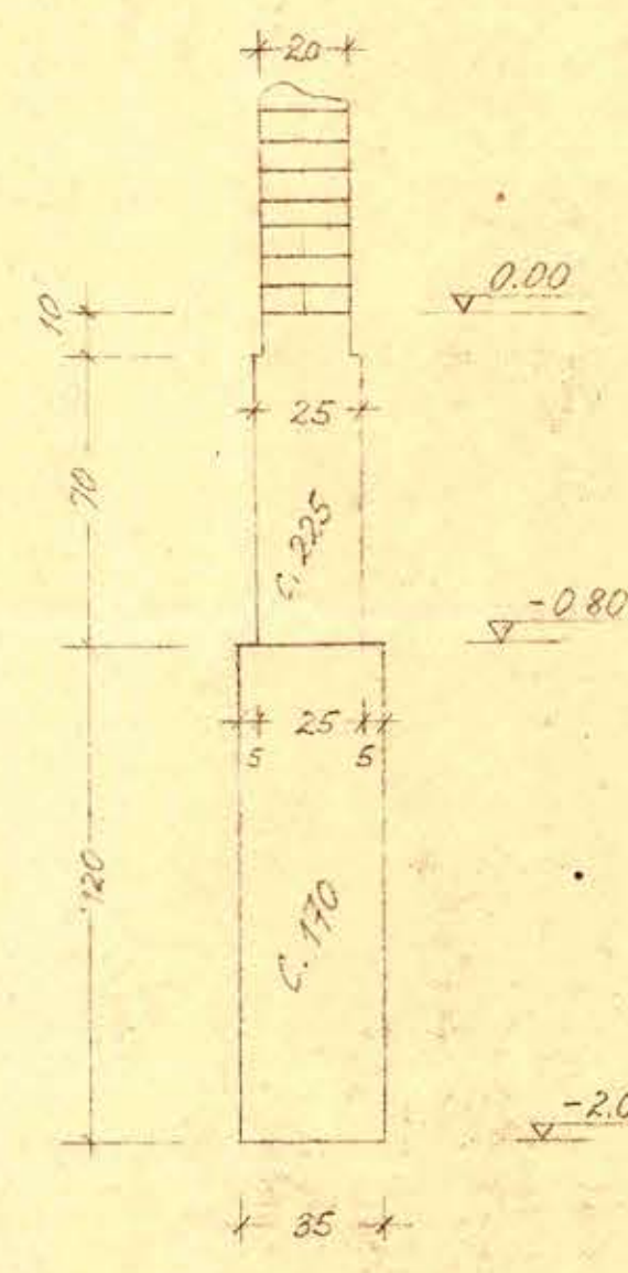
Sección 11÷11
