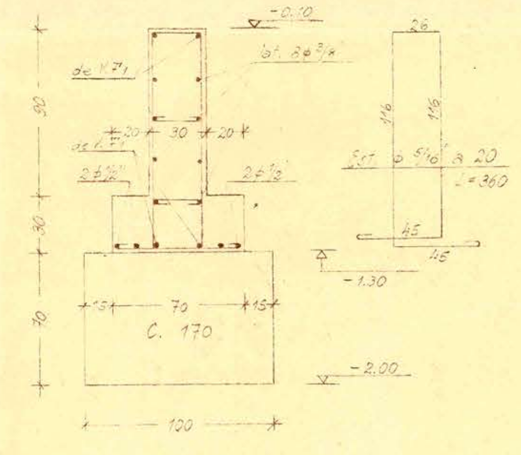
Sección 14÷14
