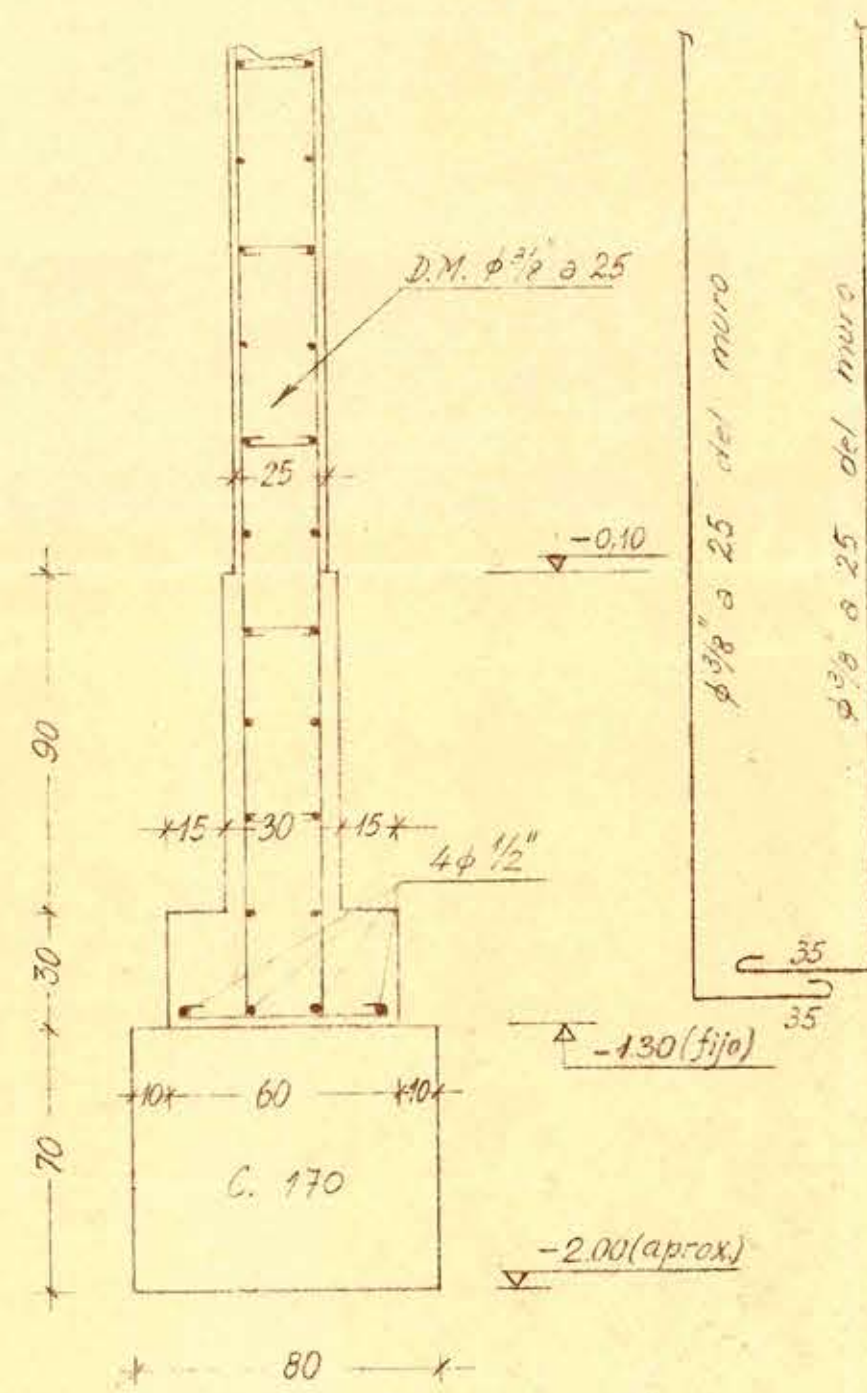
Sección 10÷10
