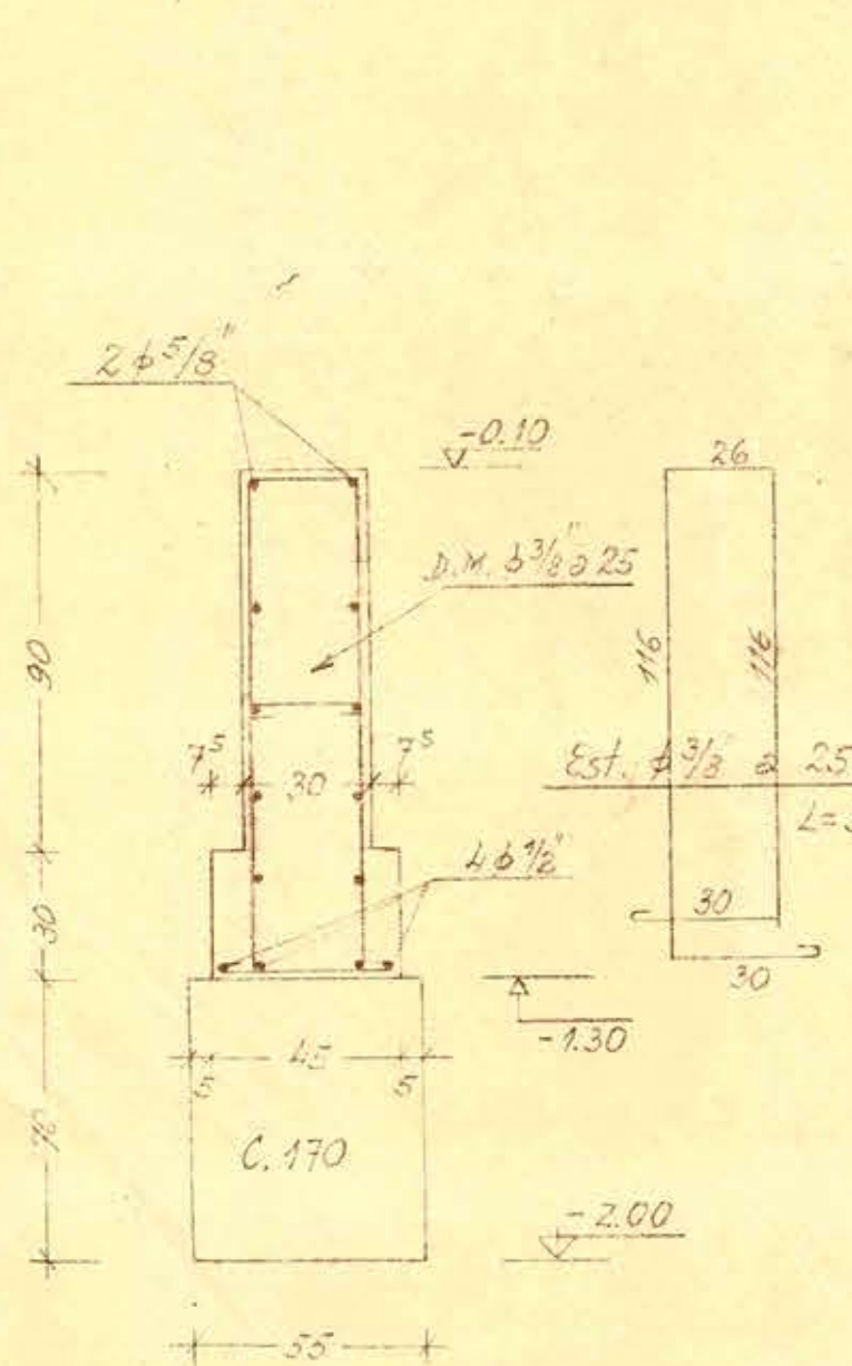
Sección 15÷15
