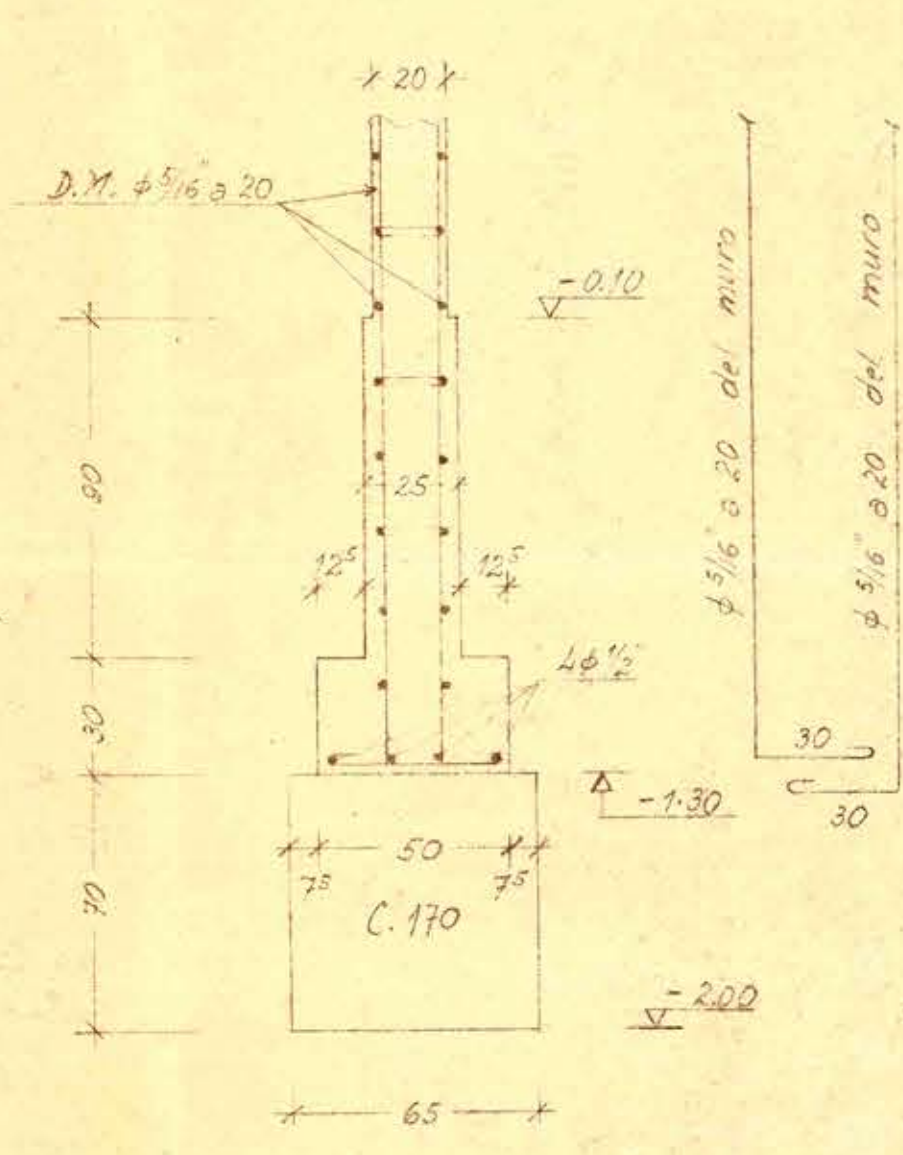
Sección 12÷12
