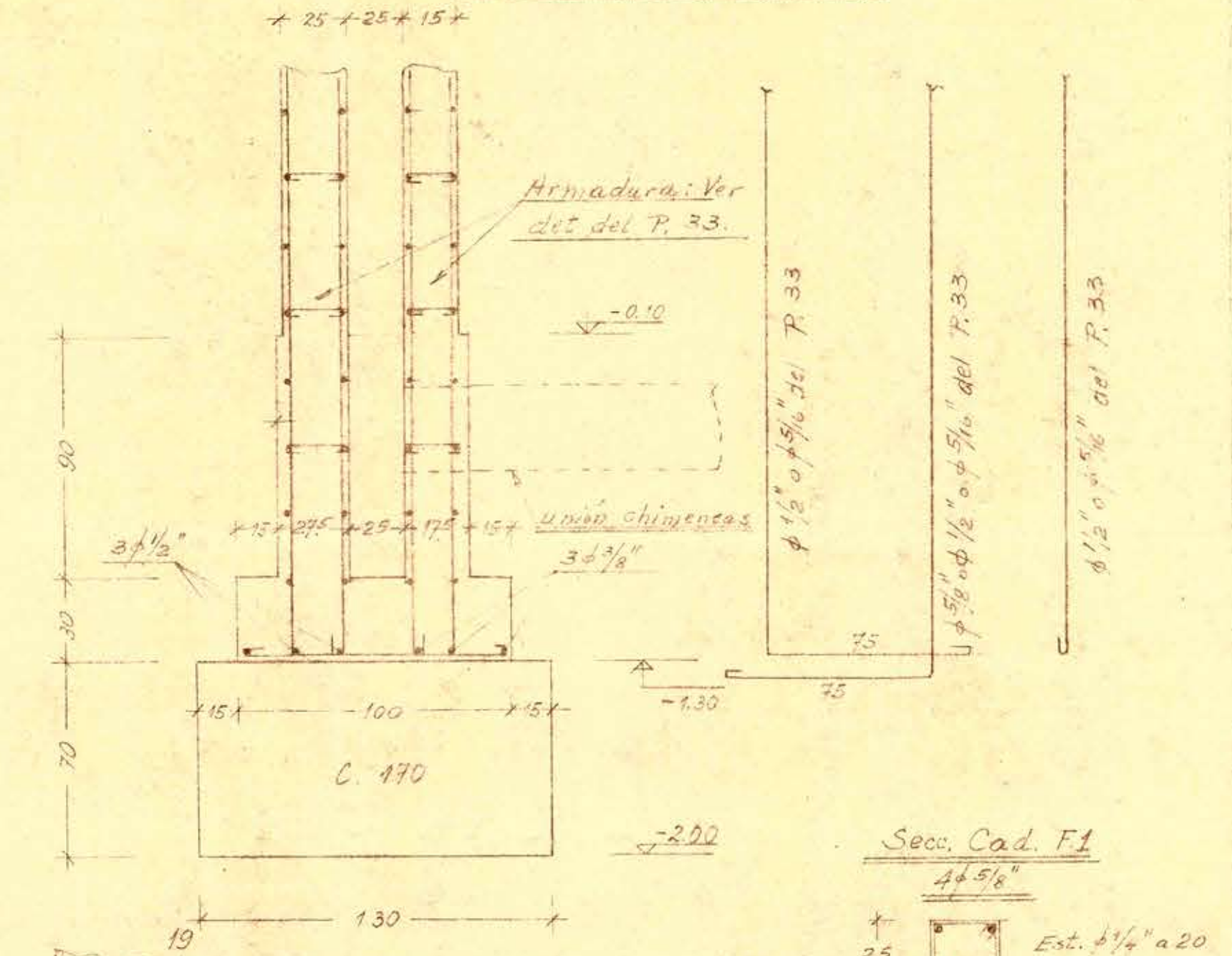
Sección 14÷14
