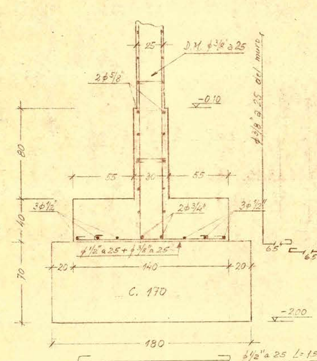
Sección 19÷19
