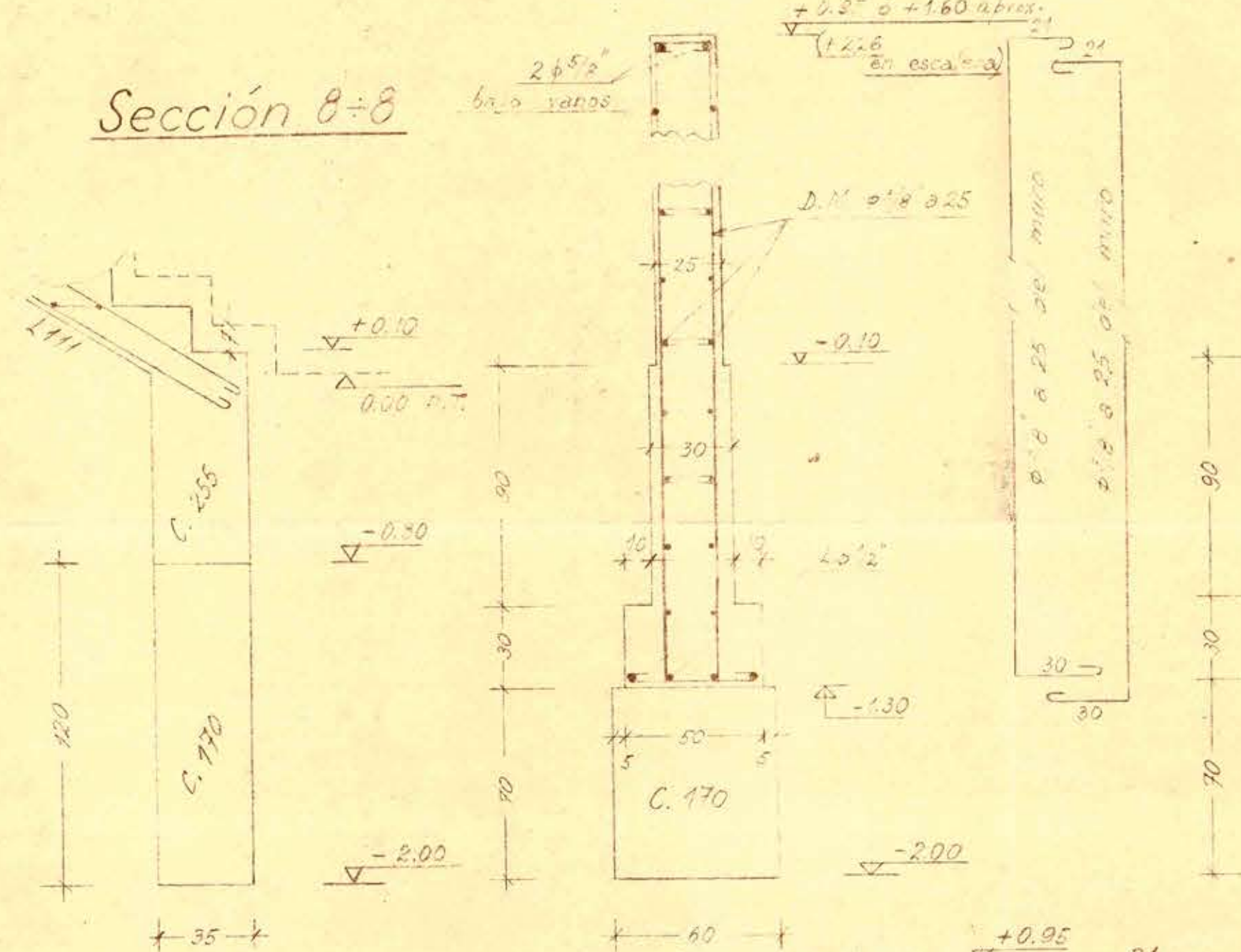
Sección 8÷8
