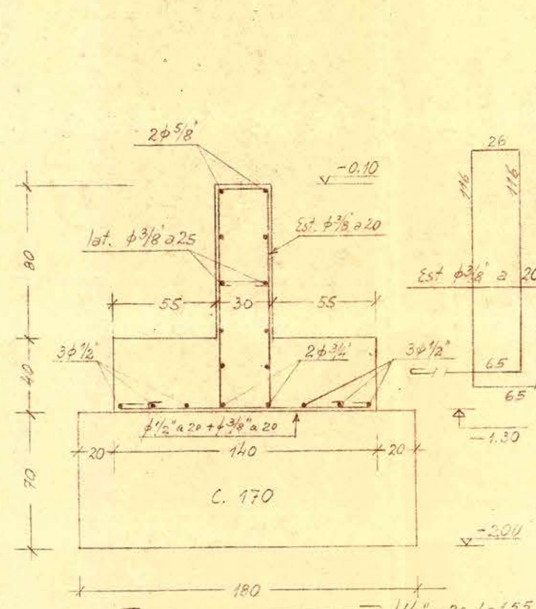
Sección 18÷18
