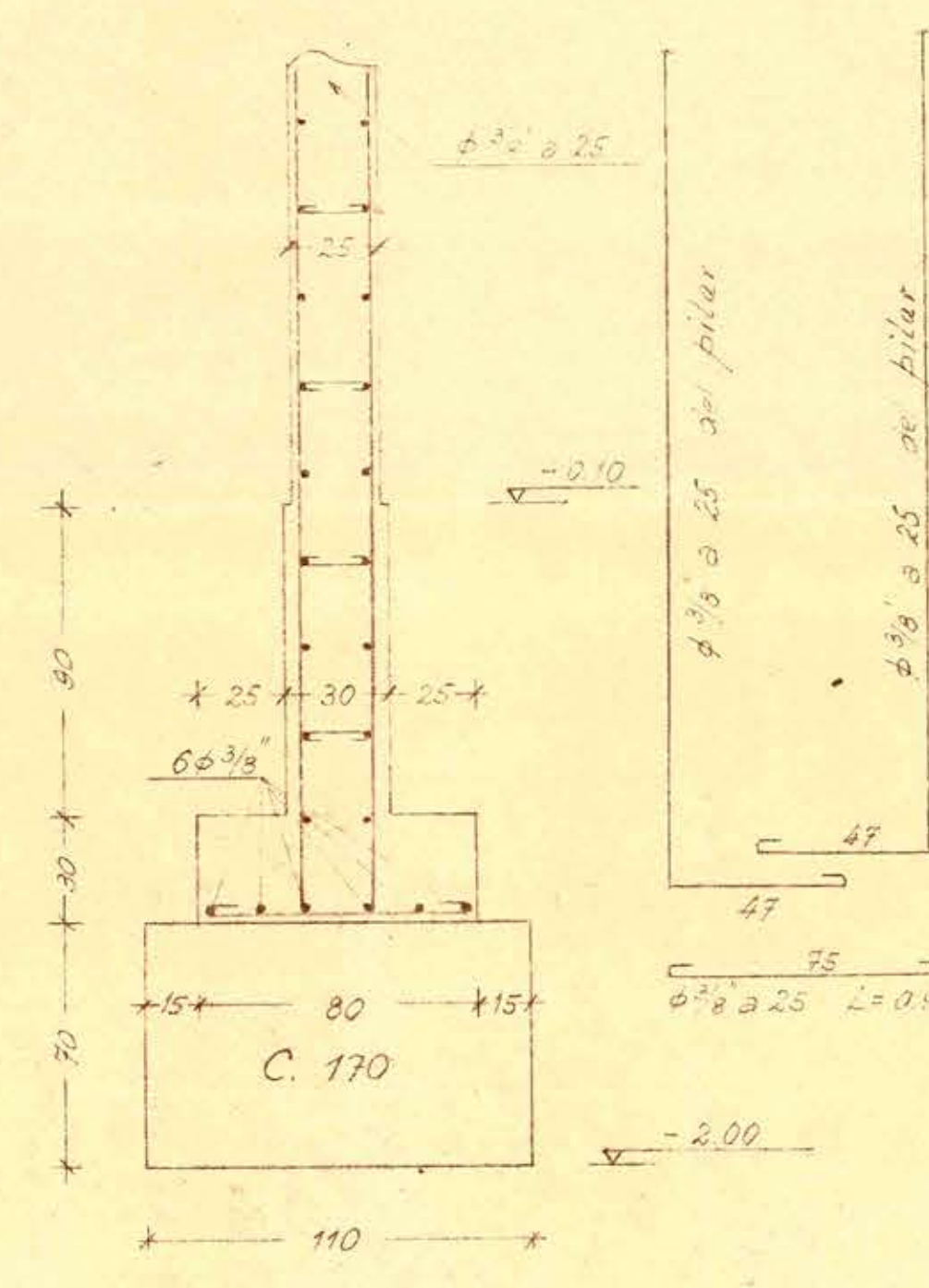
Sección 13÷13
