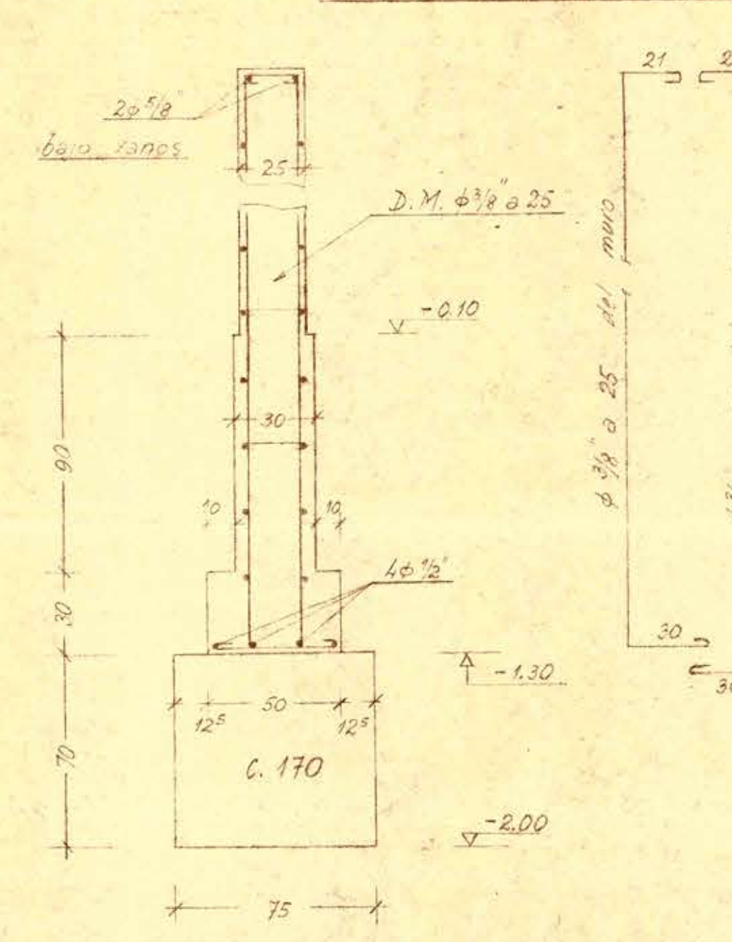
Sección 13÷13
