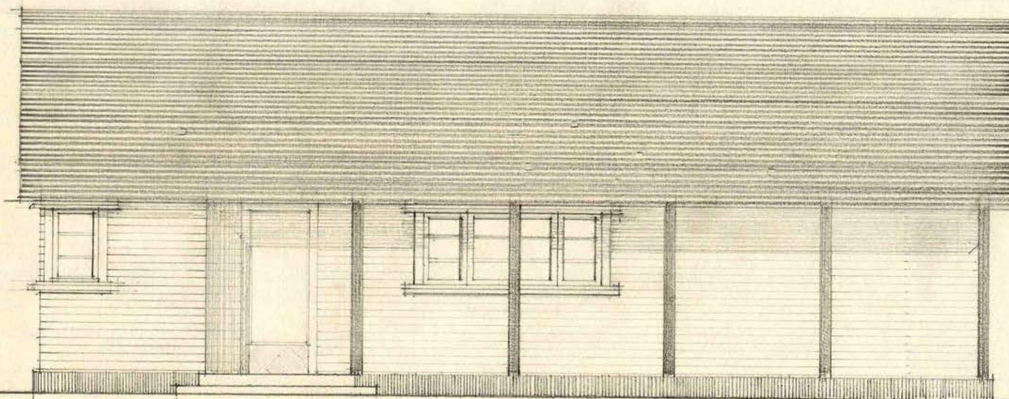
ELEVACION SUR
