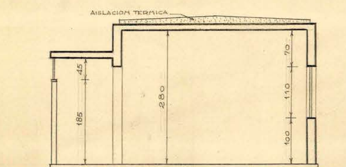
CORTE 3-3'
