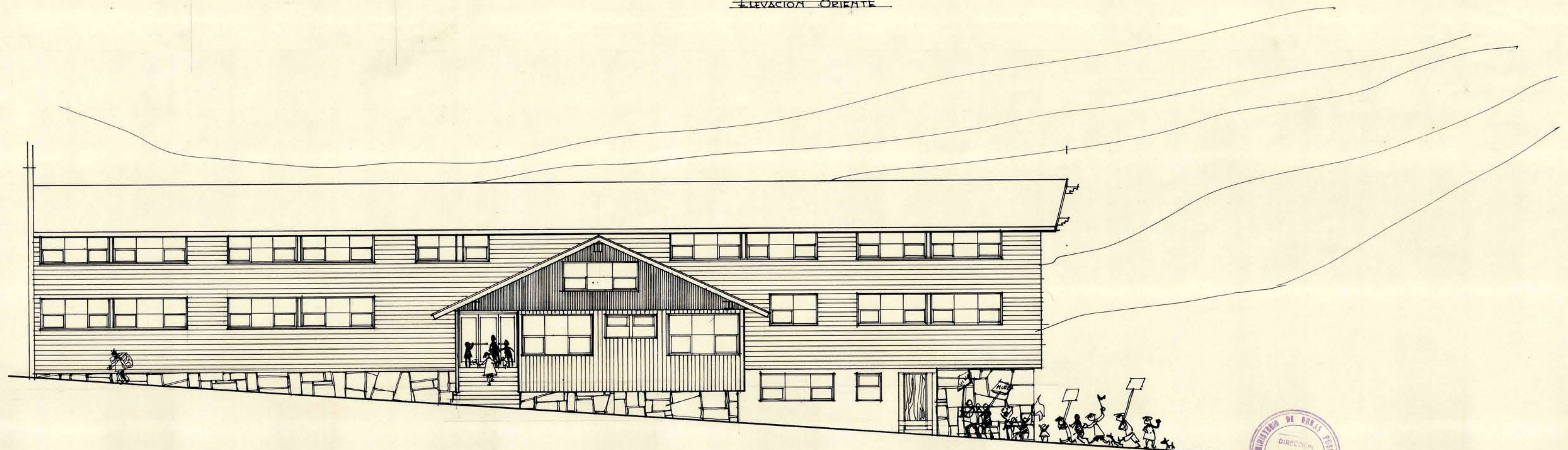
ELEVACION SUR
