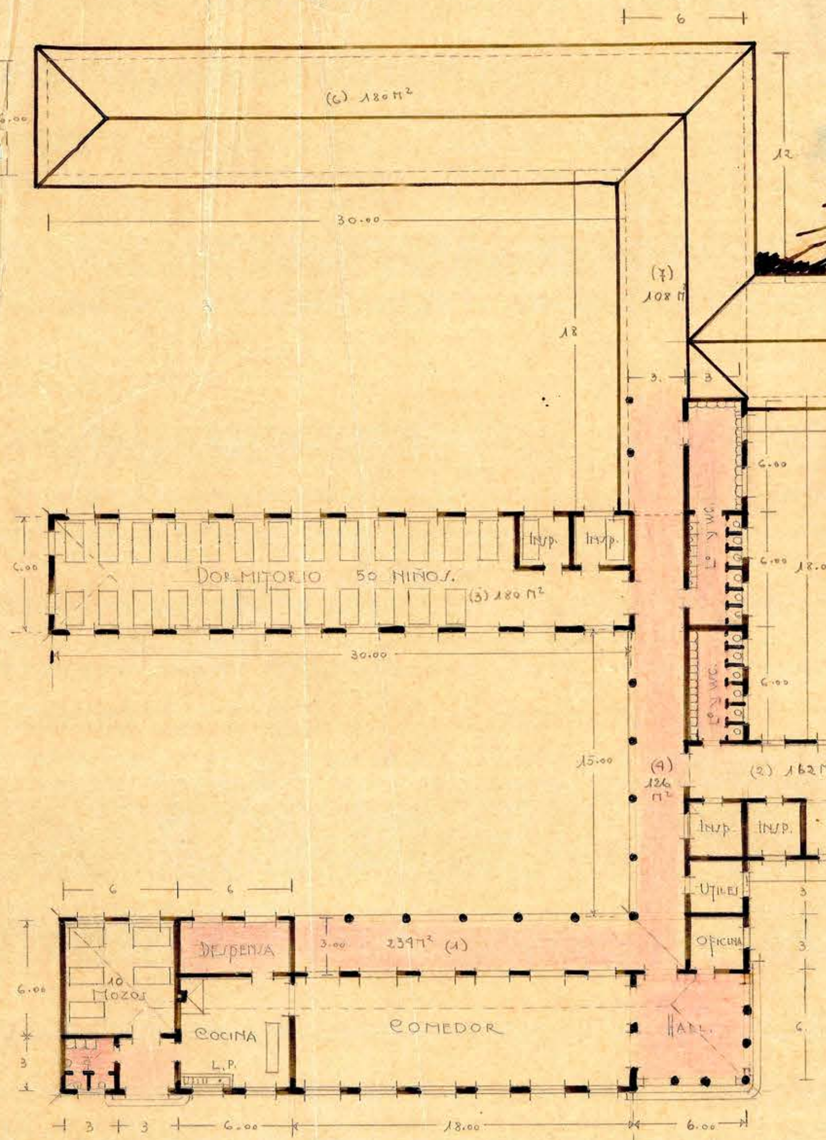
PLANTA. ESCALA: 0.05 P/MT.
