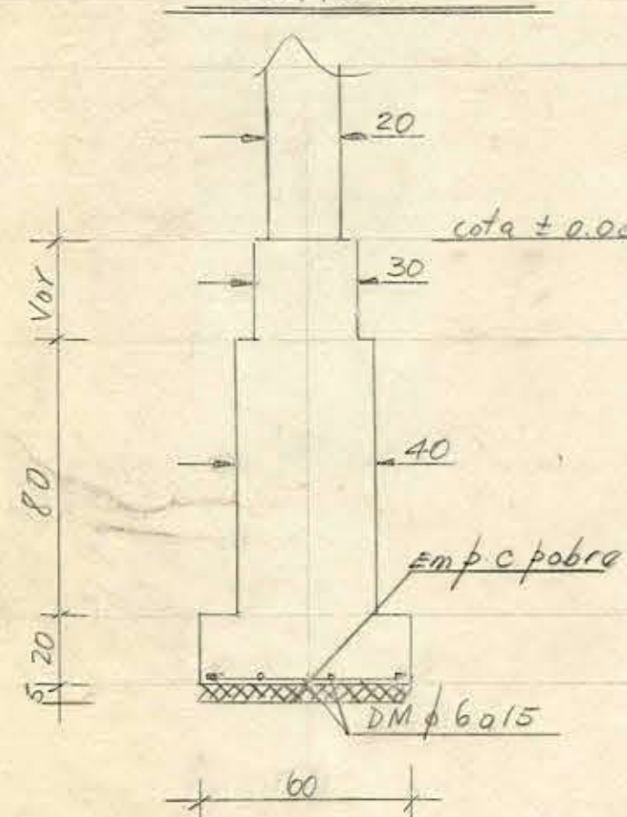
Corte A-A.
