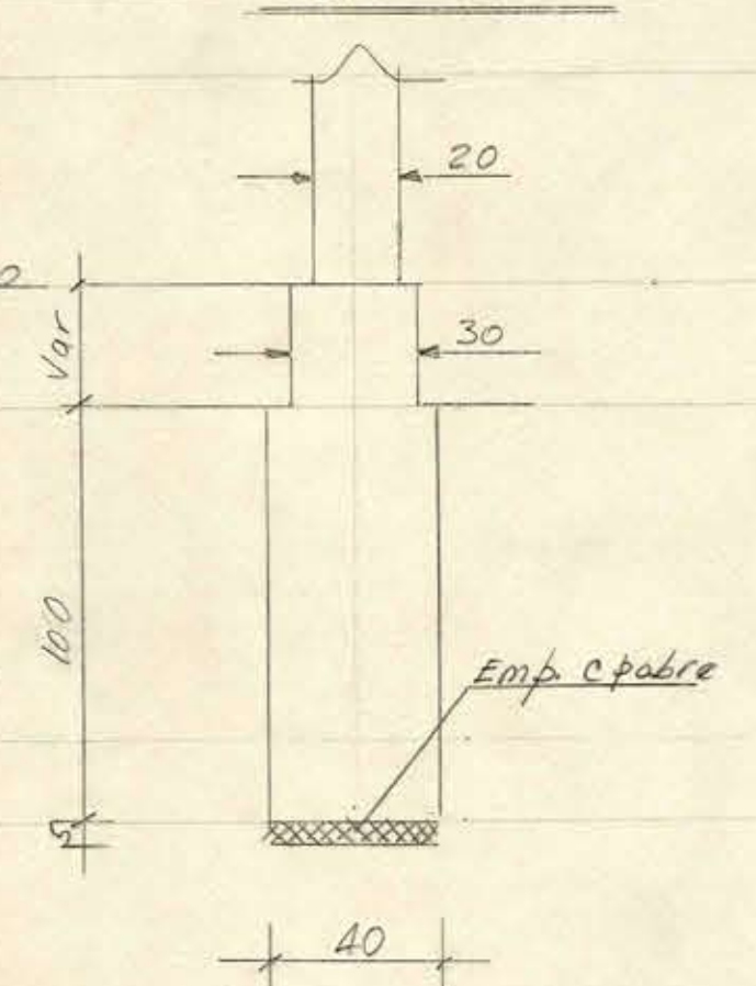
Corte B-B.
