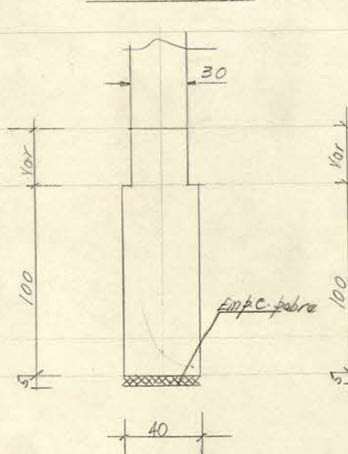
Corte C-C.
