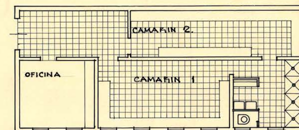
PLANTA CAMARINES Esc. 1:100
