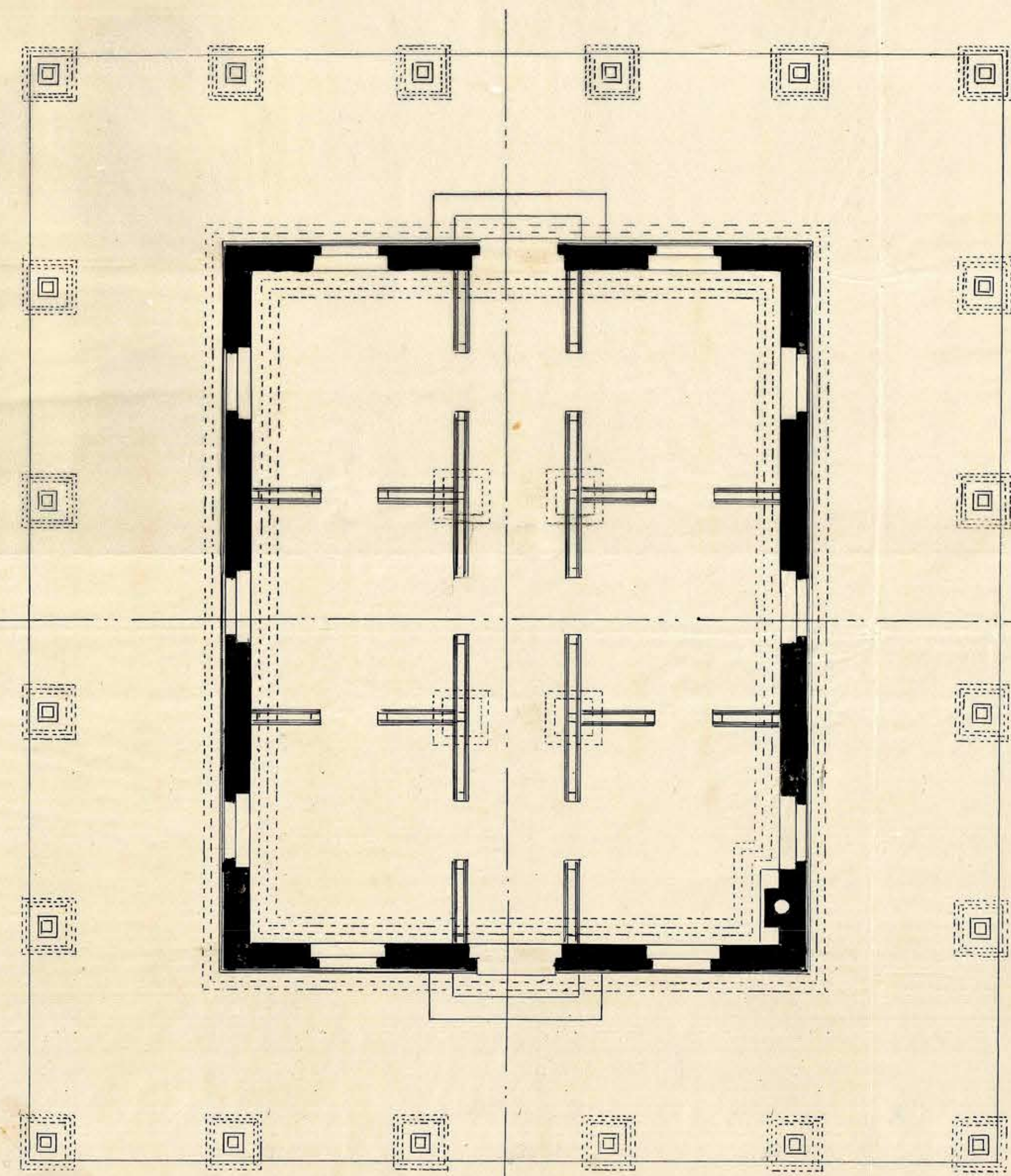
PLANO
