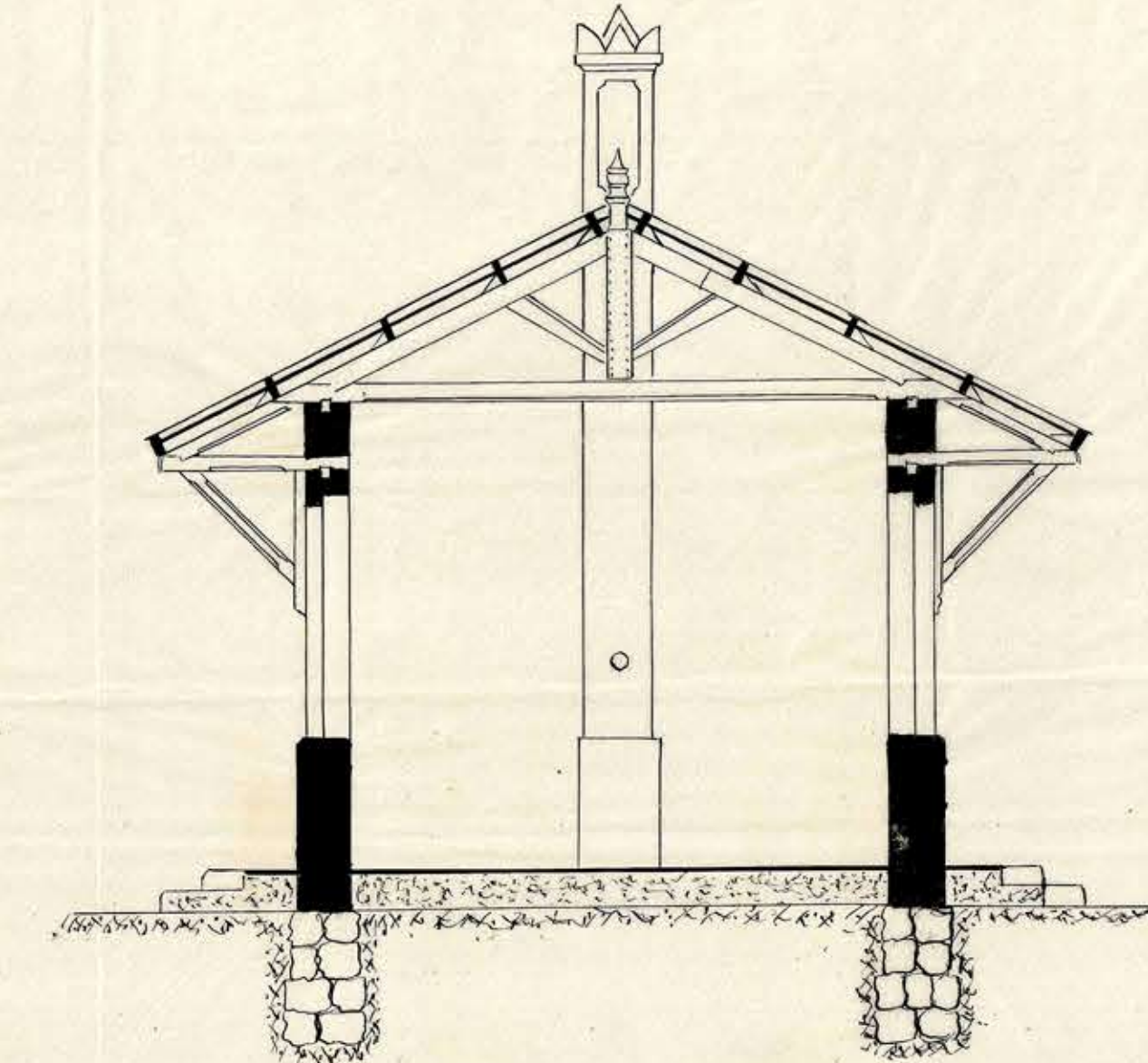
CORTE DE LA COCINA.
