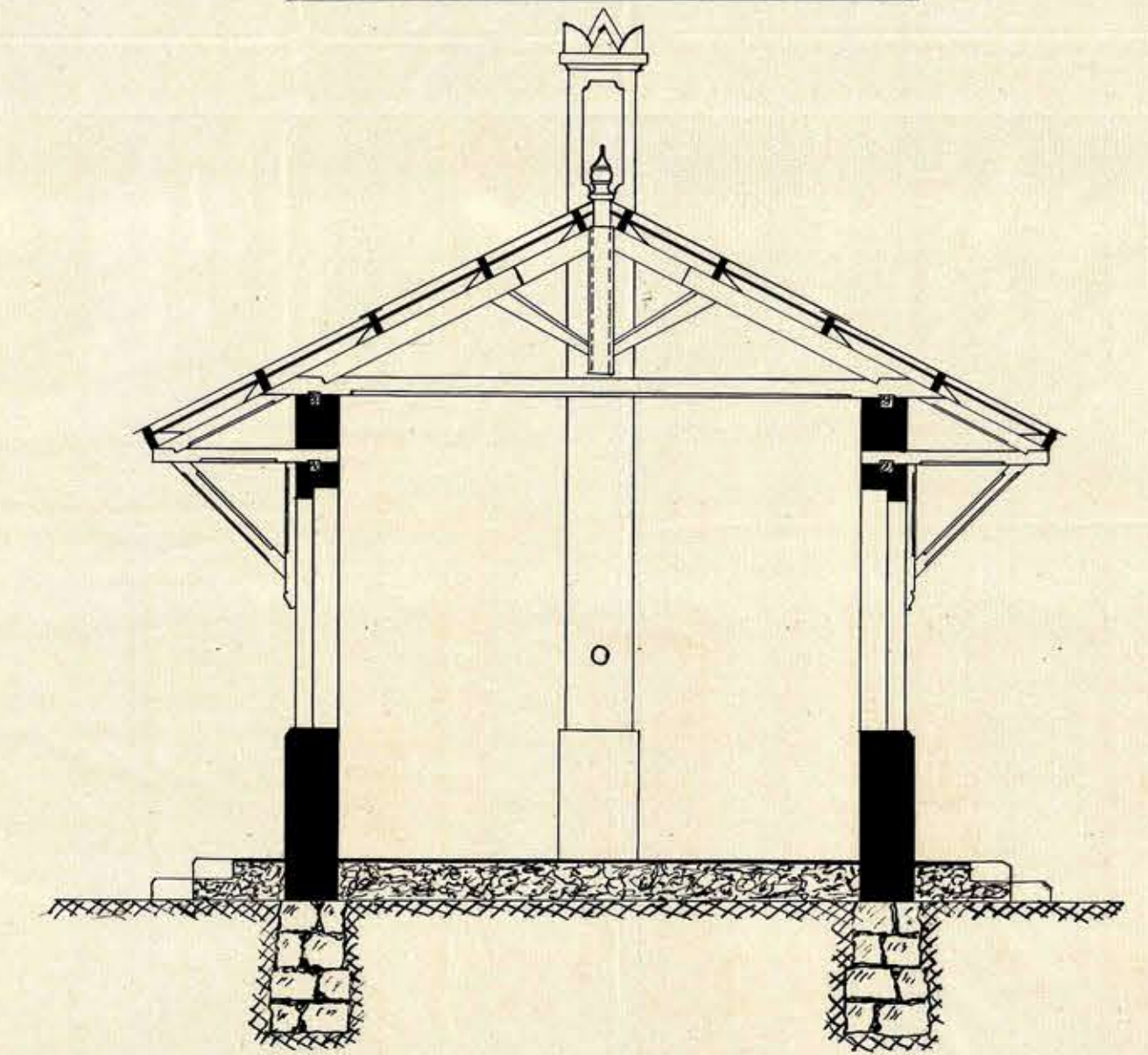
CORTE DE LA COCINA
