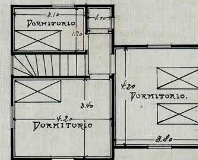
SEGUNDO PISO
