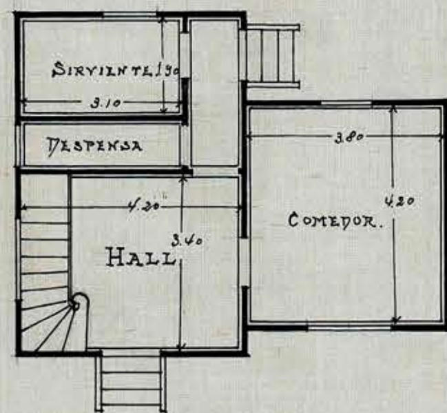
PRIMER PISO
