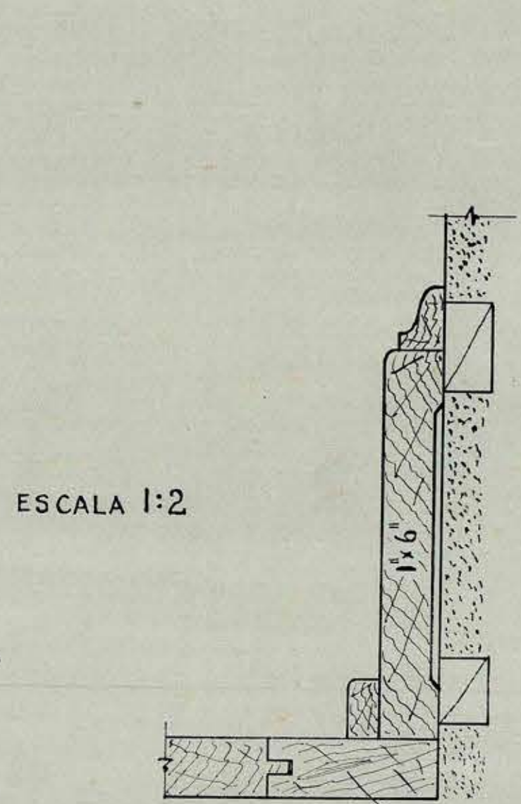
DETALLE DE LA TABLILLA PARA TIZA
