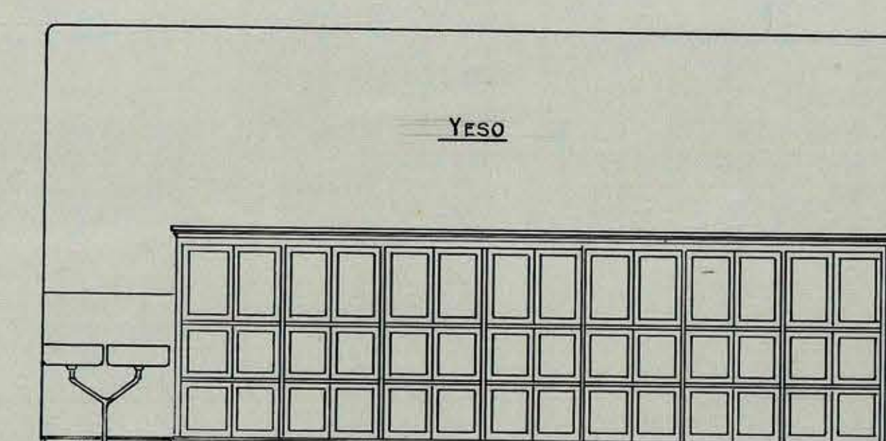
ELEVACION "C"
