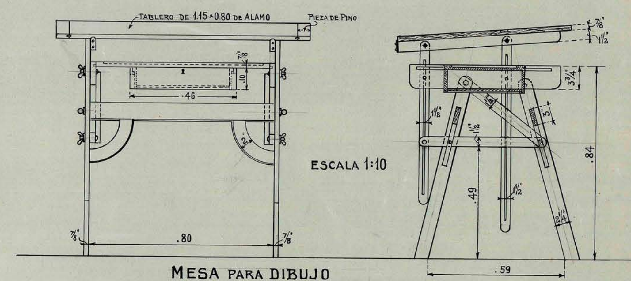
MESA PARA DIBUJO
