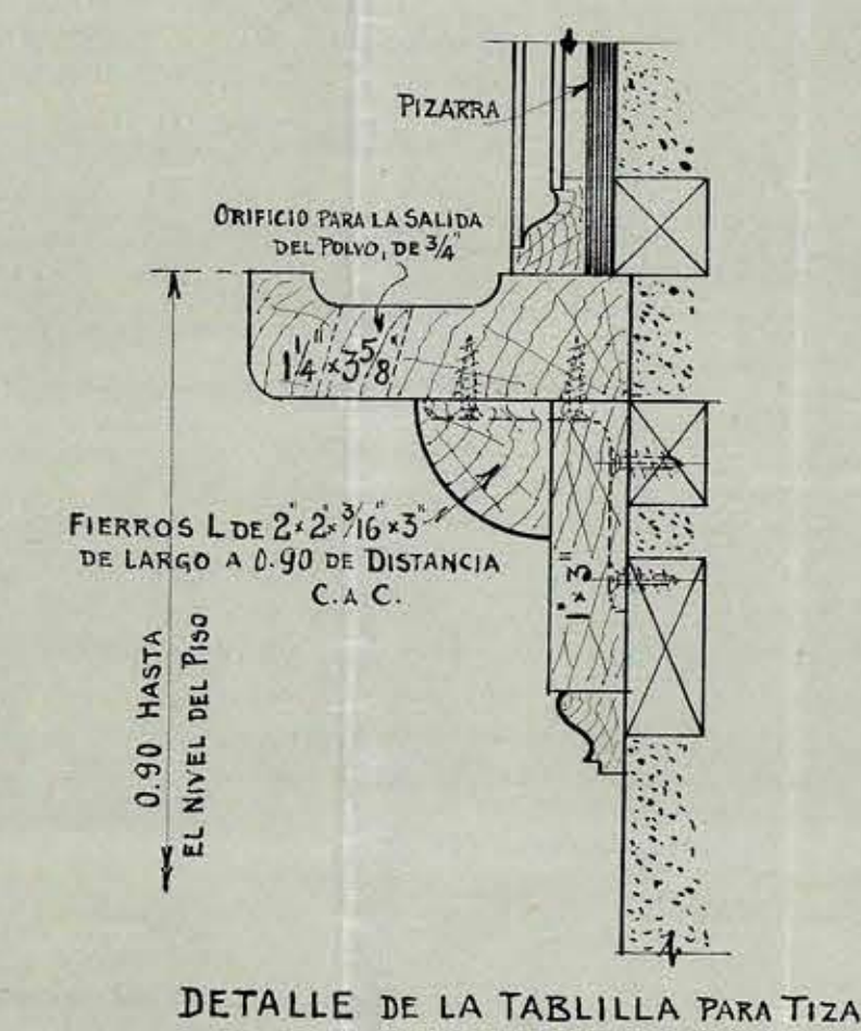
DETALLE DE LA TABLILLA PARA TIZA
