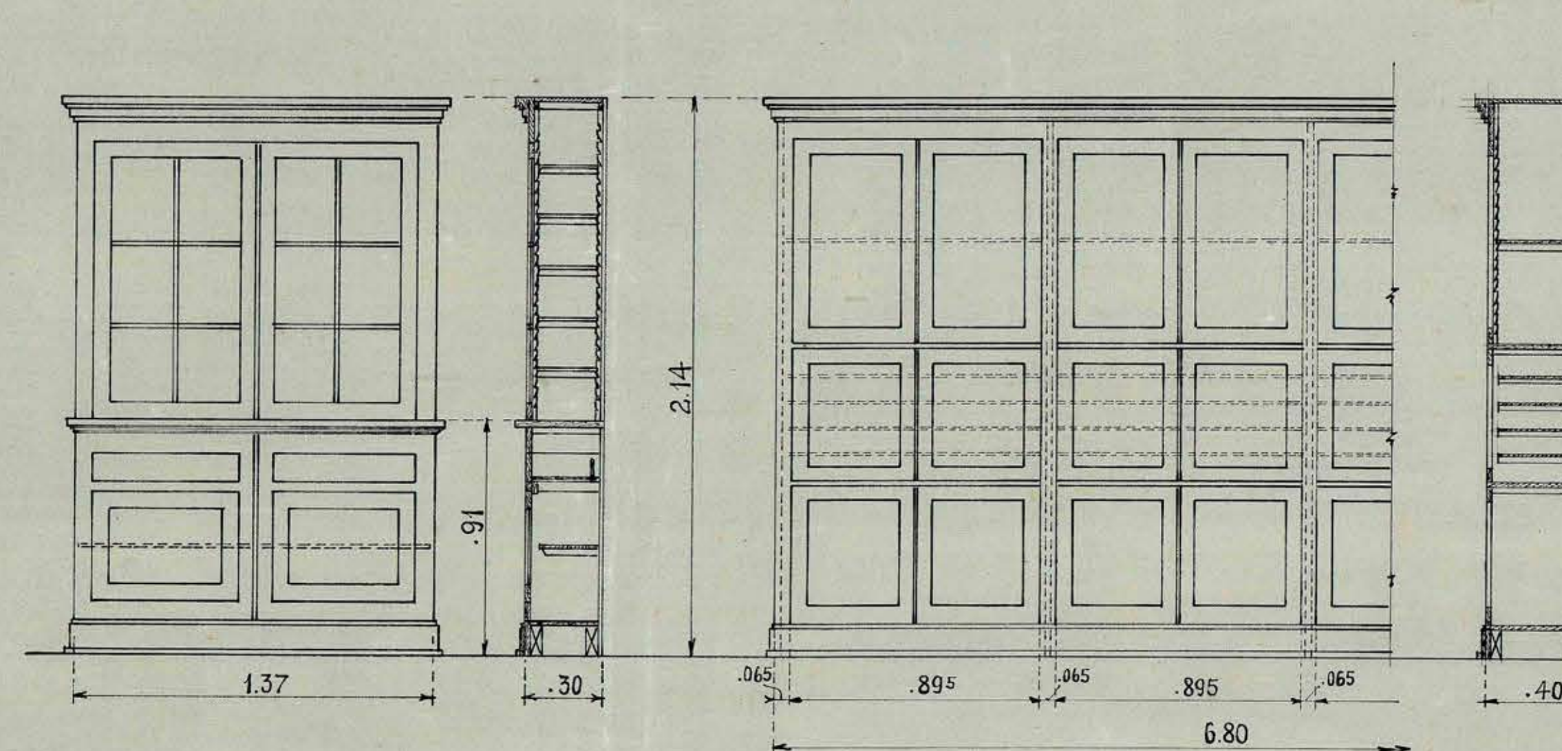
ESTANTE PARA LIBROS
