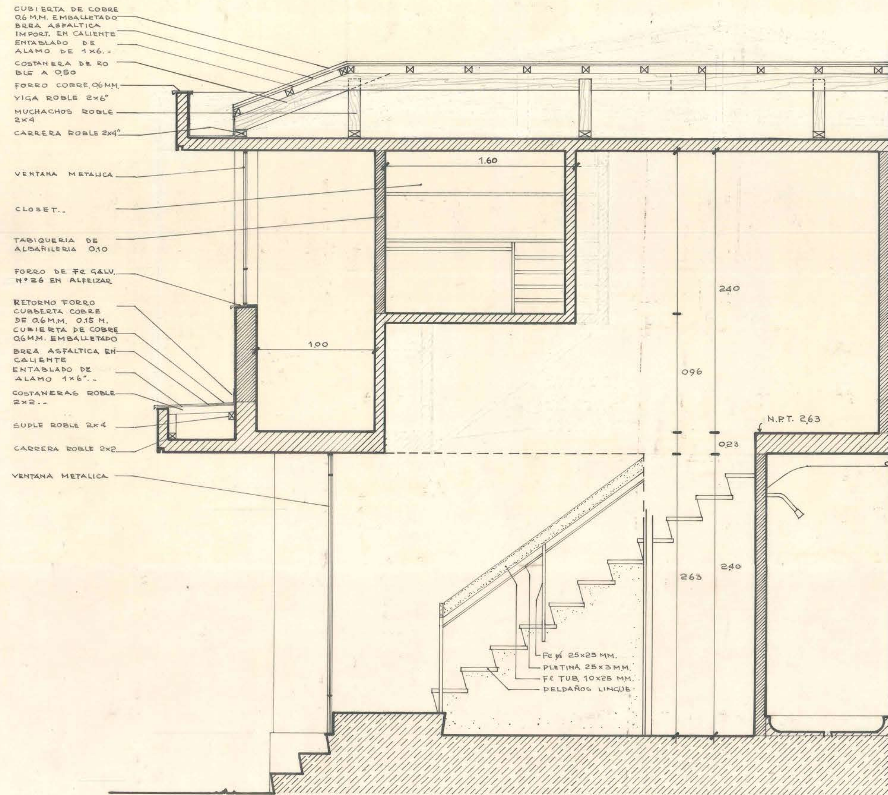
CORTE 1-1
