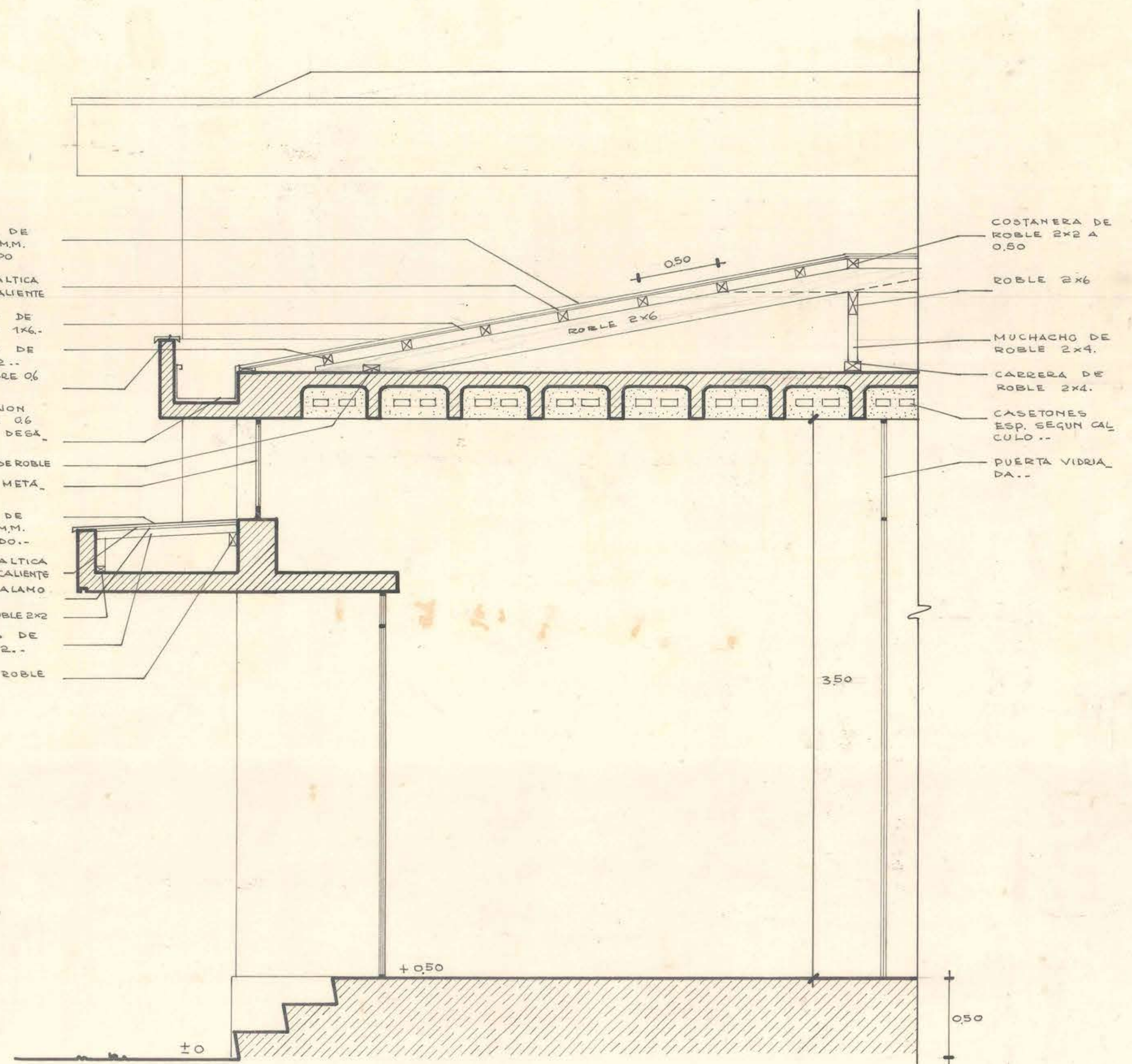
CORTE 2-2
