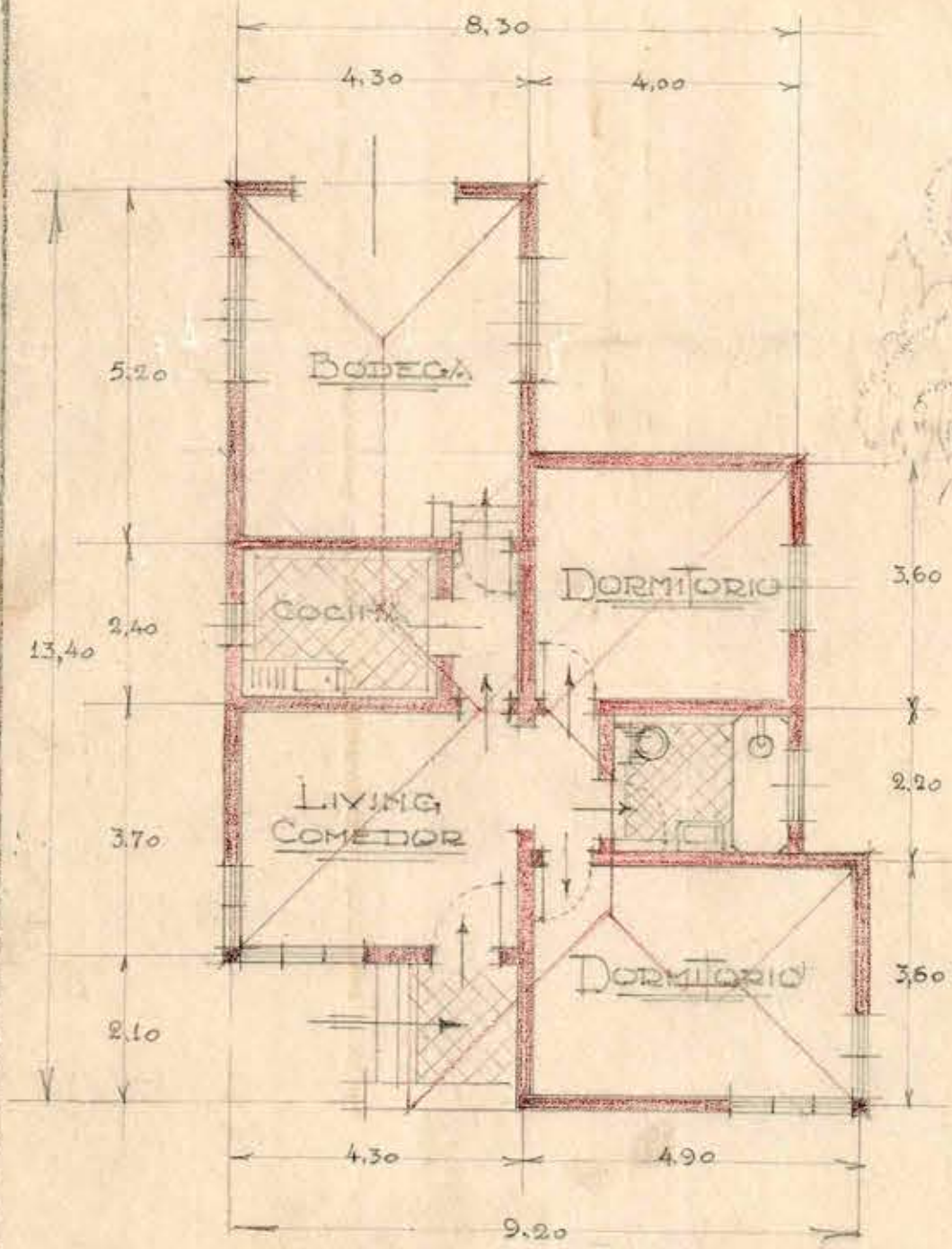
CASA PARA GUARDA HILOS EN PLACILLA - VALPARAISO - PLANTA Y FACHADAS - ESCALA 1:100 - D.G. de O.P. - DEPTO. ARQV. - 1937
