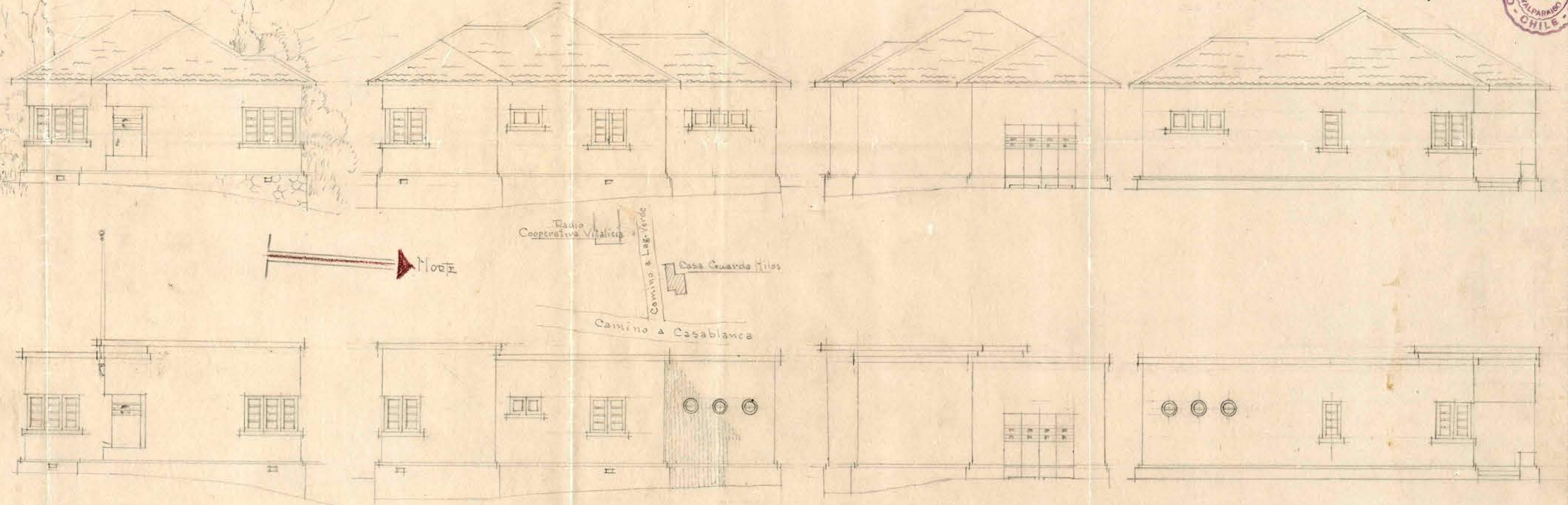
CASA PARA GUARDA HILOS EN PLACILLA - VALPARAISO - PLANTA Y FACHADAS - ESCALA 1:100 - D.G. de O.P. - DEPTO. ARQV. - 1937
