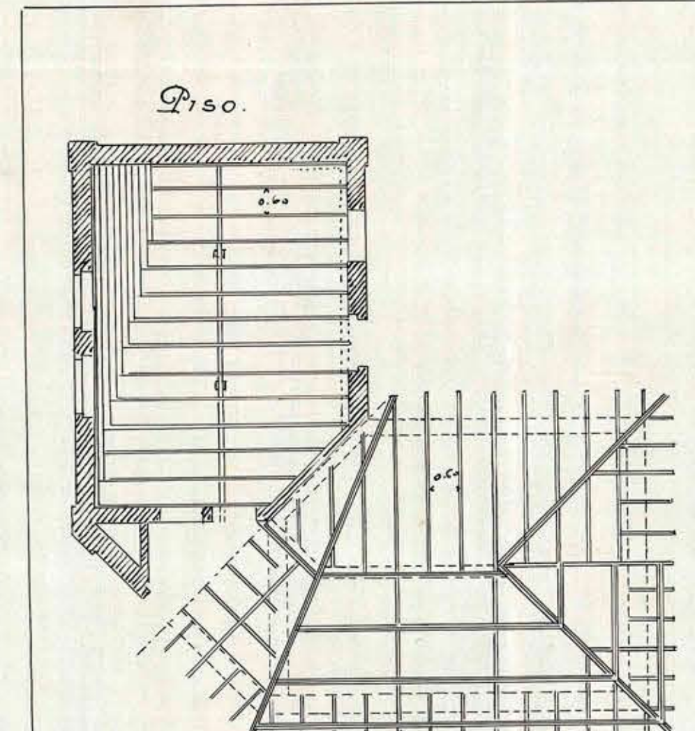
— Techumbre. —
