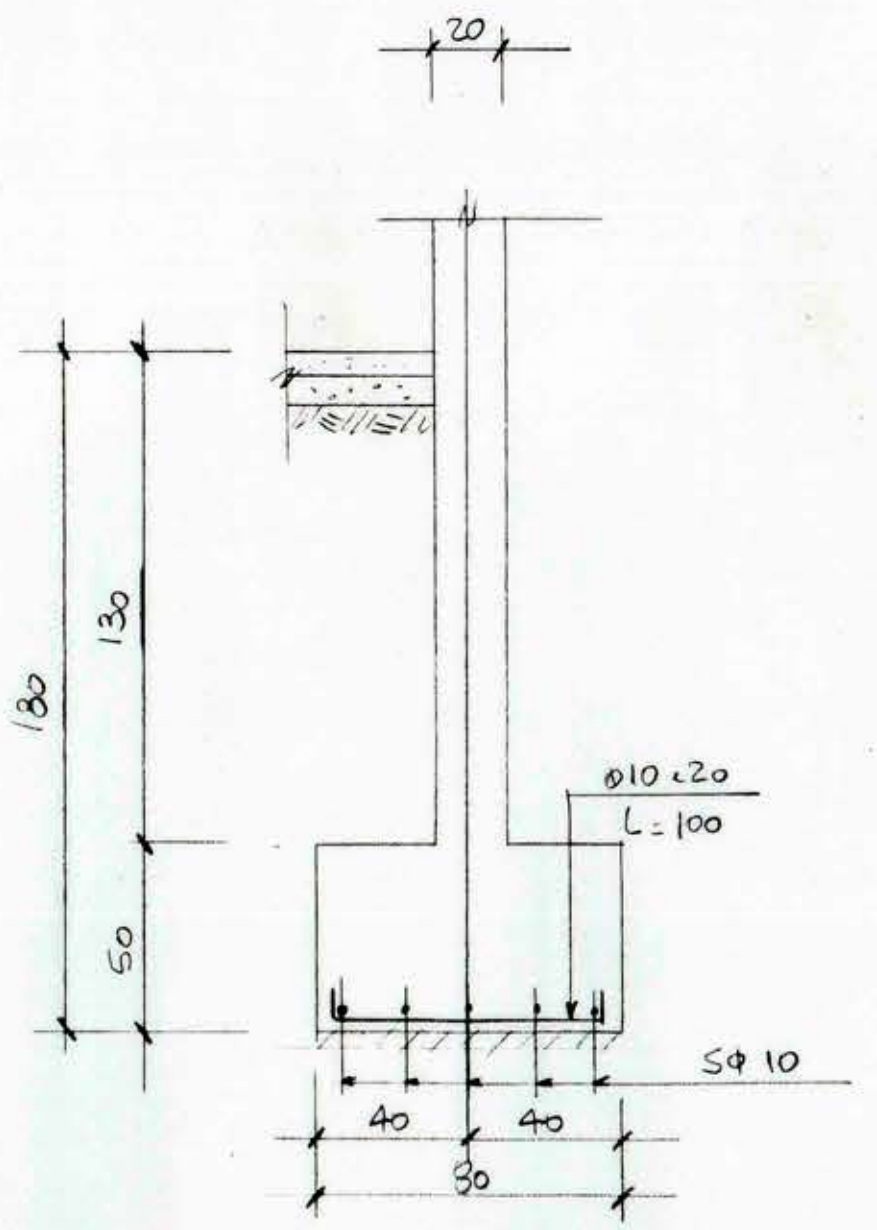
SECCION F1 φ80/150
