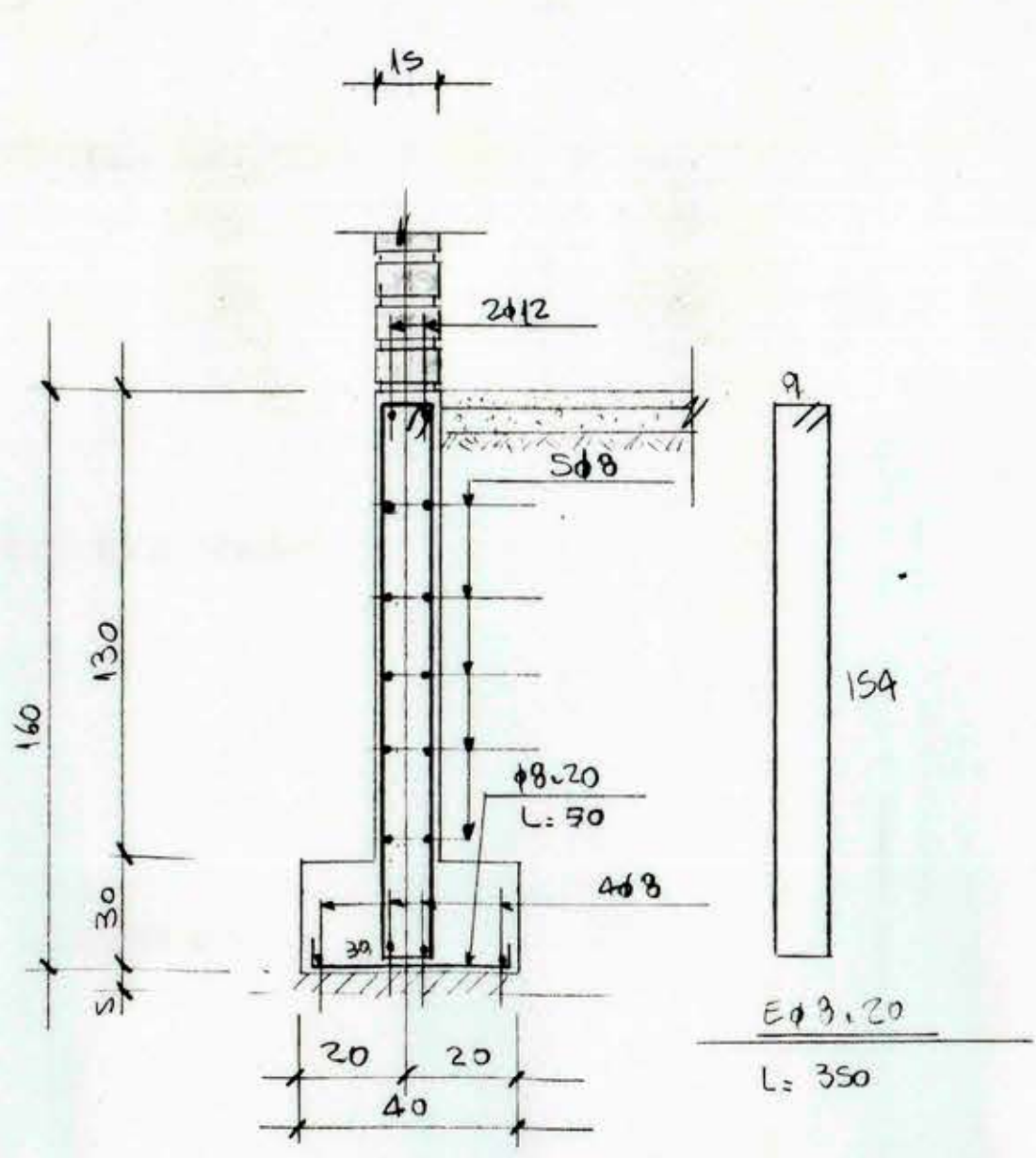
SECCION A-A
