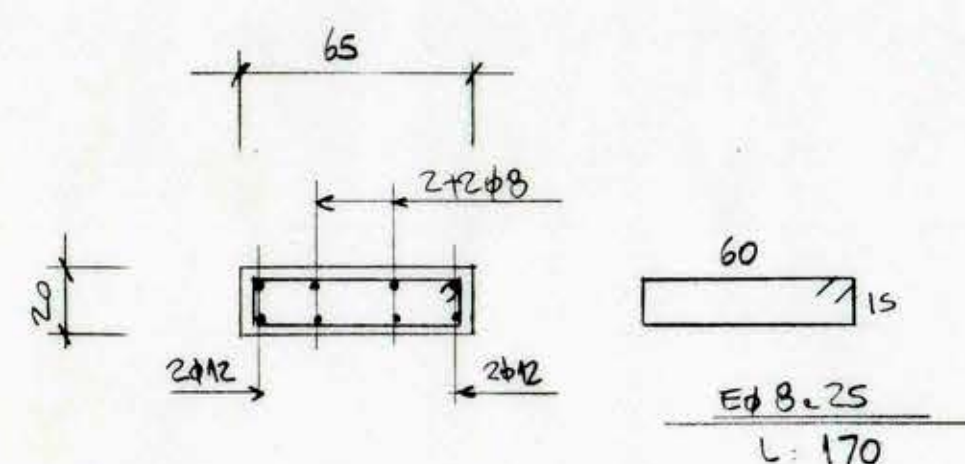
SECCION P1 20/65
