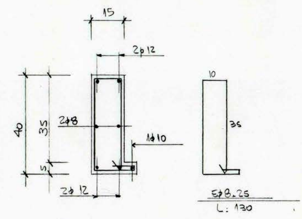
SECCION CAD 15/40/5+5
