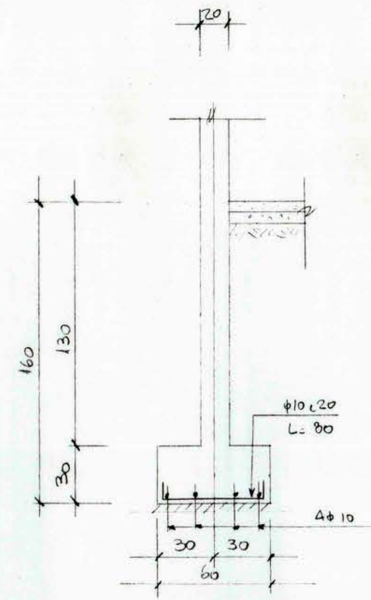
SECCION C-C
