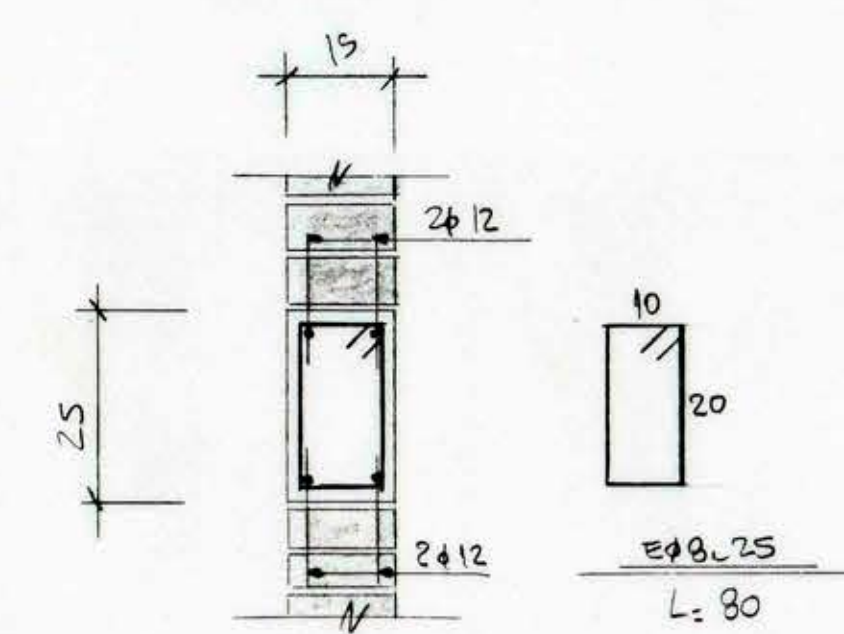
SECCION CAD 15/25
