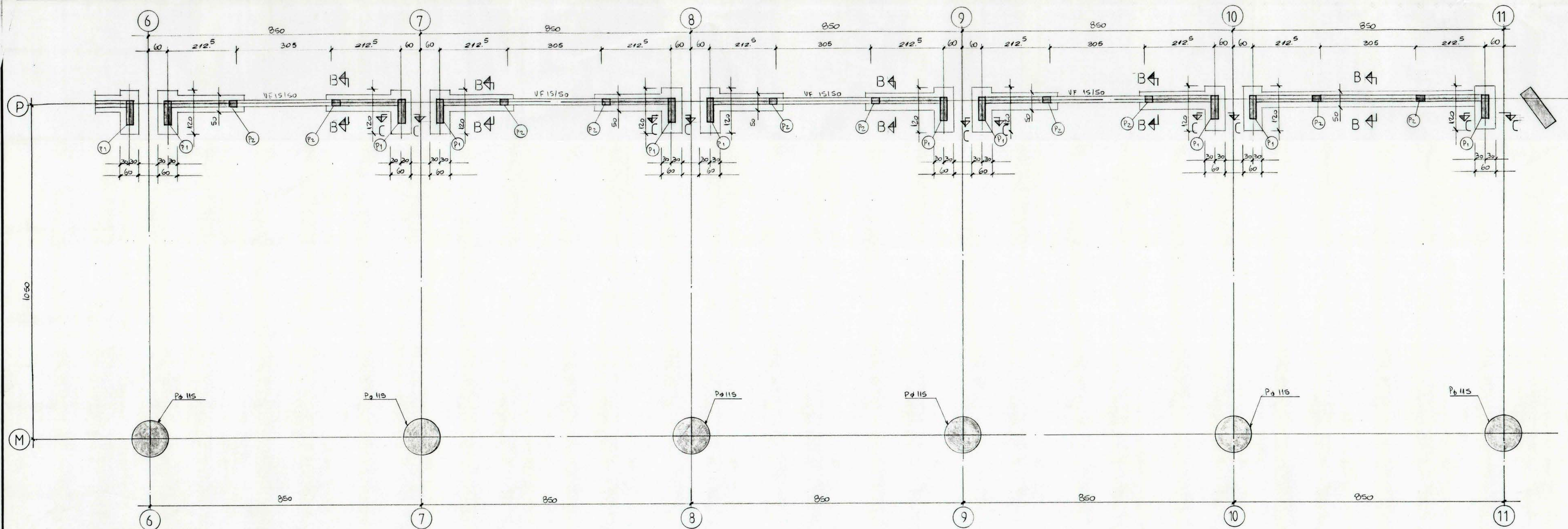
PLANTA DE FUNDACIONES
