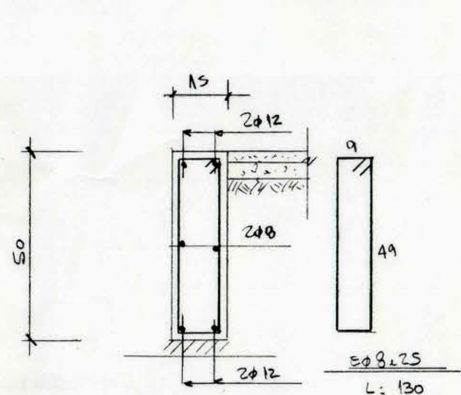
SECCION VF 15/50
