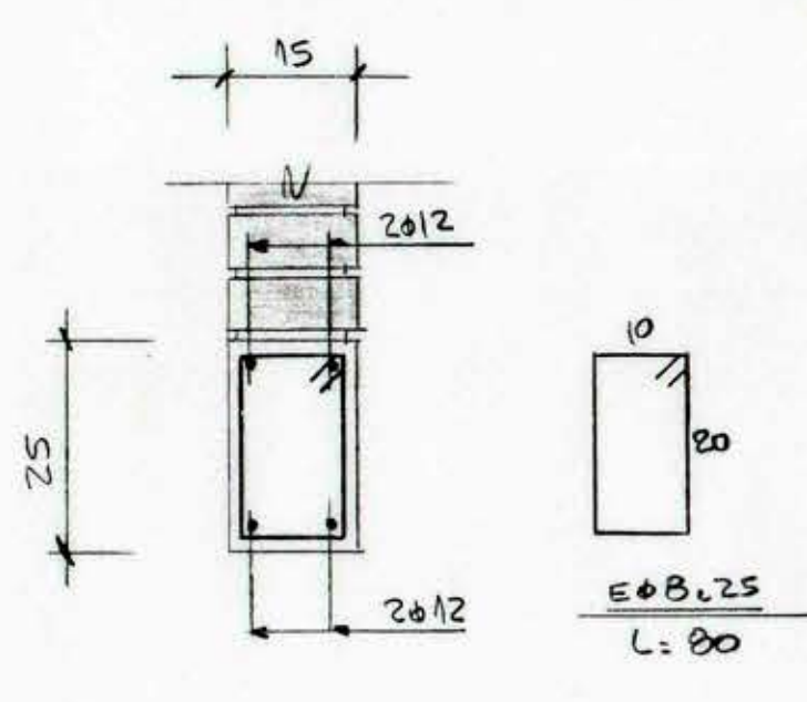
SECCION V 15/25
