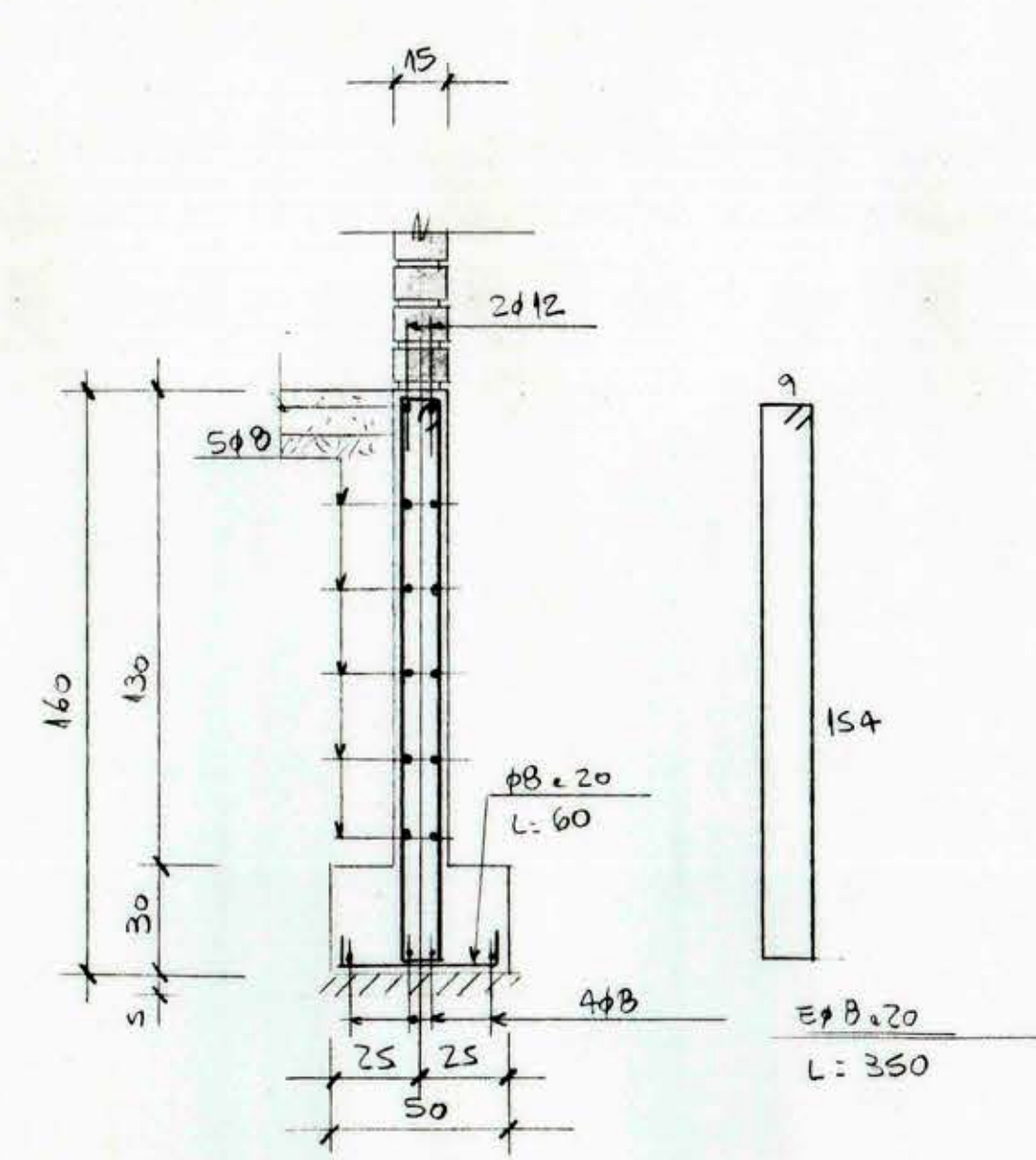
SECCION B-B
