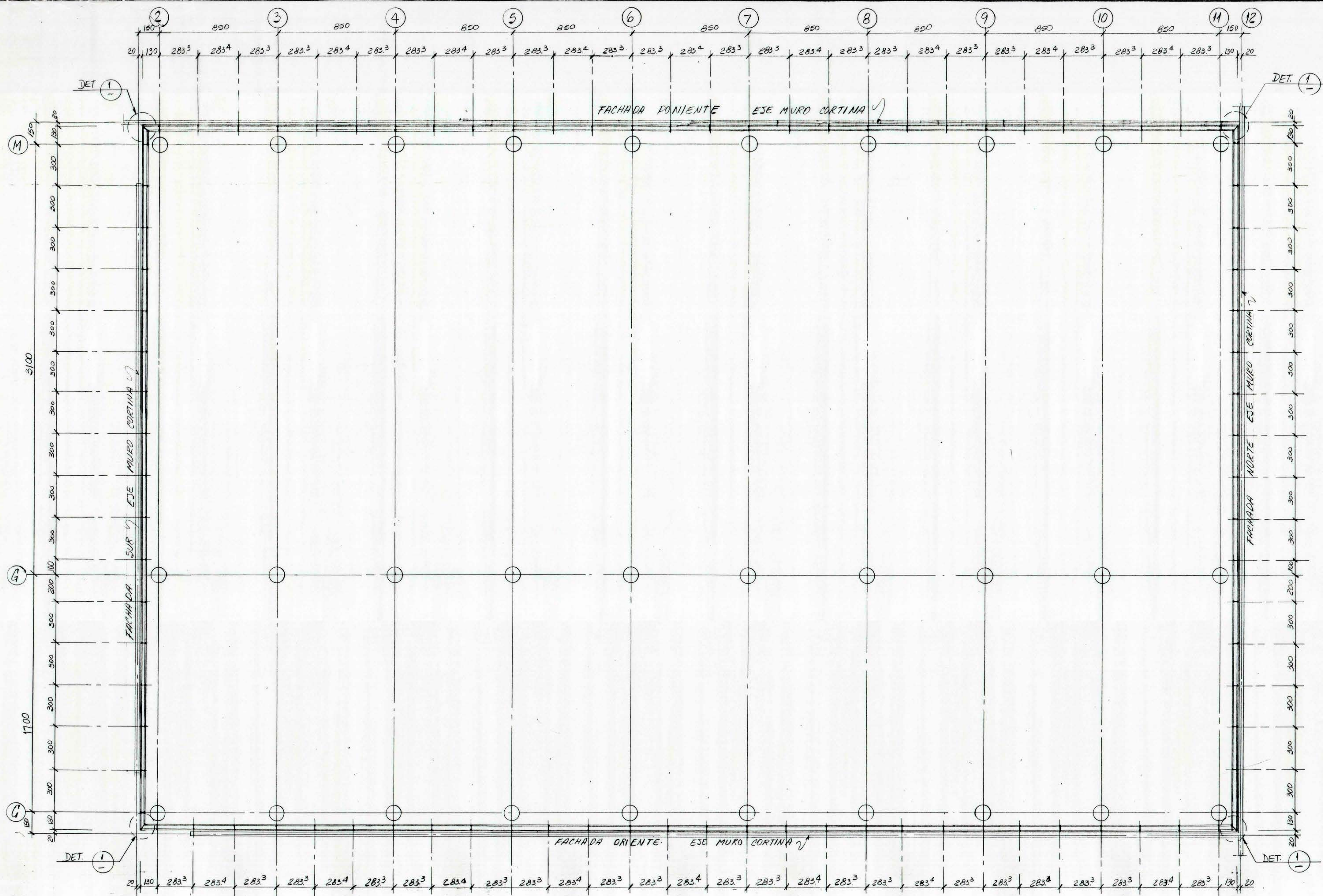
PLANTA GENERAL MUROS CORTINAS ESC 1/125
