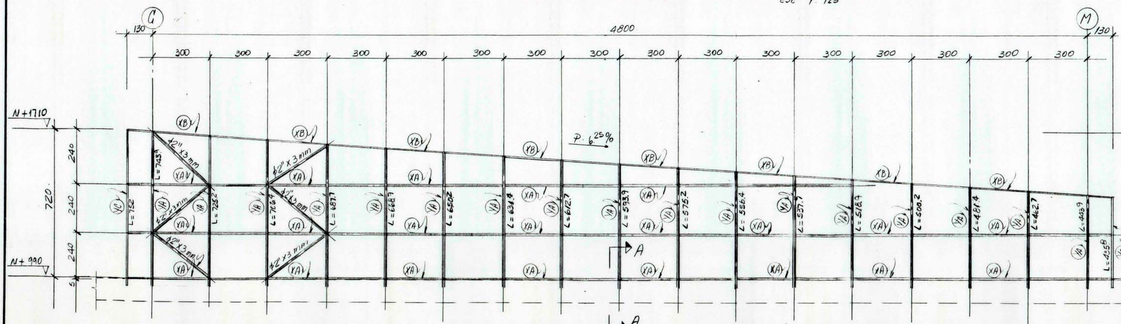
ESTRUCTURA MURO CORTINA FACHADA NORTE ESC 1/100
