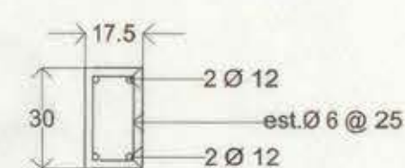
CADENA FUNDACION CF ESCALA 1:20
