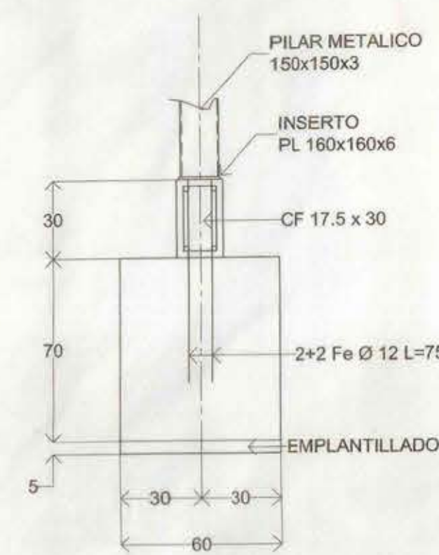
FUNDACION EJE PASILLO ESCALA 1:20
