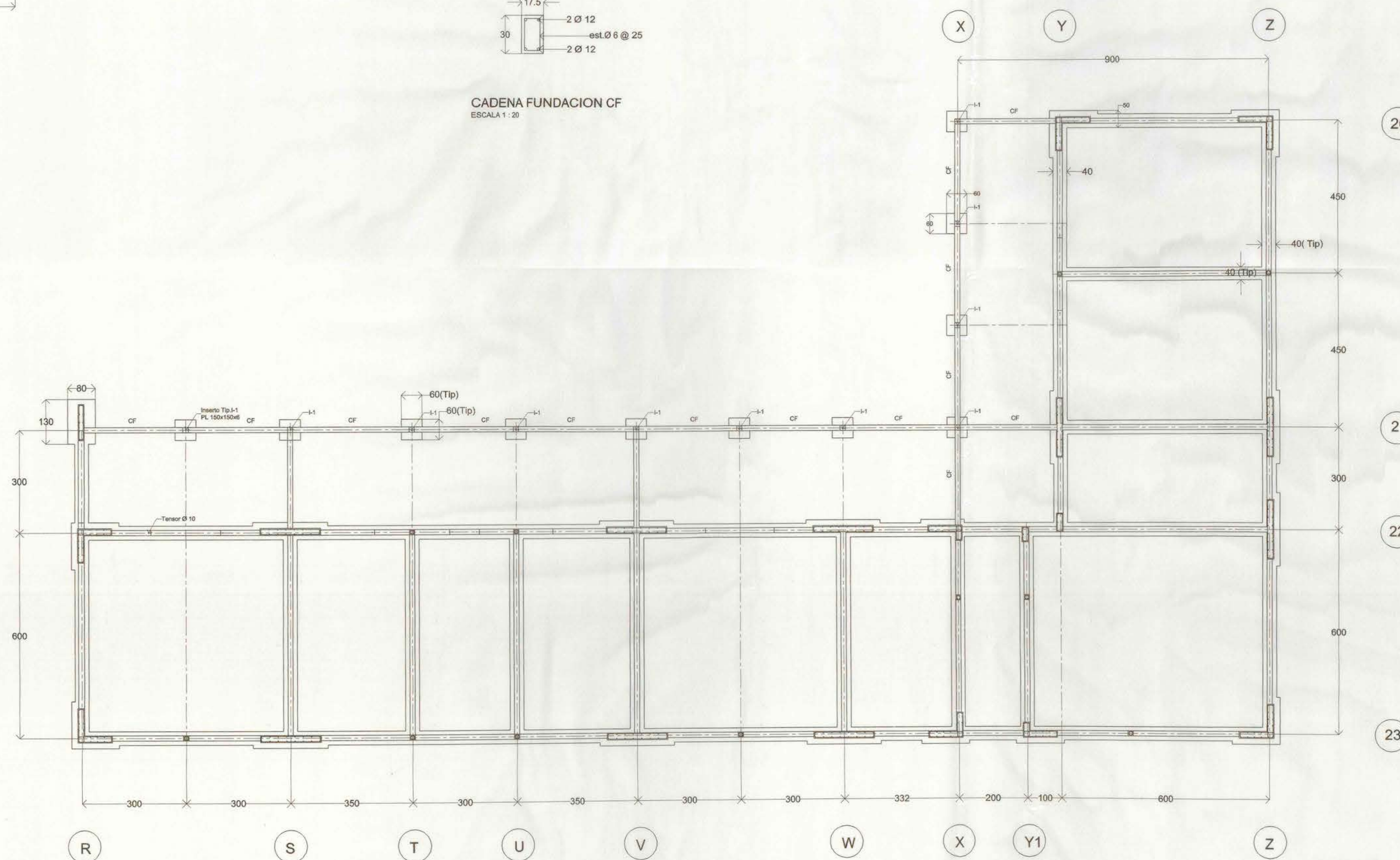
PLANTA FUNDACIONES PABELLON C ESCALA 1:75
