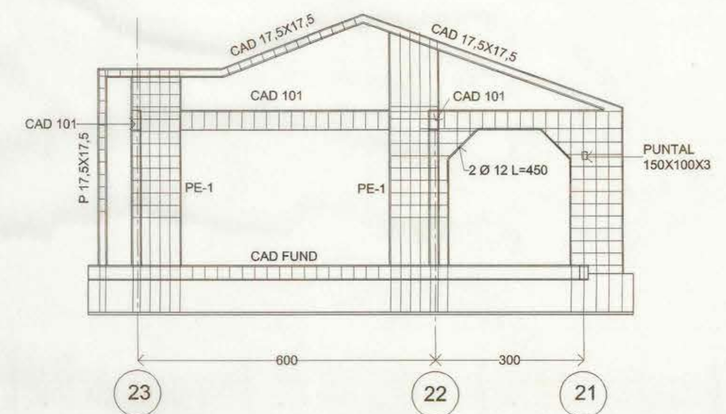
ELEVACION MURO EJE R ESCALA 1:75
