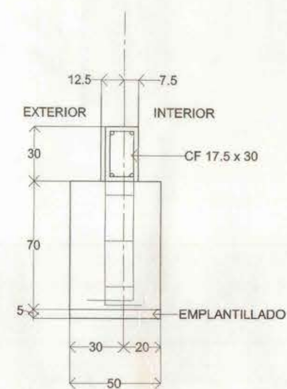
CORTE FUNDACION MACHONES ESCALA 1:20
