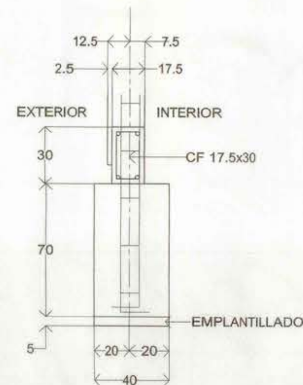
CORTE FUNDACION P1 ESCALA 1:20
