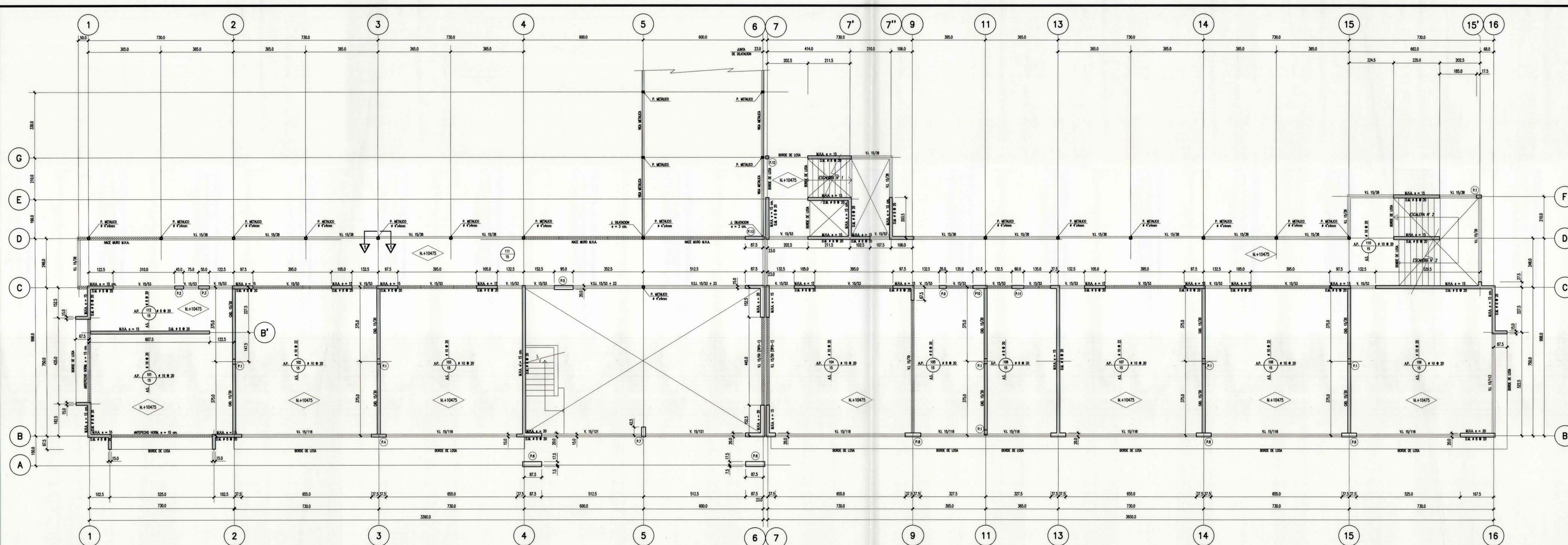
PLANTA DE ESTRUCTURA LOSA CIELO 1° PISO
