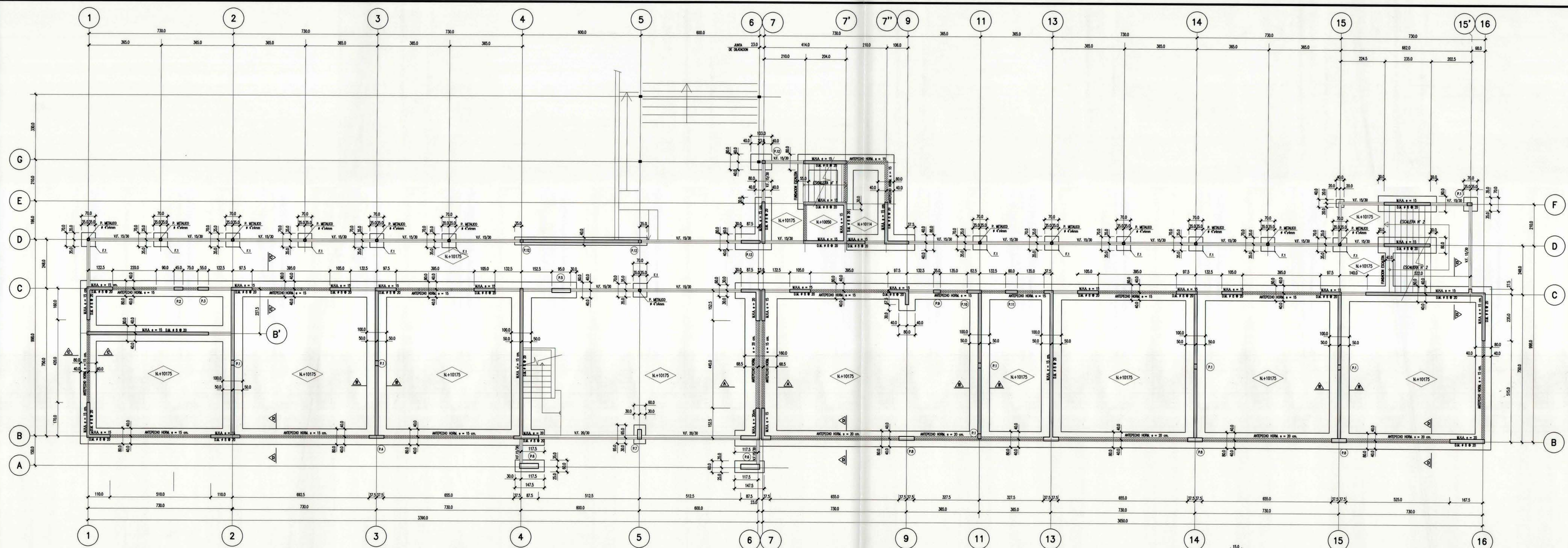
PLANTA DE FUNDACIONES
