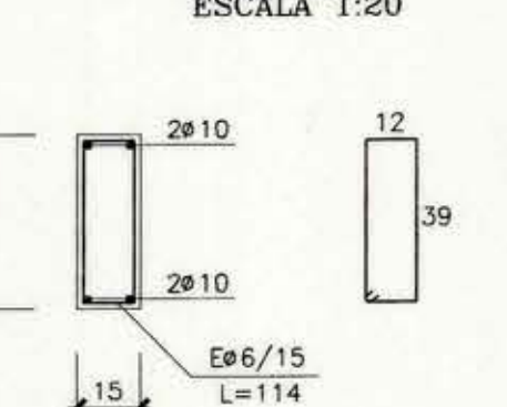
CORTE 3-3 ESCALA 1:20
