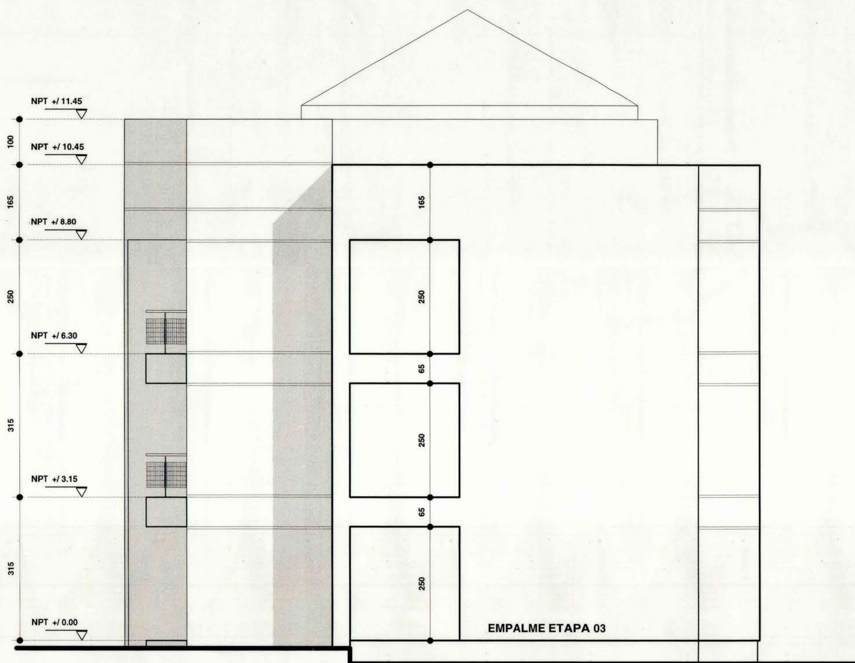
ETAPA N° 01 ELEVACION ORIENTE
