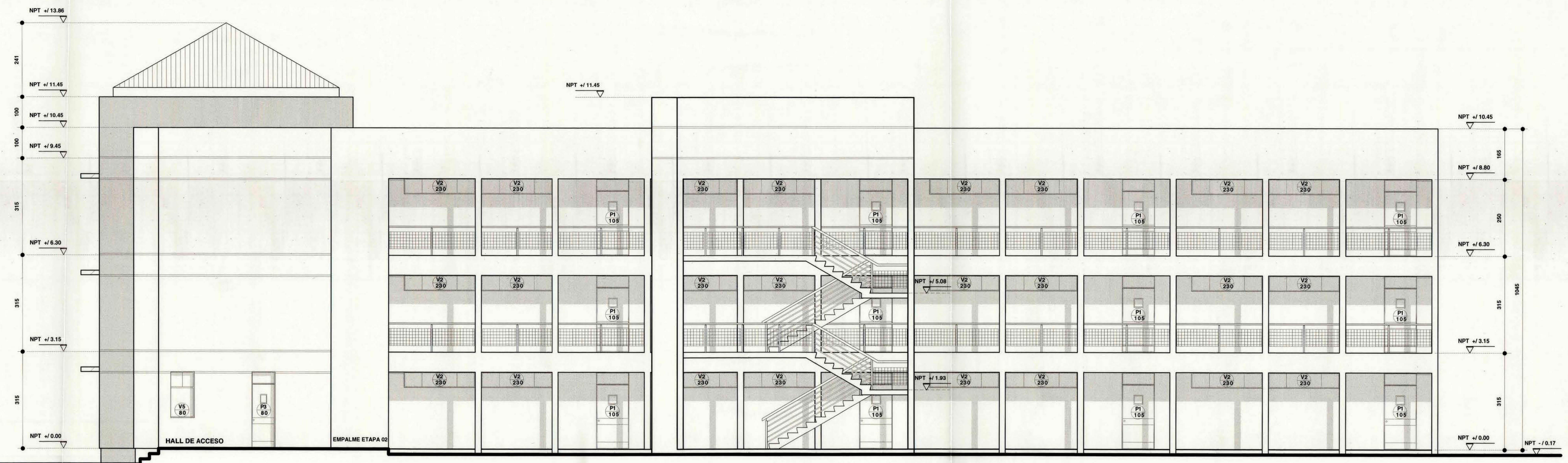
ELEVACION INTERIOR PATIO
