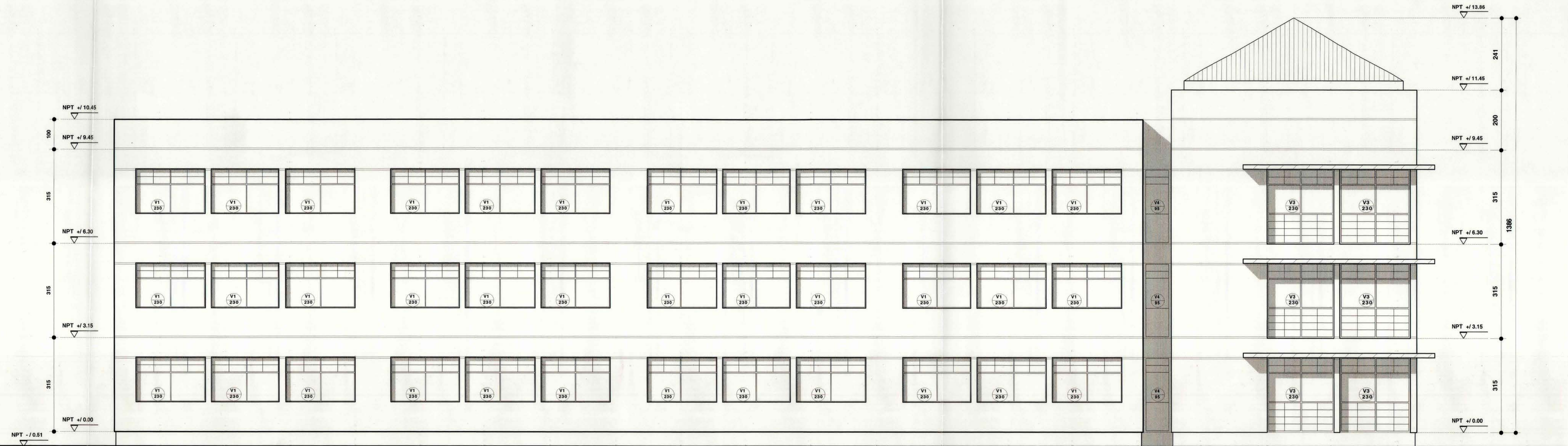
ELEVACION NORTE
