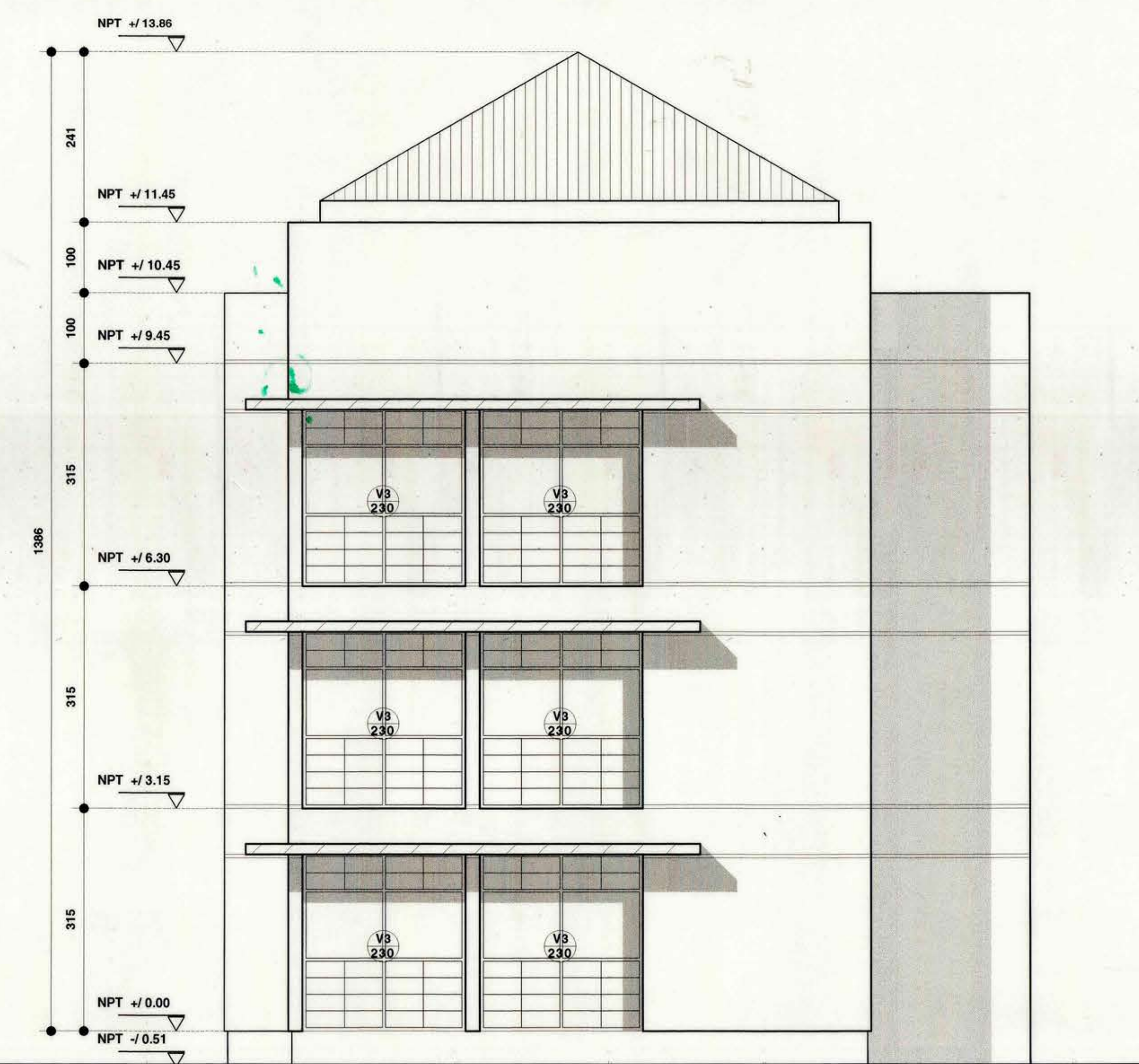
ETAPA N° 01 ELEVACION FACHADA ACCESO
