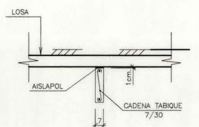
DILATACION DE TABIQUE BAJO LOSA ESCALA 1:20
