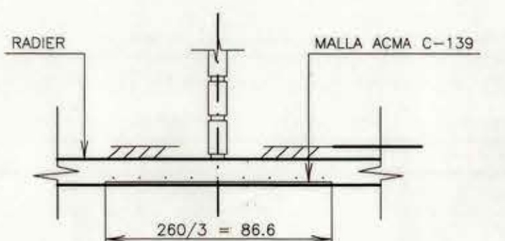
REFUERZO RADIER BAJO TABIQUERIA ESCALA 1:20
