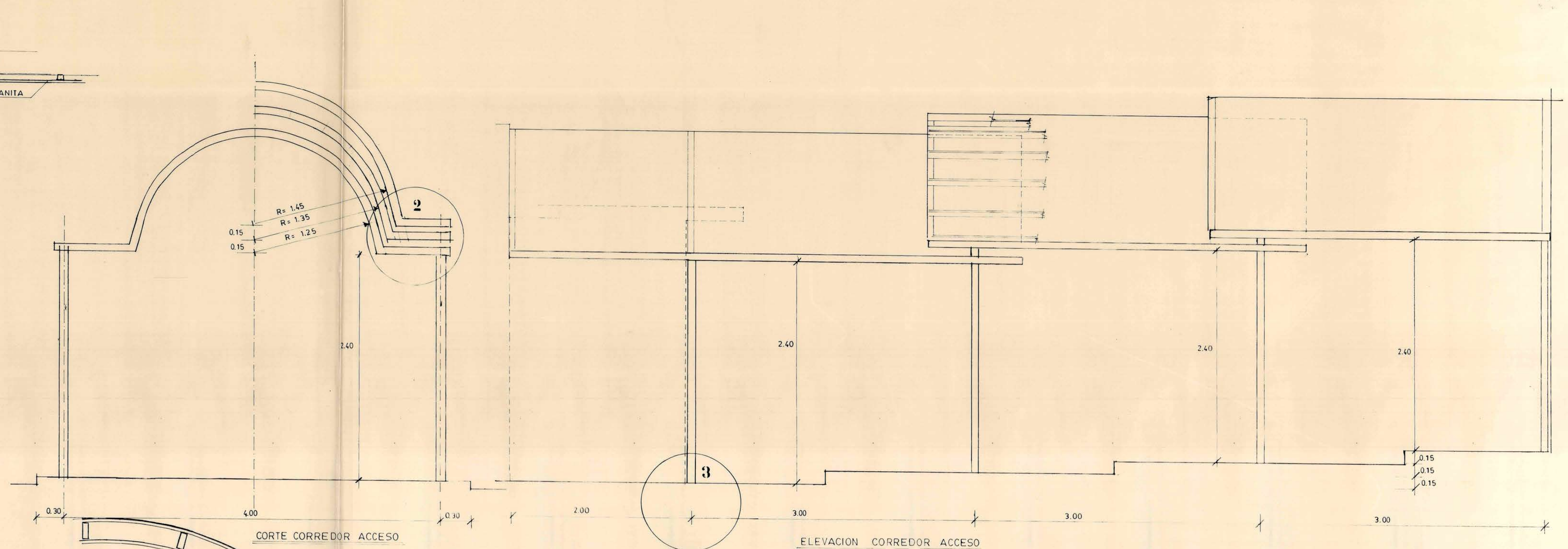
ELEVACION CORREDOR ACCESO
