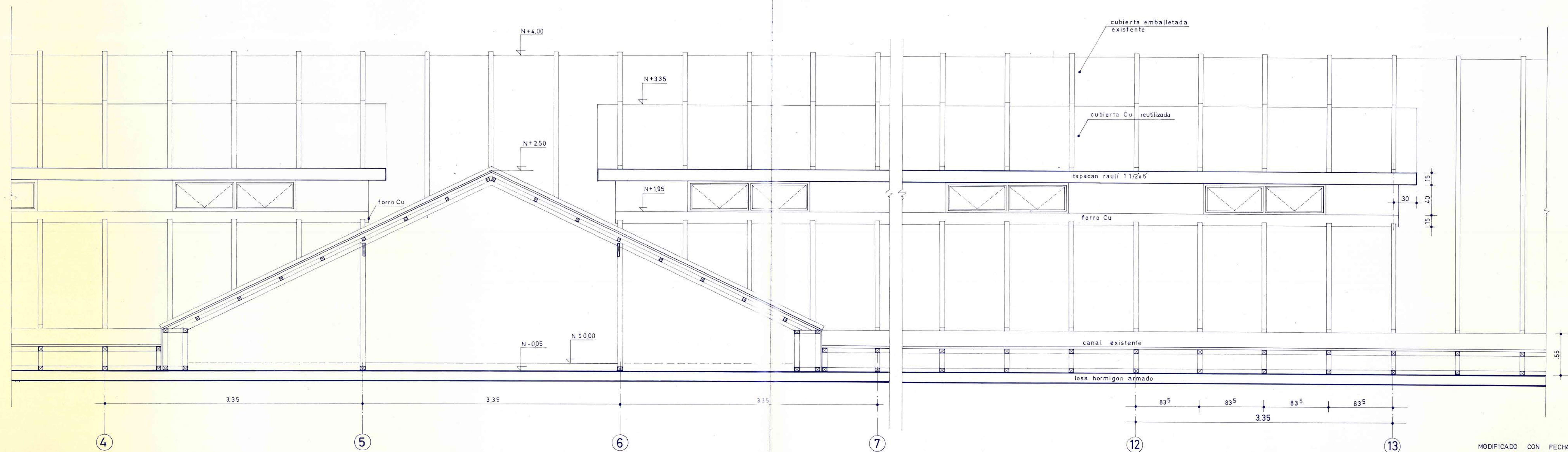
CORTE-ELEVACION SUR ESCALA 1:20
