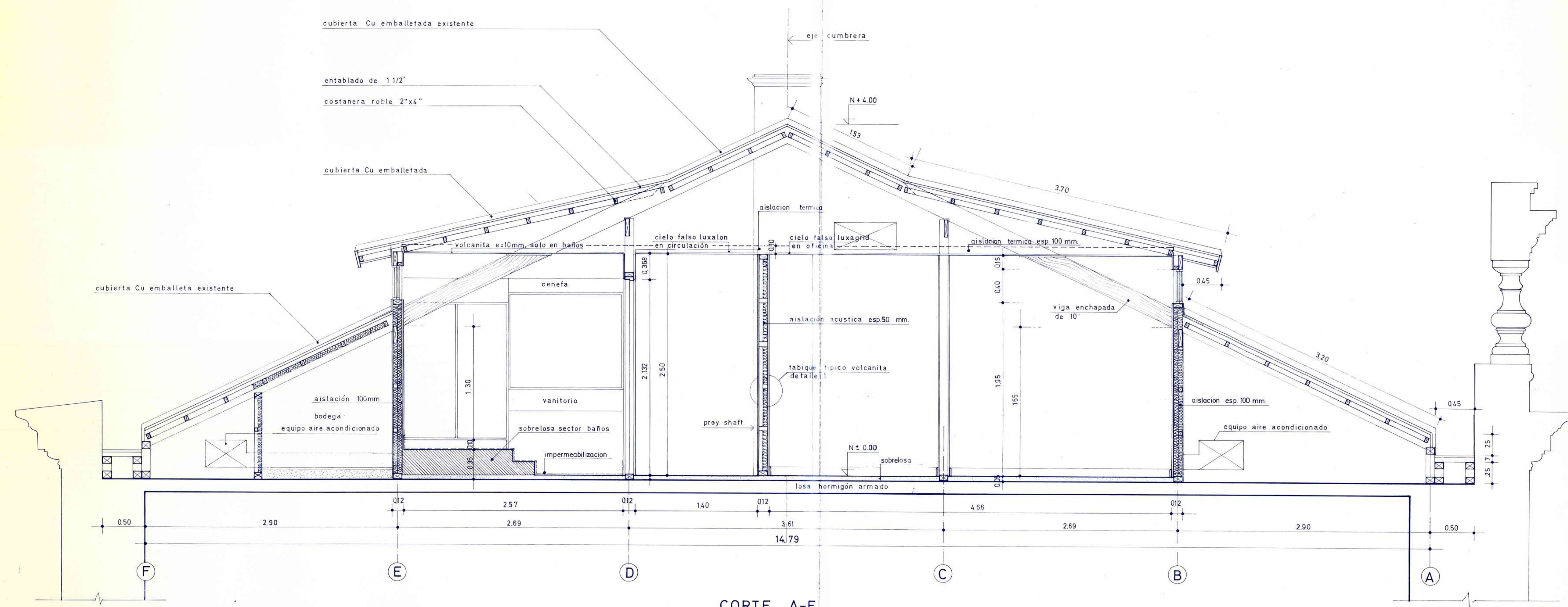
CORTE A-F ESCALA 1:20
