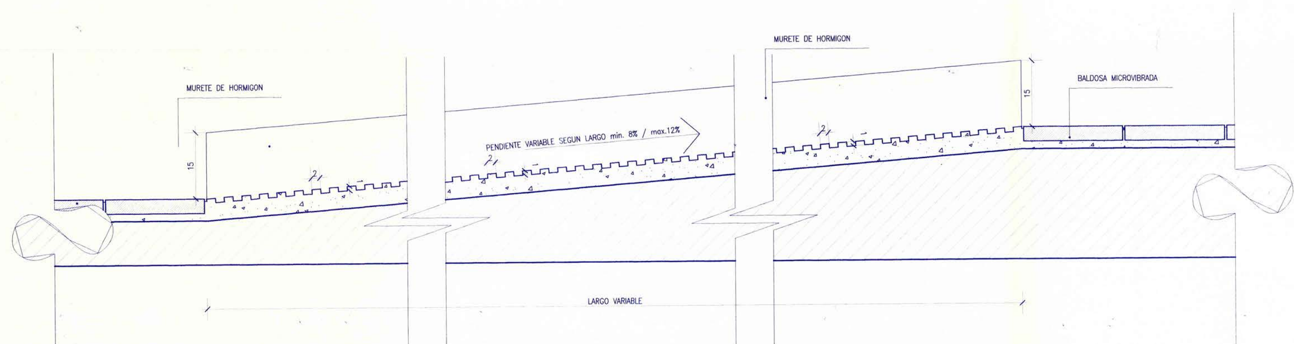
DETALLE RAMPA (Largo y pendiente variable segun caso) ESC. 1/5
