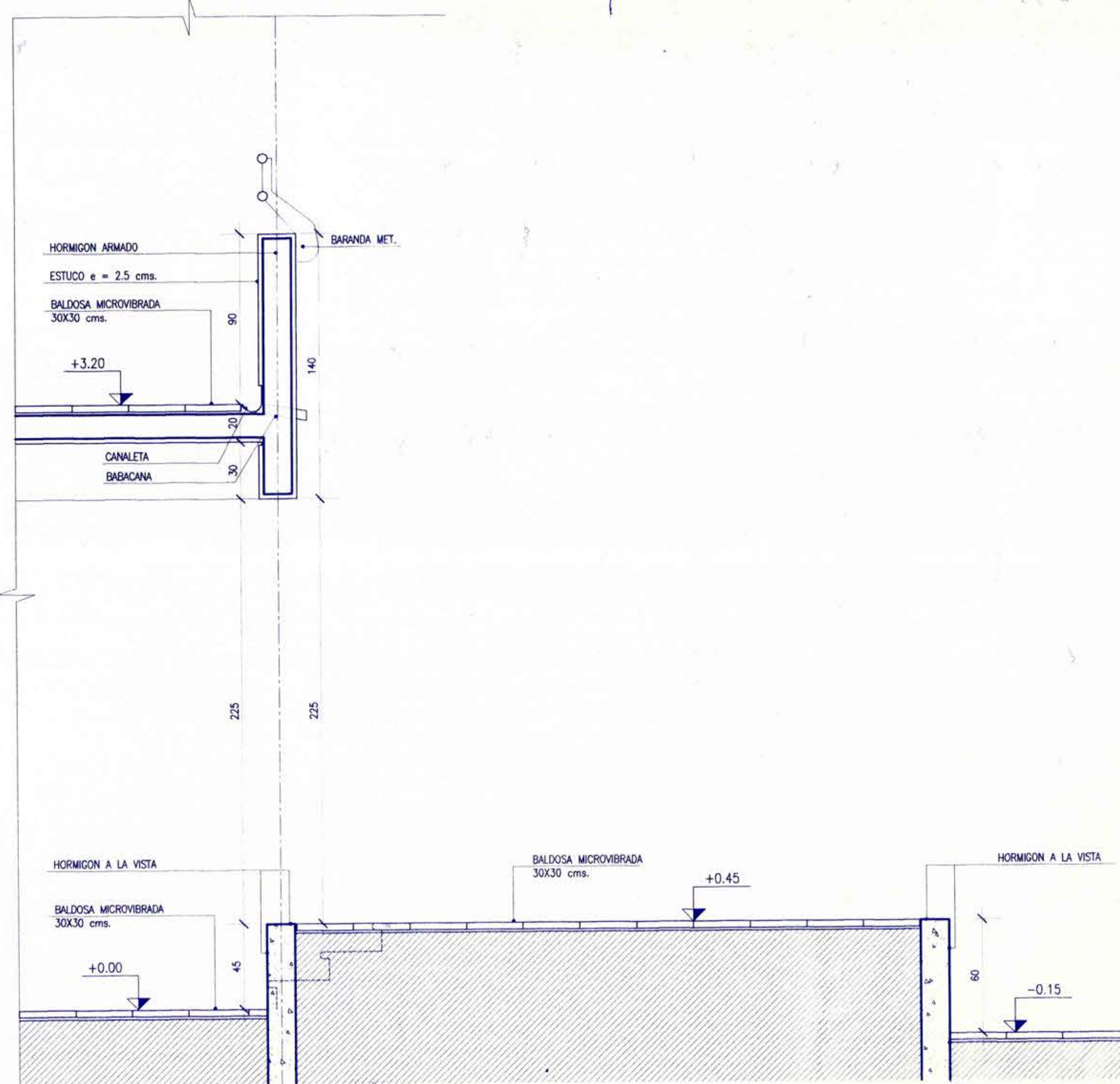
DETALLE ZONA DE ACTOS ESC. 1/20
