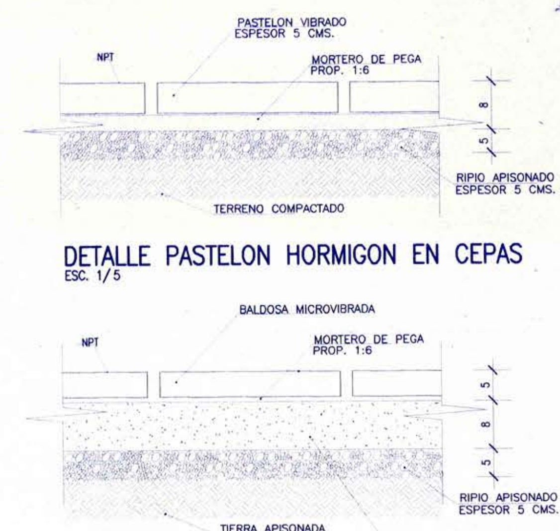
DETALLE BALDOSA MICROVIBRADA MODELO COLONIAL ESC. 1/5
