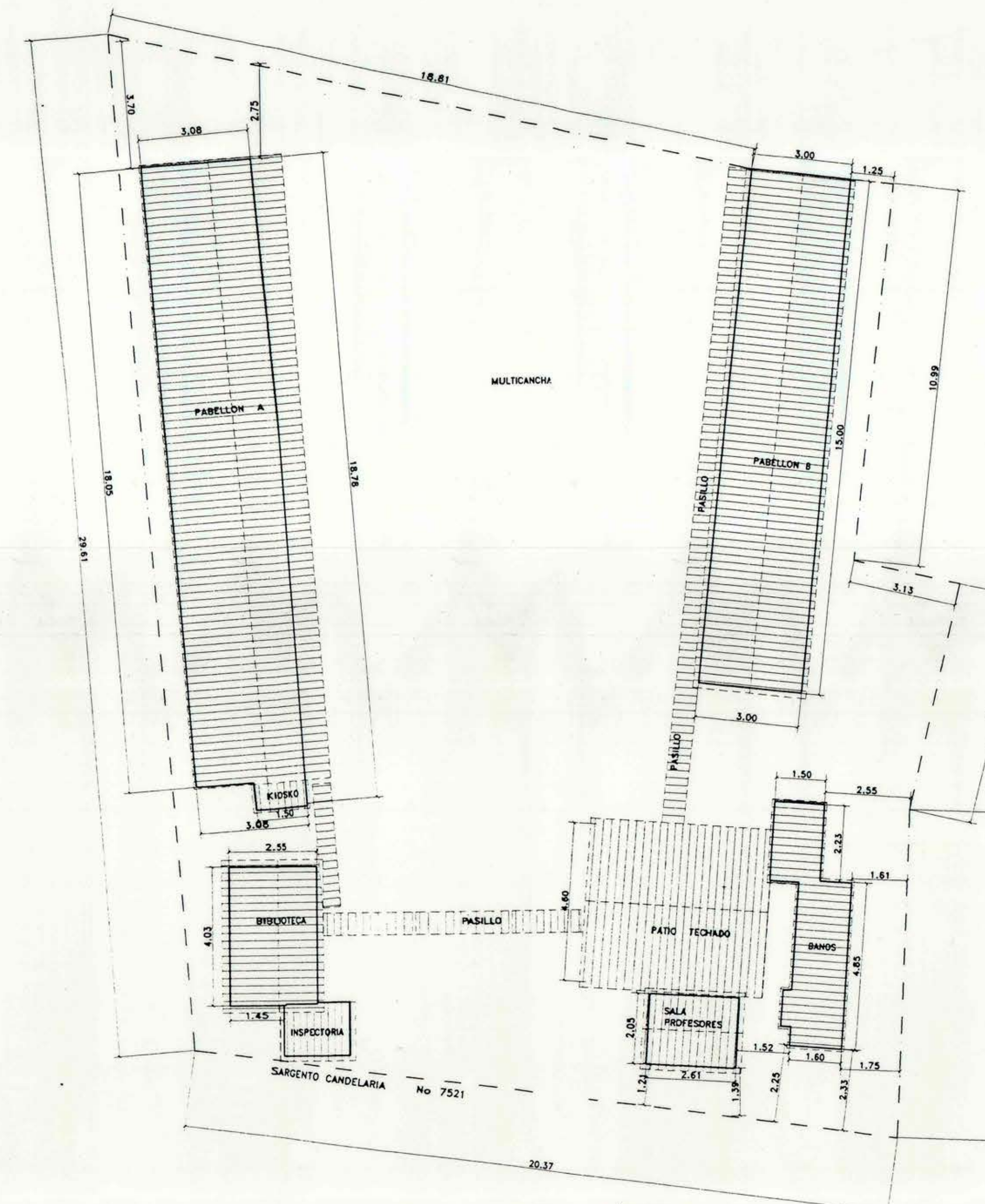
EMPLAZAMIENTO ESC. 1/200
