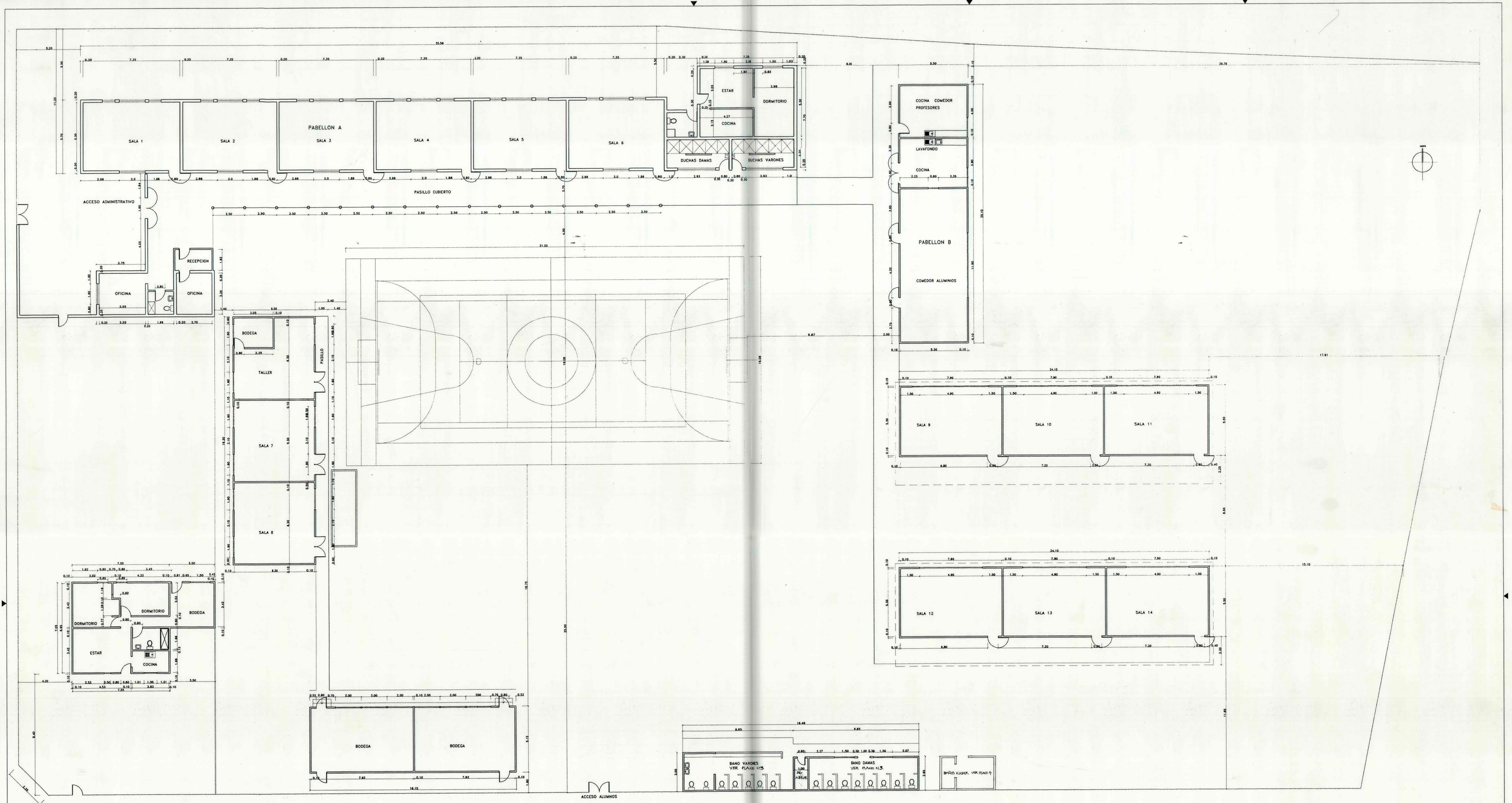
PLANTA GENERAL ARQUITECTURA
