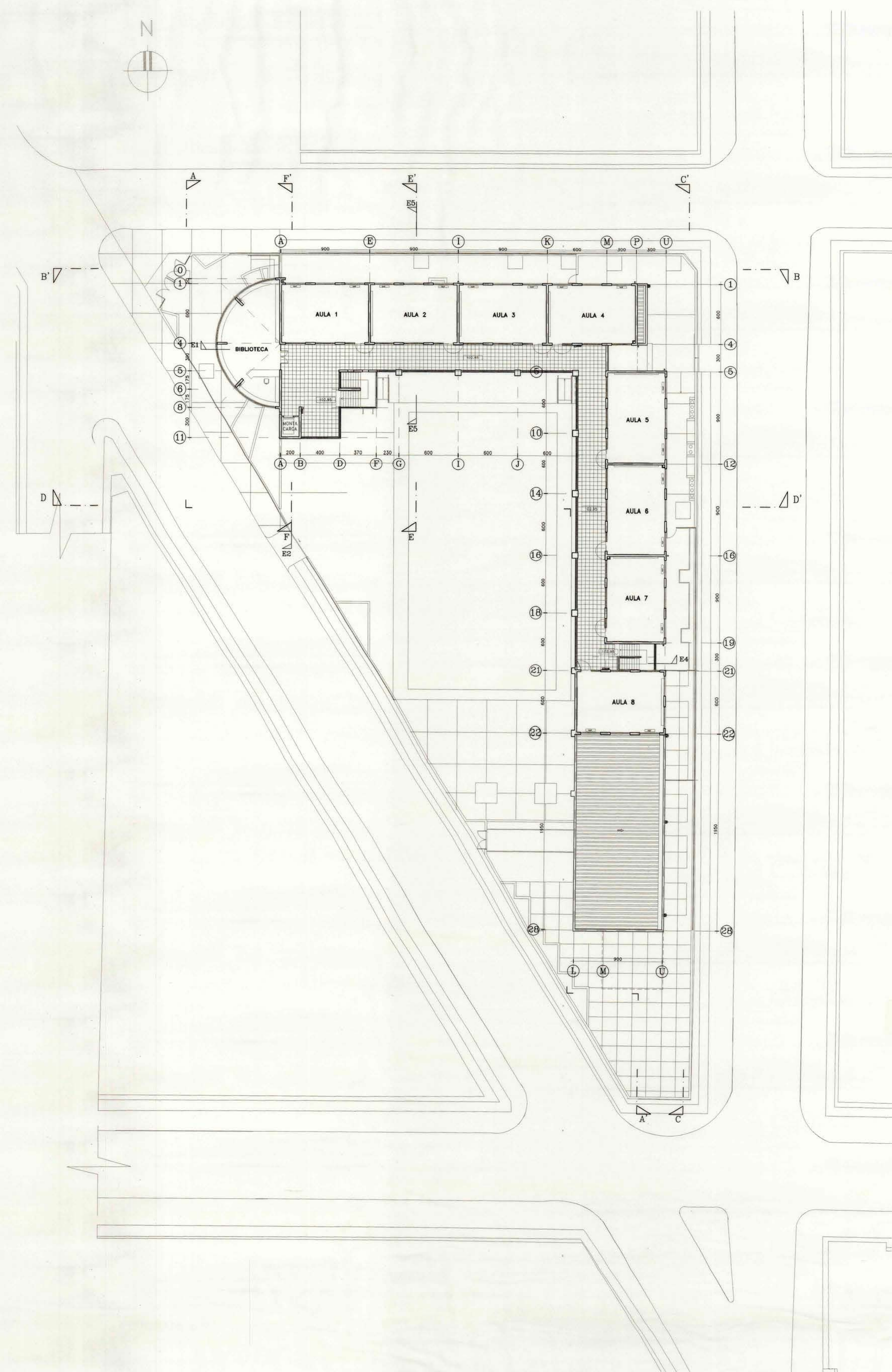
PLANTA GENERAL ARQUITECTURA 2° NIVEL
