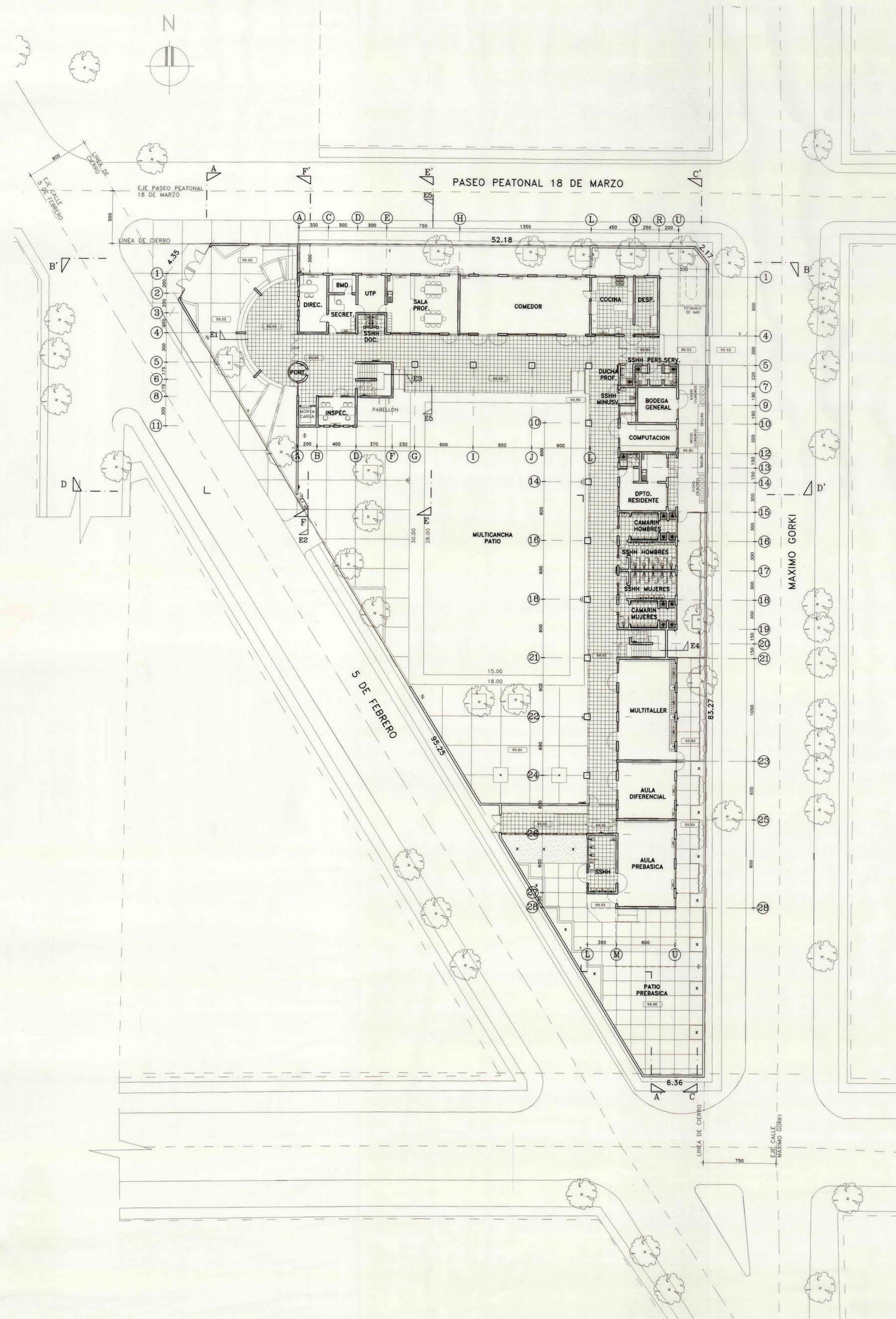
PLANTA GENERAL ARQUITECTURA 1° NIVEL
