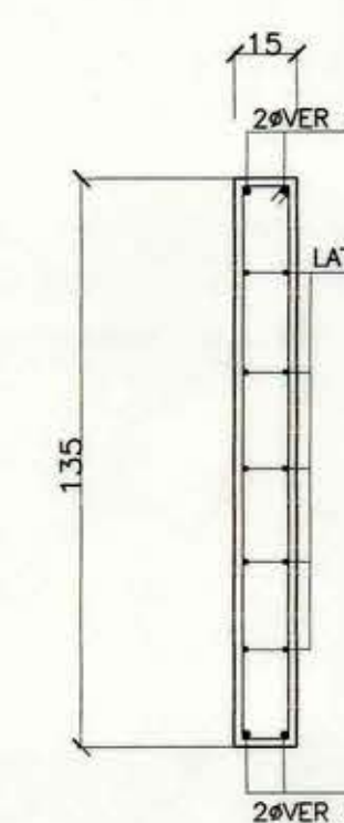
PILAR P11. ESCALA 1:20.
