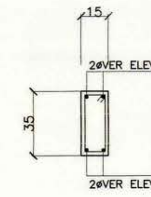
PILAR P10. ESCALA 1:20.
