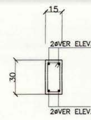
PILAR P13. ESCALA 1:20.
