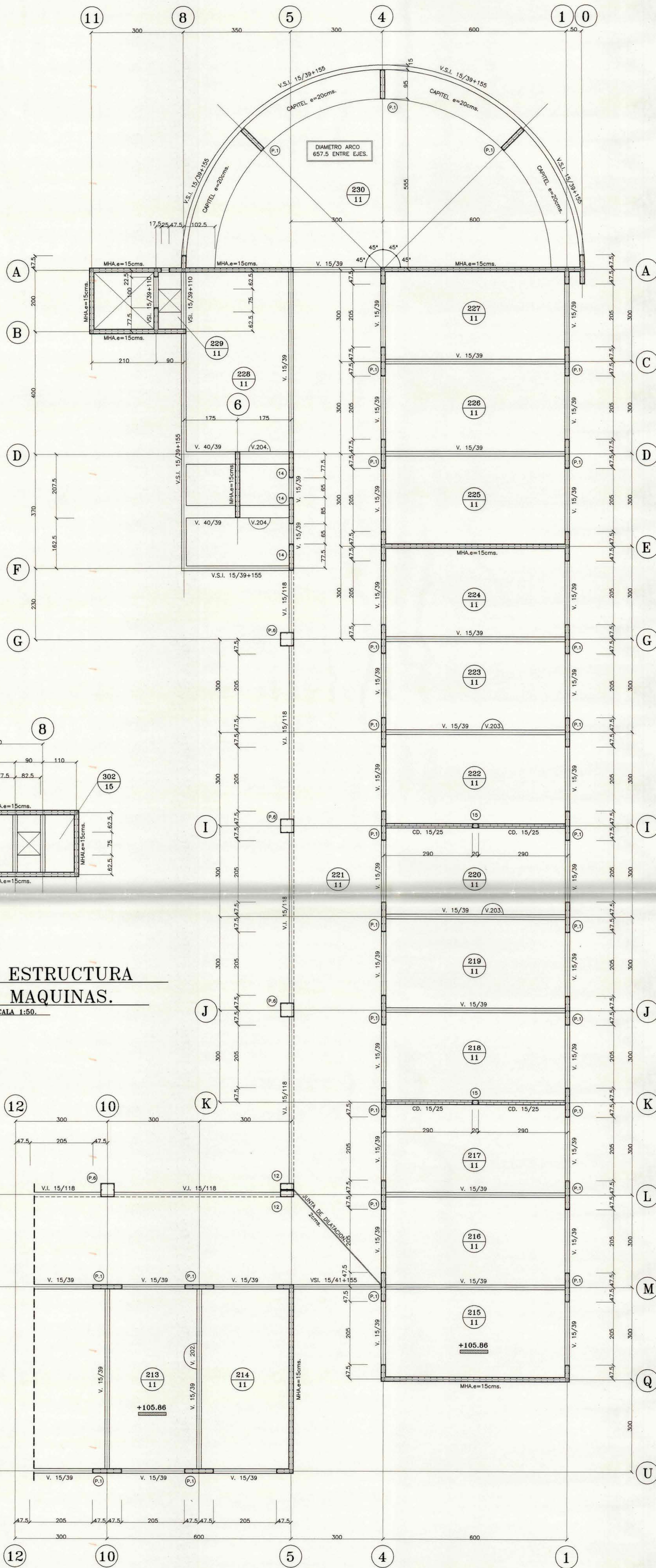
PLANTA DE ESTRUCTURA CIELO 2° PISO SECTOR B. ESCALA 1:50.
