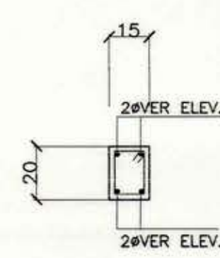
PILAR P15. ESCALA 1:20.
