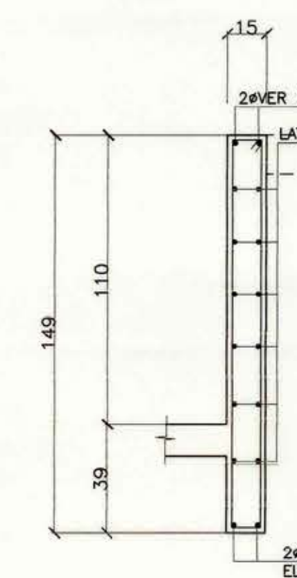
VSI.15/39+110. ESCALA 1:20.
