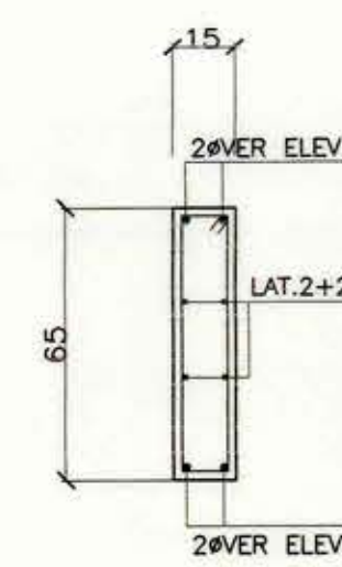
PILAR P8. ESCALA 1:20.
