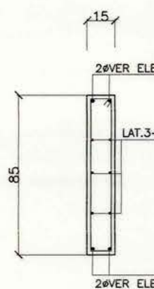
PILAR P14. ESCALA 1:20.
