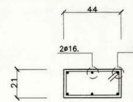
PILAR P12. ESCALA 1:20.
