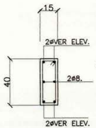
PILAR P9. ESCALA 1:20.
