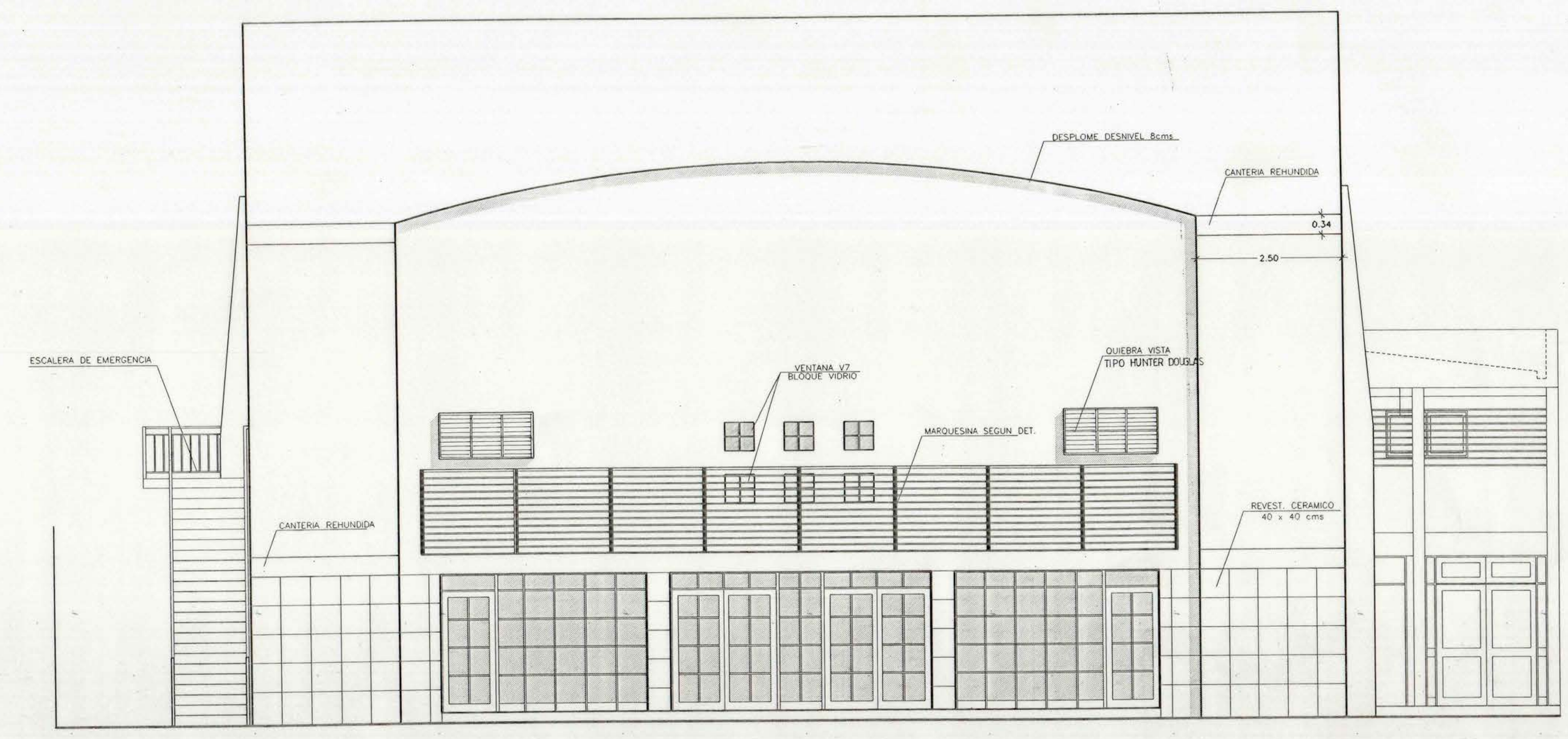
ELEVACION PRINCIPAL DETALLES ESCALA 1:50
