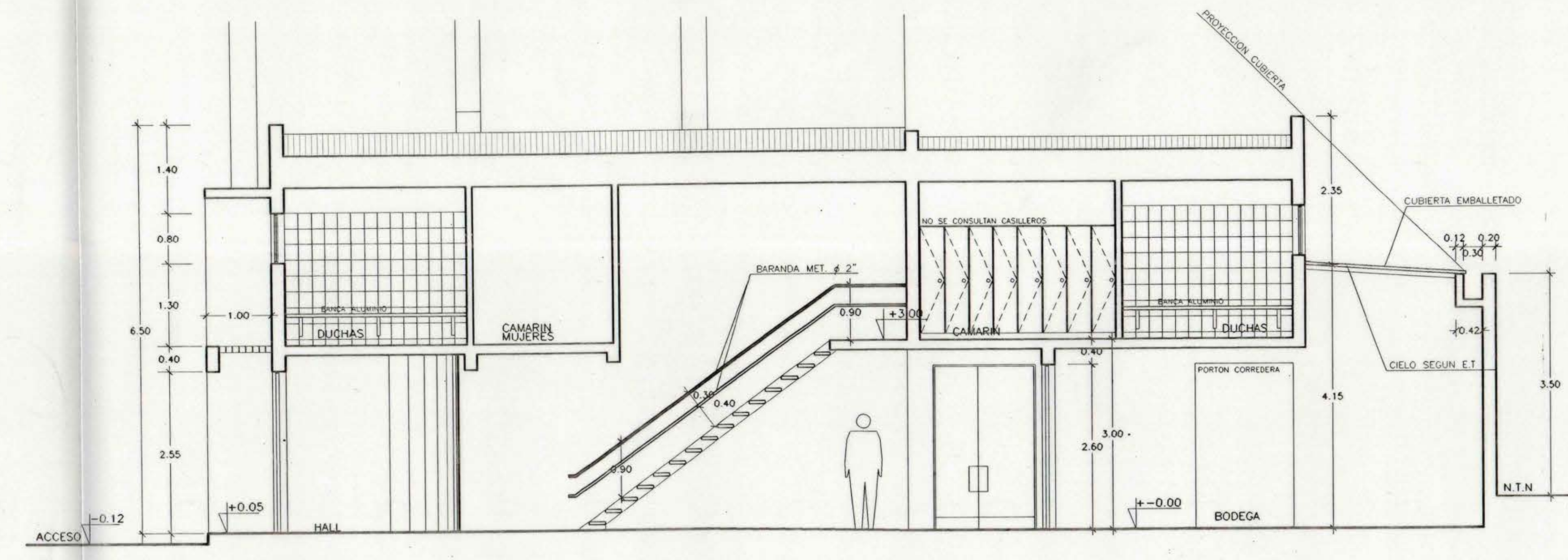
CORTE D-D ESCALERA ESCALA 1:50
