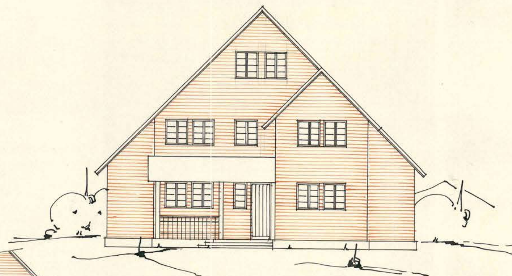
FACŢADA C.
