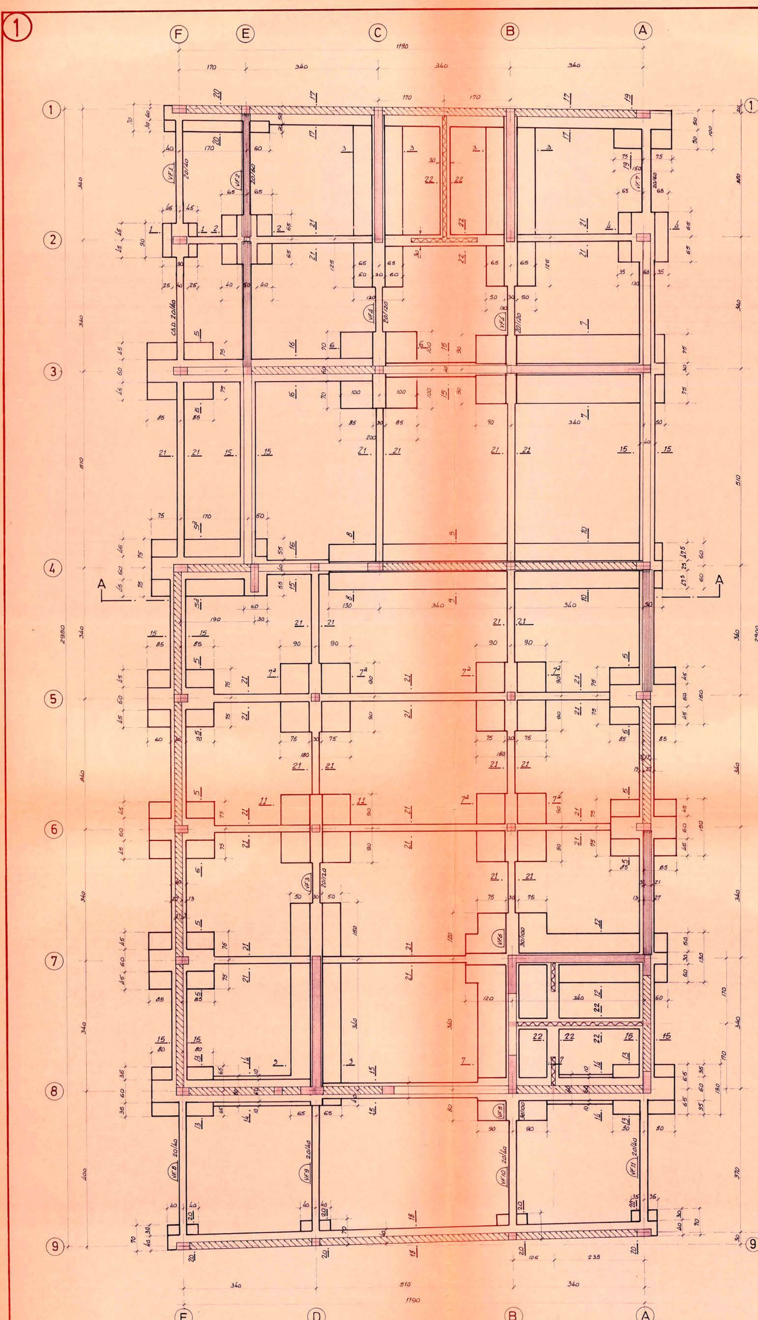
PLANTA FUNDACIONES
