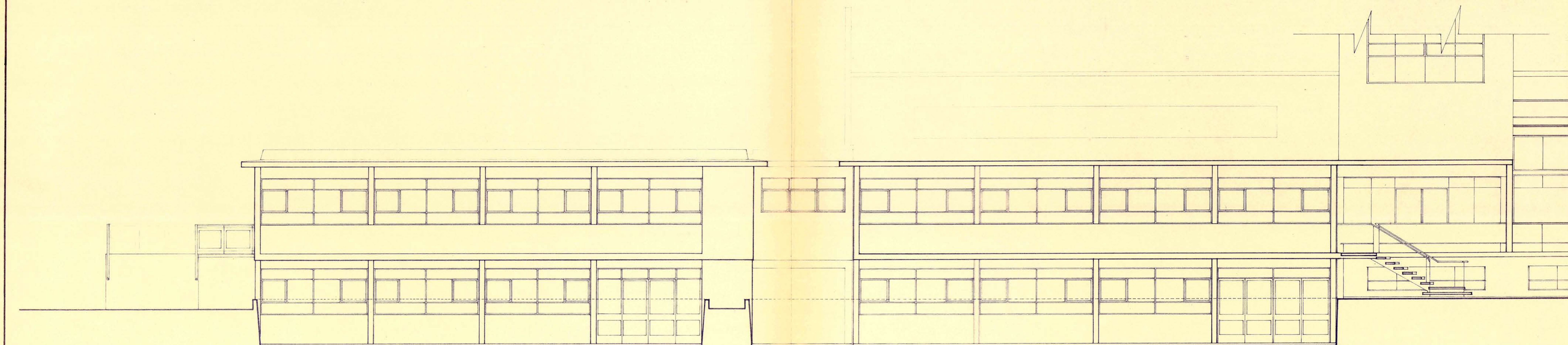
ELEVACION PONIENTE. (principal)
