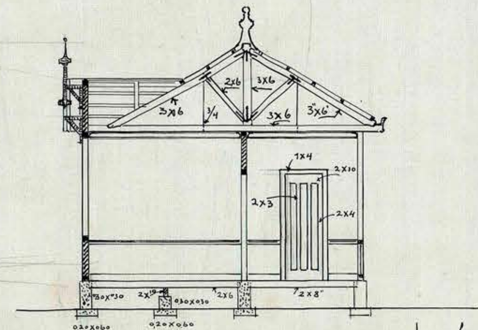
CORTE EN LA OFICINA Y PORTICO
