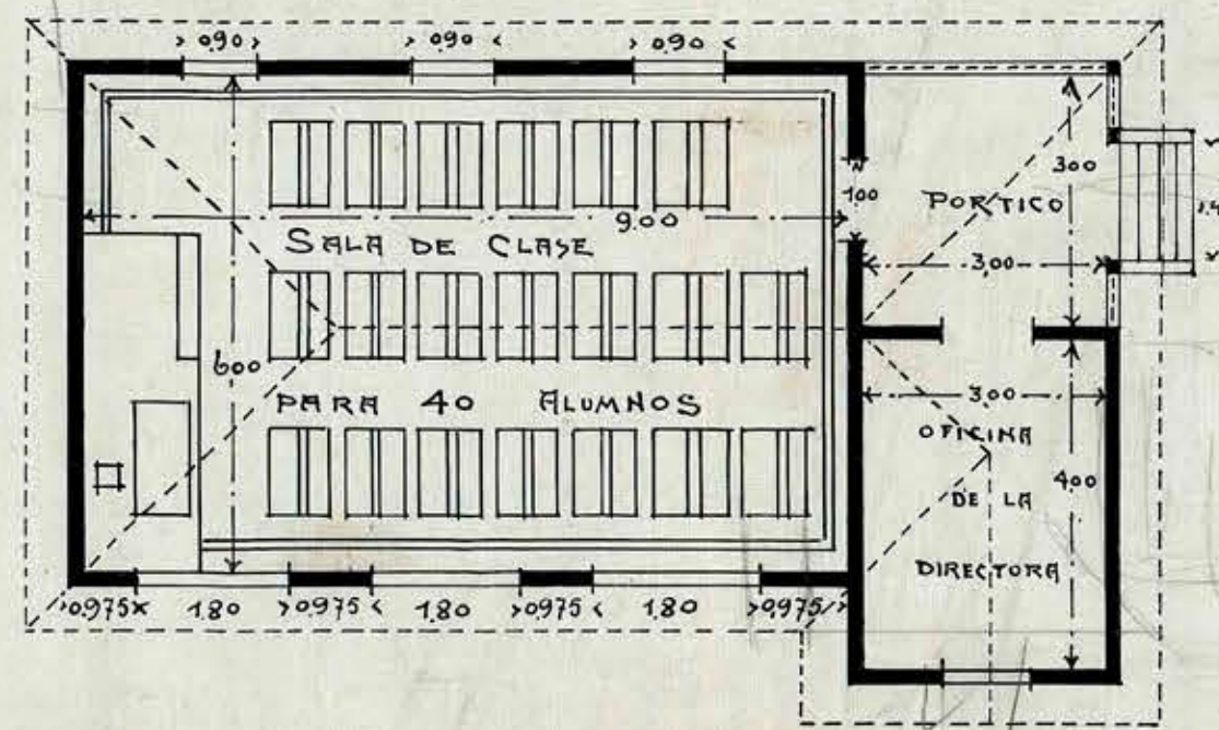
PLANO HORIZONTAL DE LA ESCUELA
