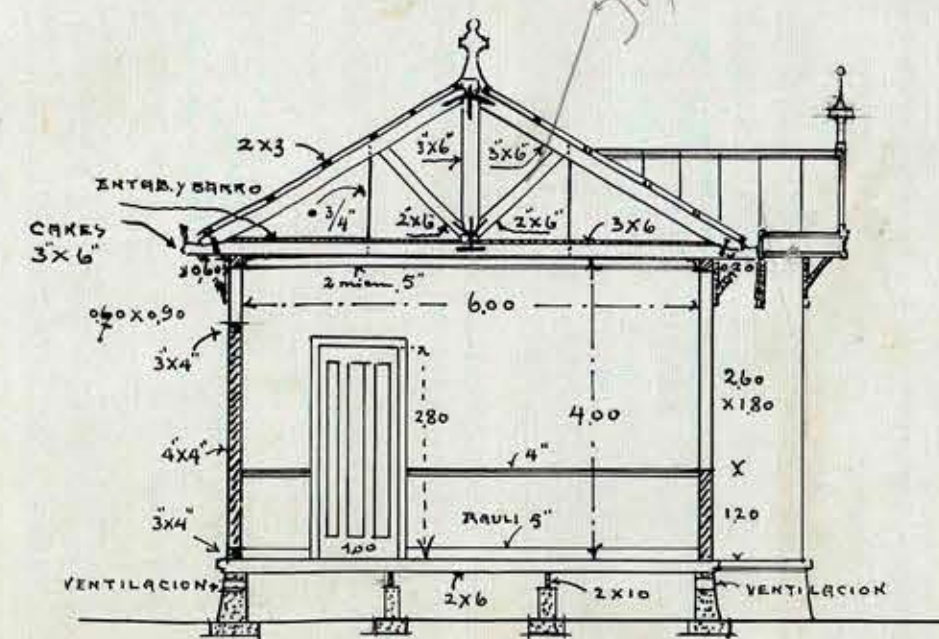
CORTE EN SALA DE CLASE
