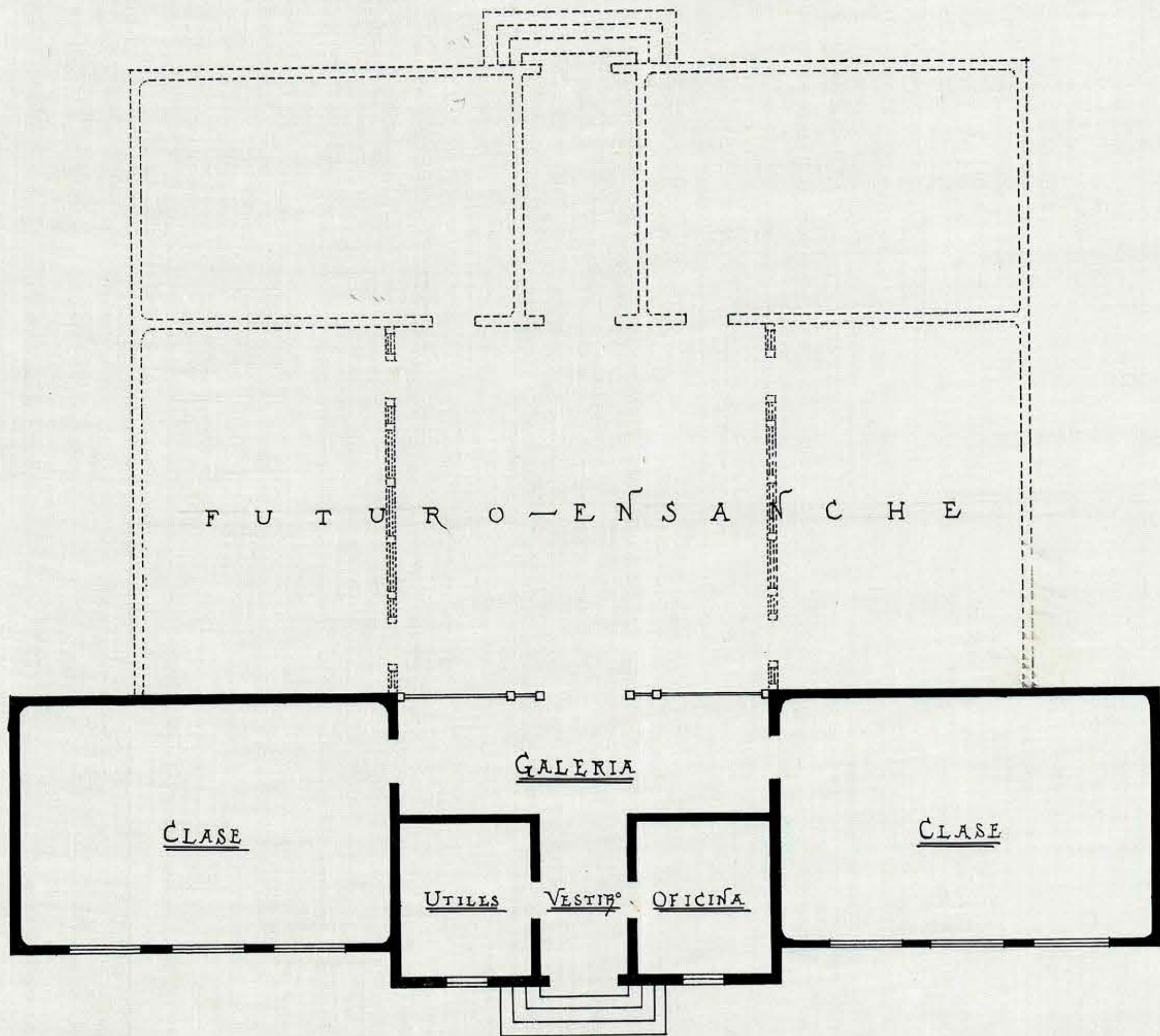
PLANO HORIZONTAL
