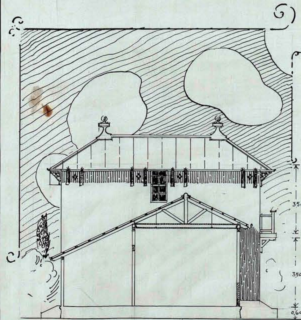
CORTE EN SALA DE CLASE Eje 001 7/8
