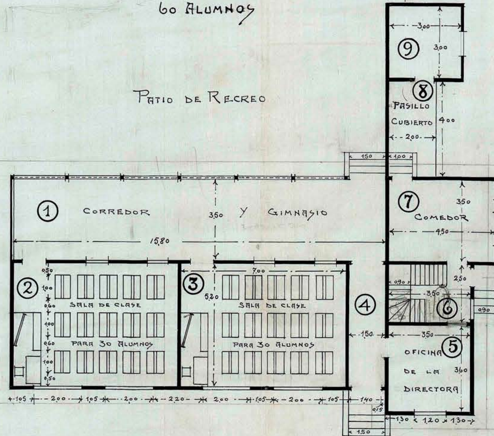
PLANO HORIZONTAL DE LA ESCUELA
