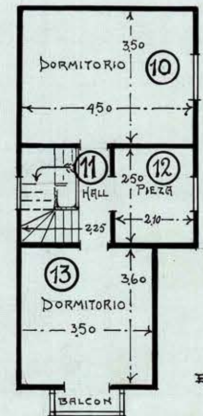
SEGUNDO PISO DE LA CASA DE LA PRECEPTORA
