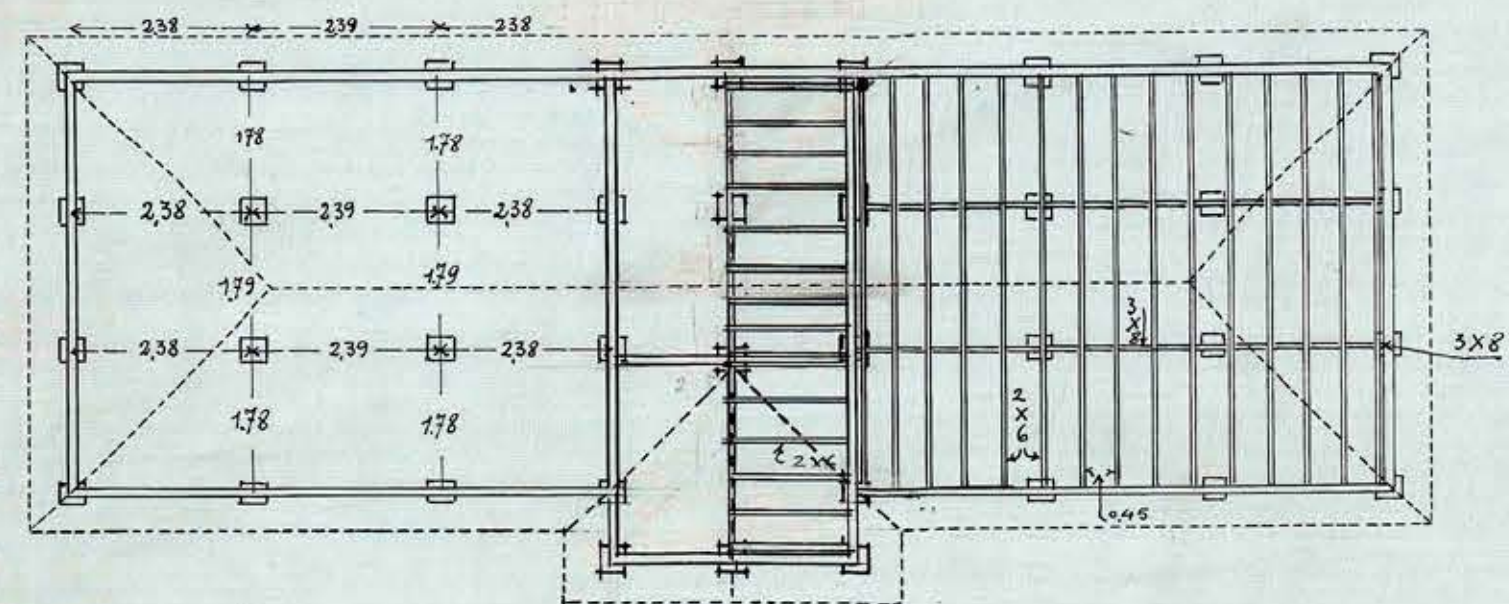
PLANO DE LOS ENVIGADOS
