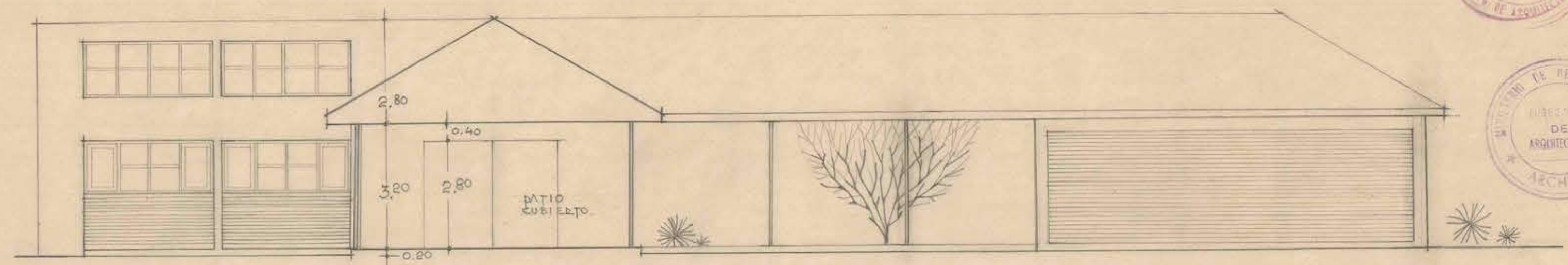
CORTE A-N
