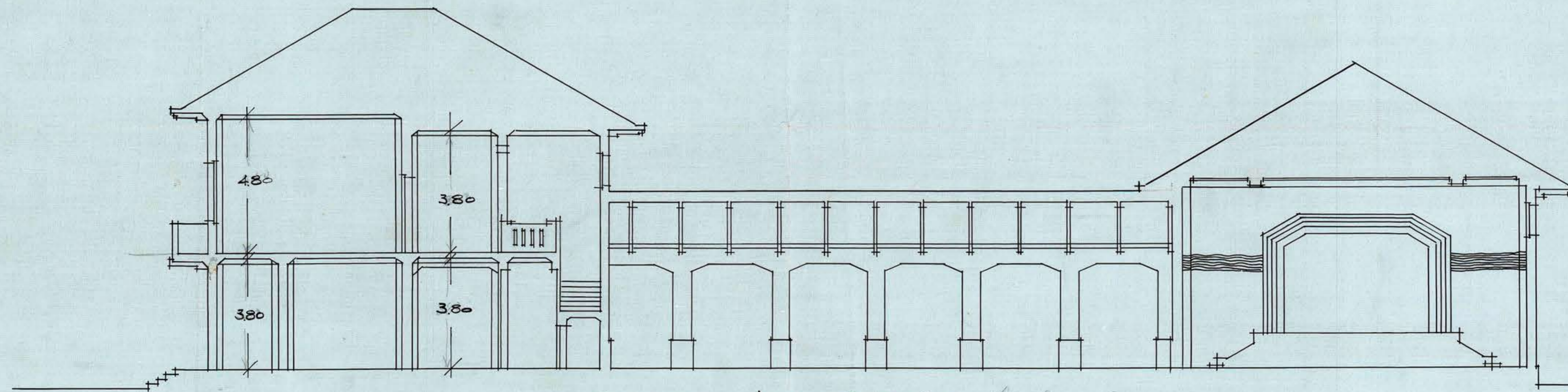
SECCION LONGITUDINAL
