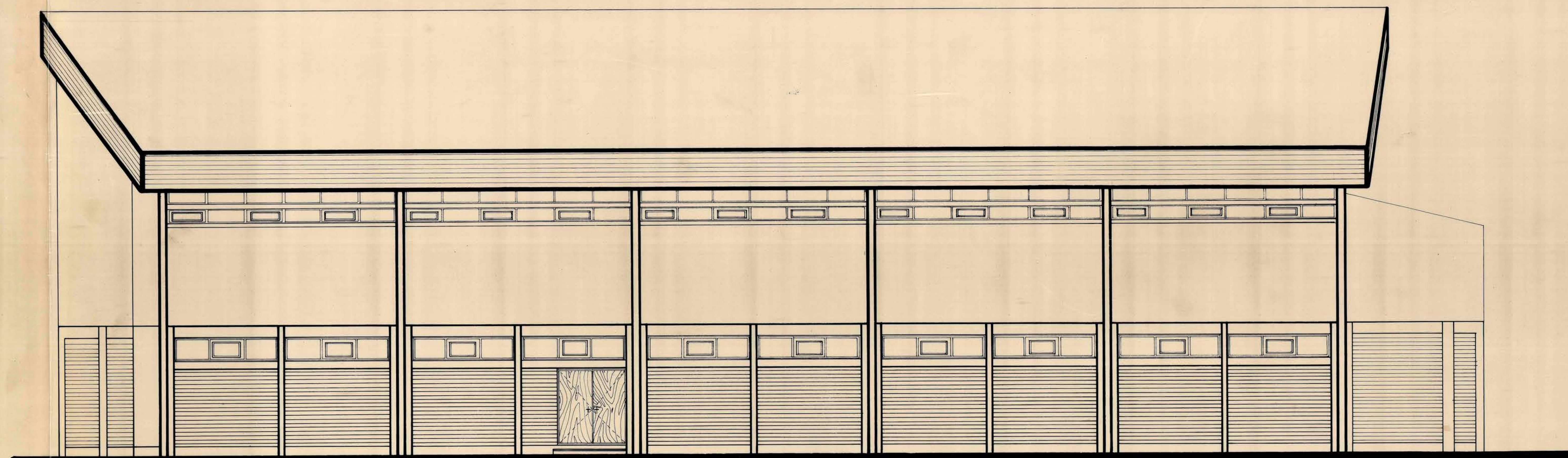
ELEVACION SUR Escala 1:50
