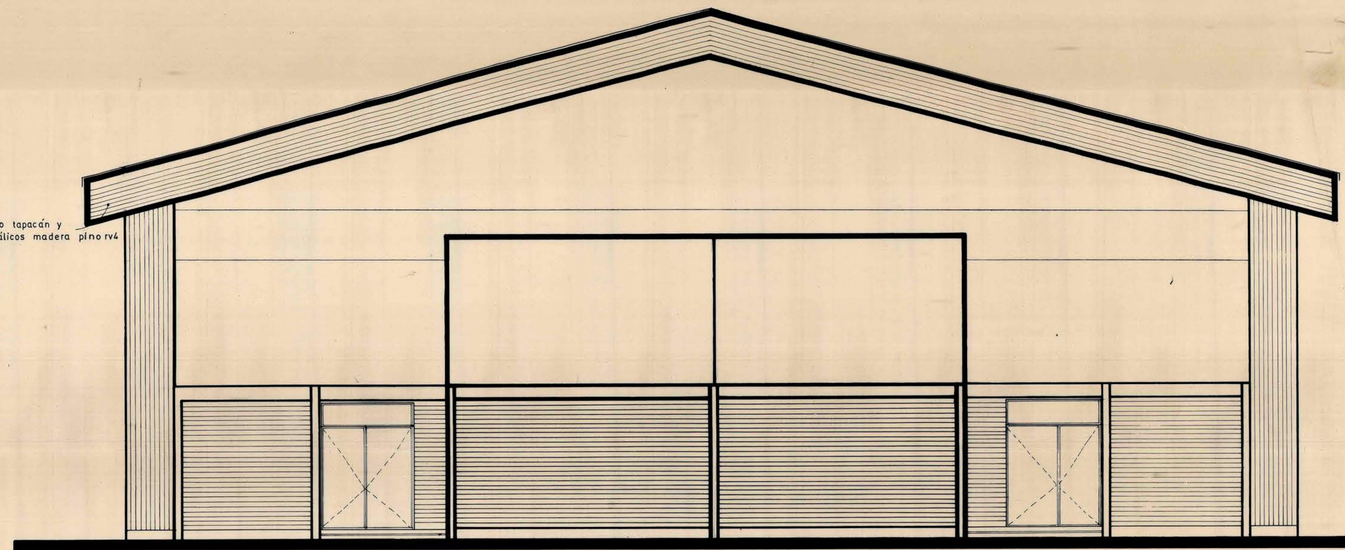
ELEVACION POSTERIOR Escala 1:50
