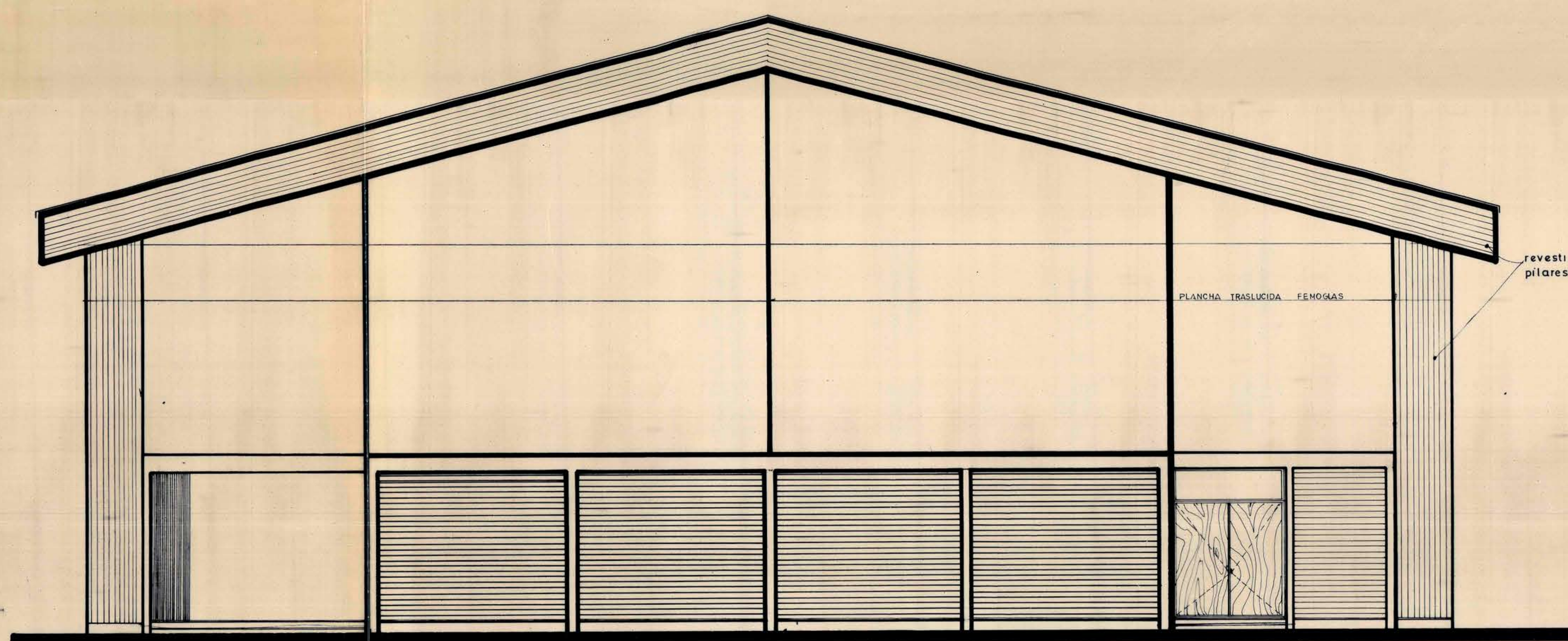
ELEVACION PRINCIPAL Escala 1:50
