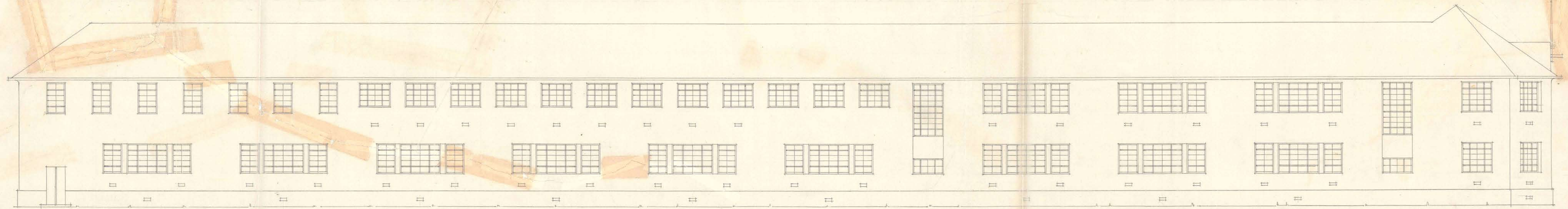
FACHADA A LA CALLE QUILLOTA.
