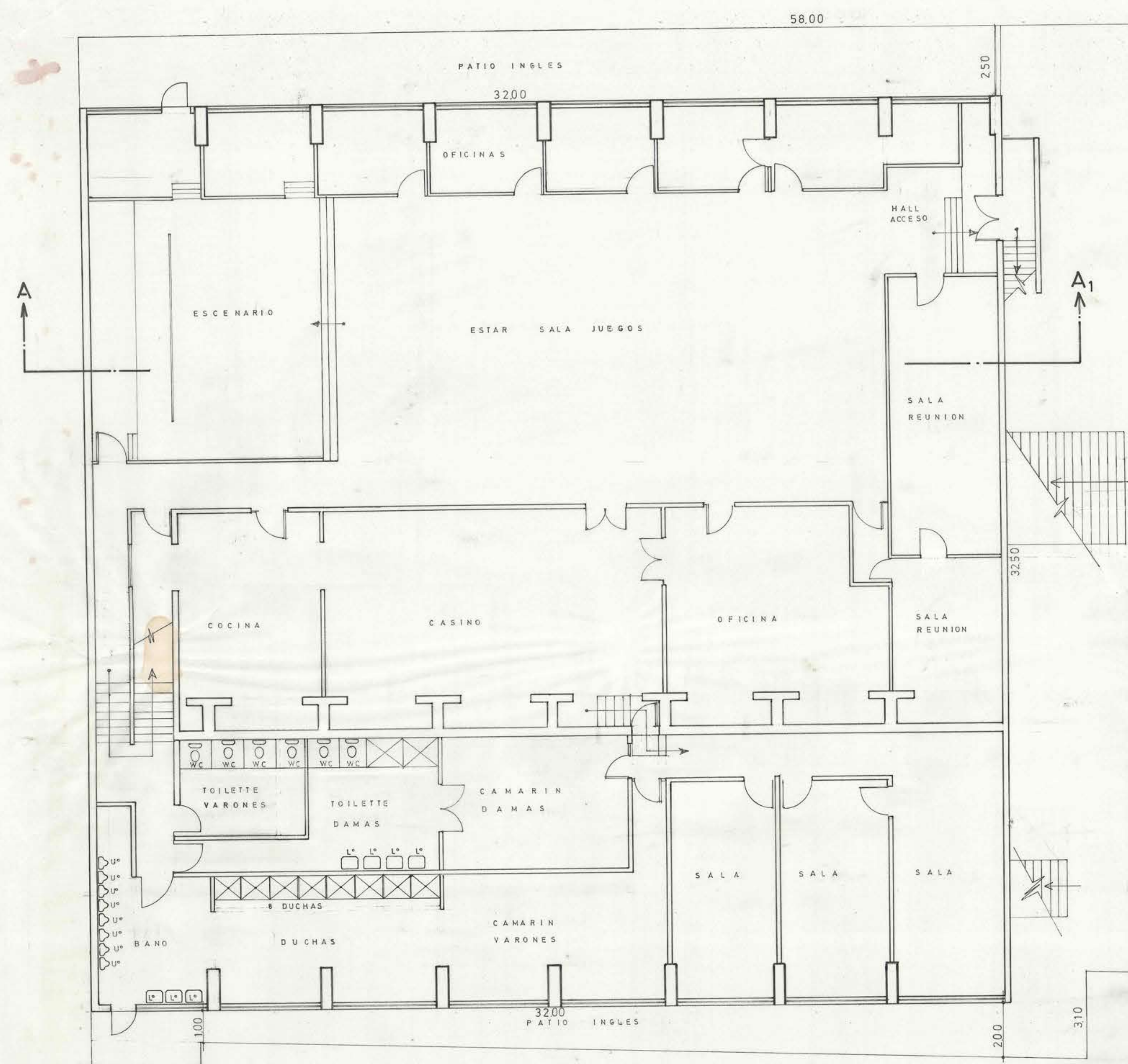
PLANTA A NIVEL INFERIOR
