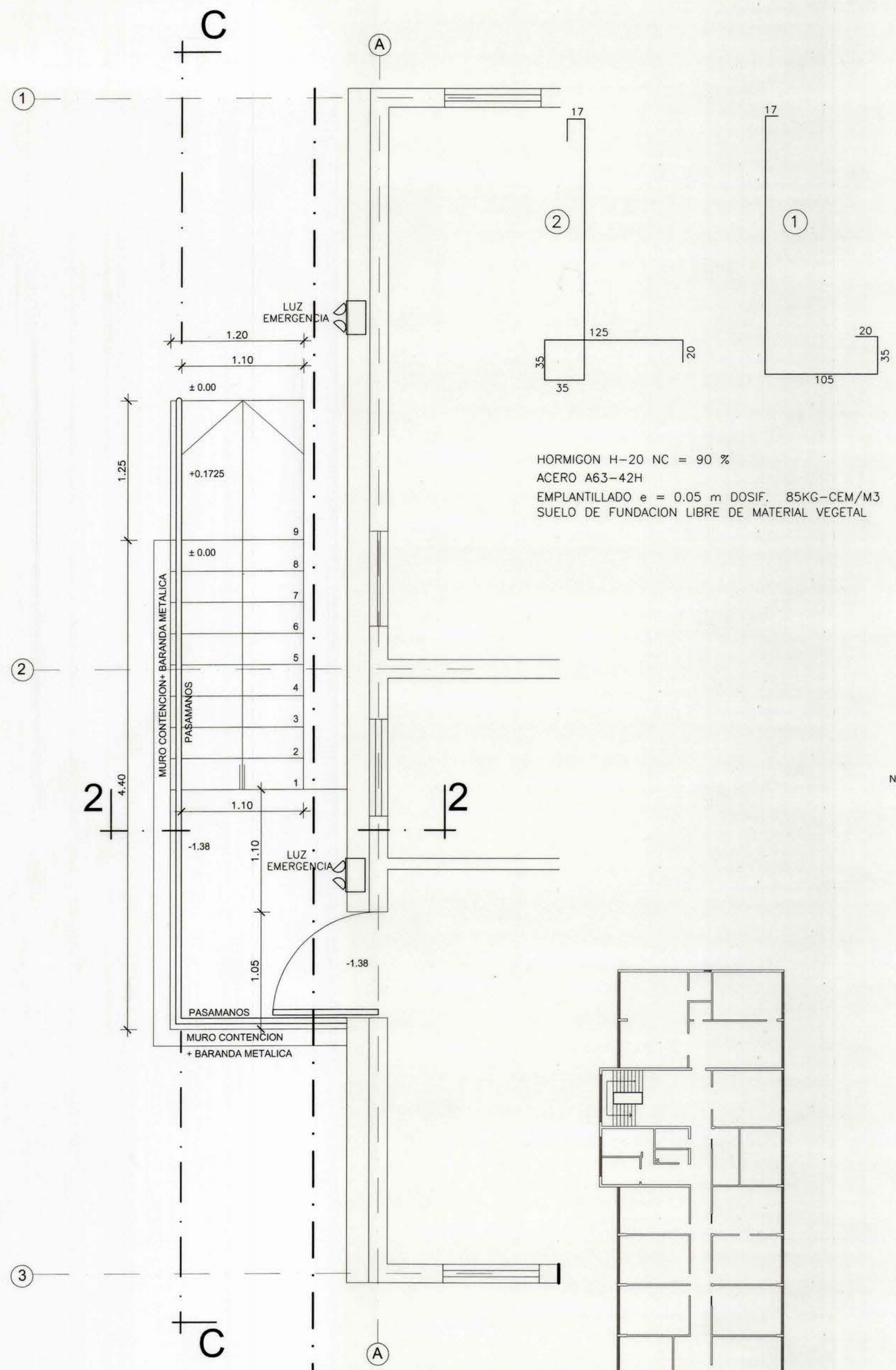
PLANTA ESCALA ZOCALO ESCALA 1 : 25
