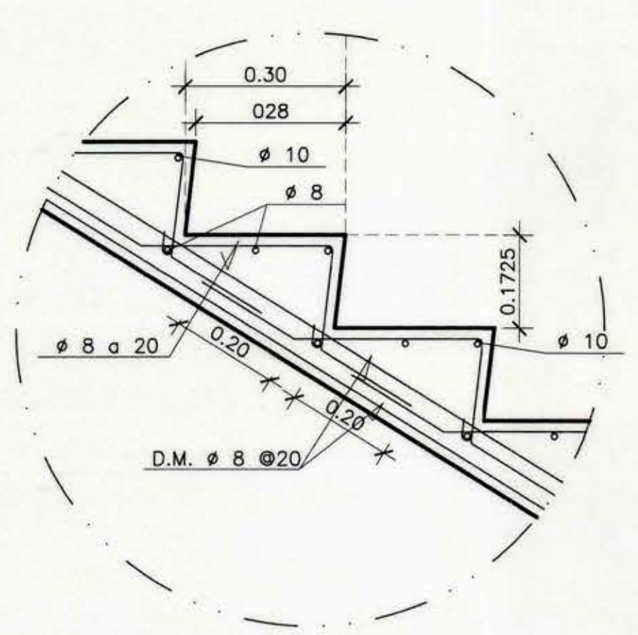
DETALLE ESCALA ZOCALO ESCALA 1 : 10
