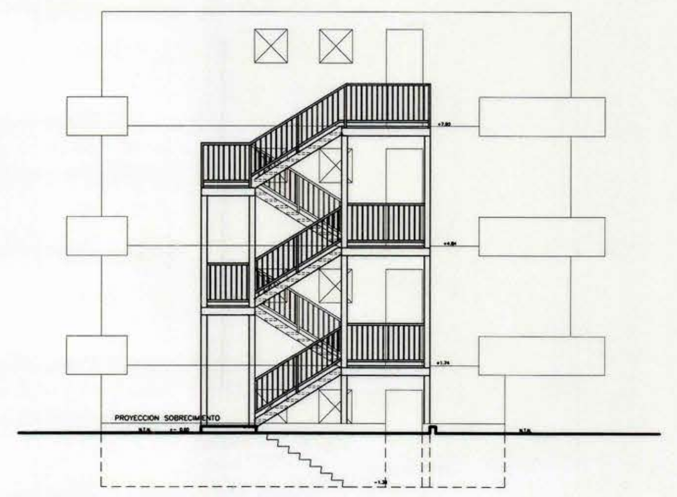
ELEVACION SUR ESCALA 1 ESCALA 1 : 100
