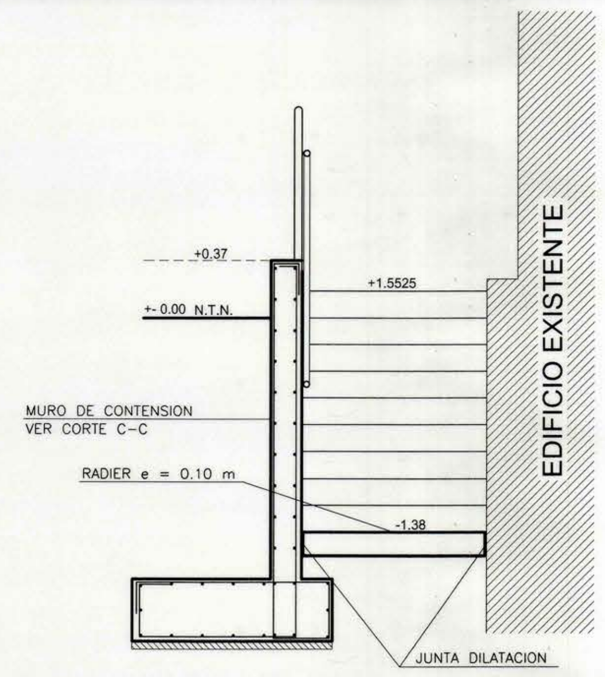
CORTE 2-2 ESCALA ZOCALO ESCALA 1 : 25
