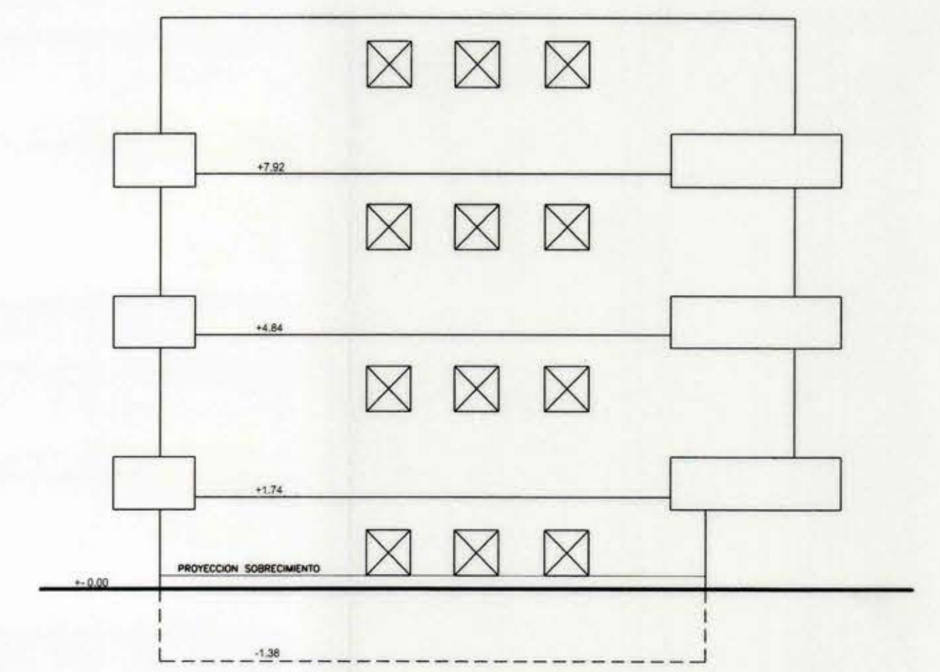
ELEVACION EXISTENTE ESCALA 1 : 100
