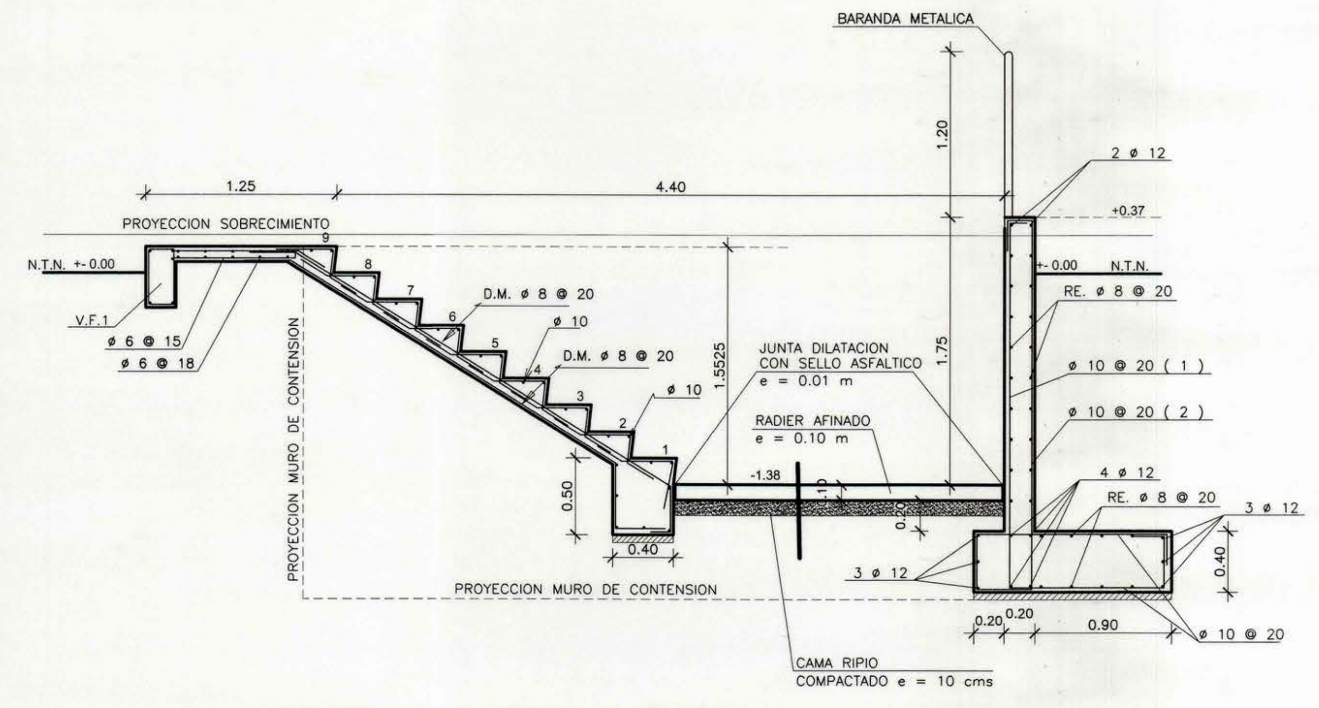
CORTE C-C ESCALA ZOCALO ESCALA 1 : 25
