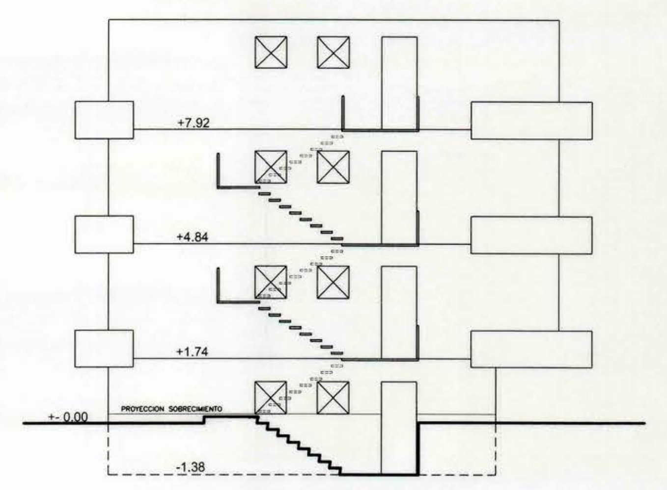
ESQUEMA ELEVACION A-A ESCALA 1 ESCALA 1 : 100
