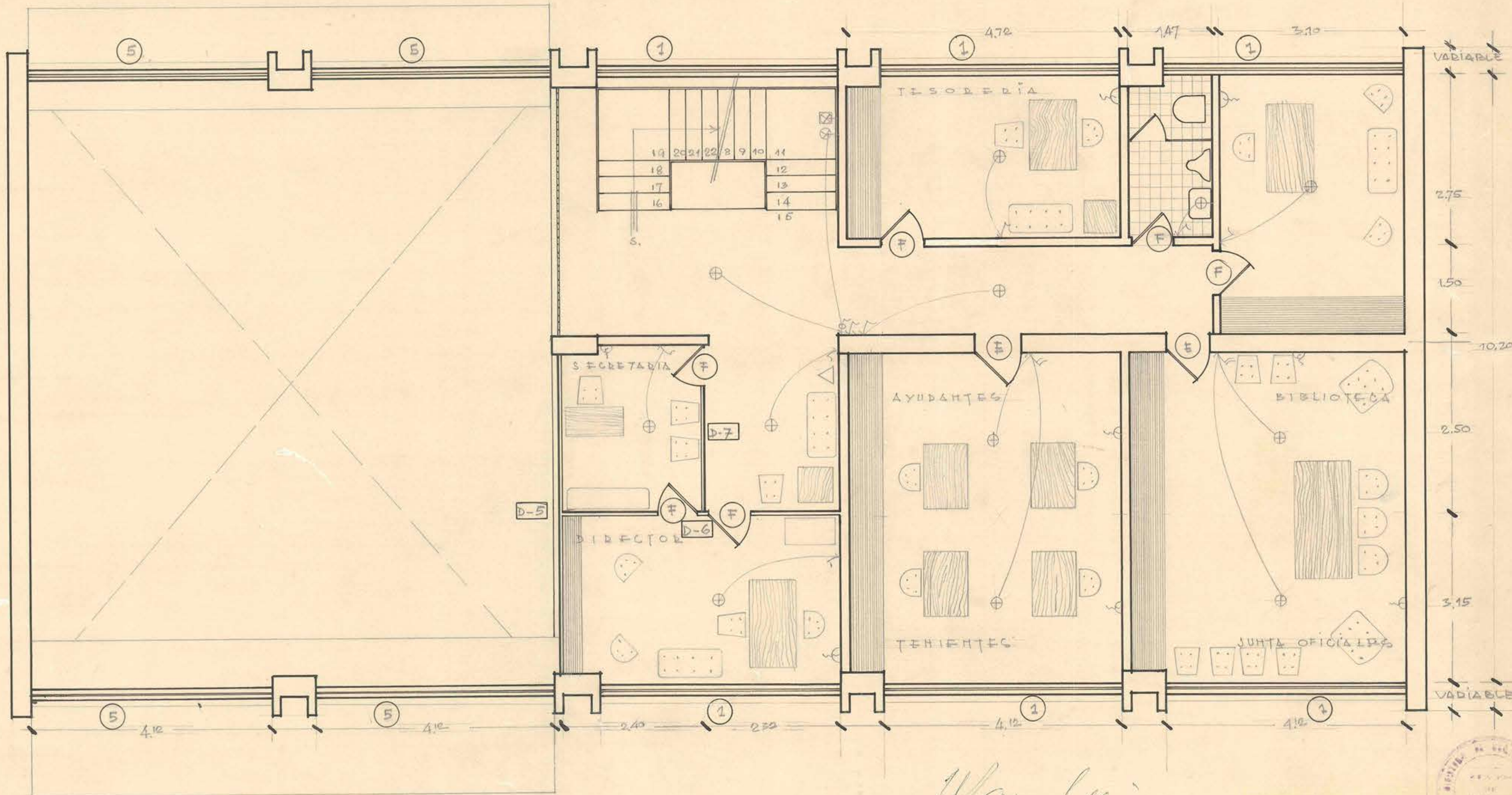
PLANTA 2º PISO 2 de Guayaquil
