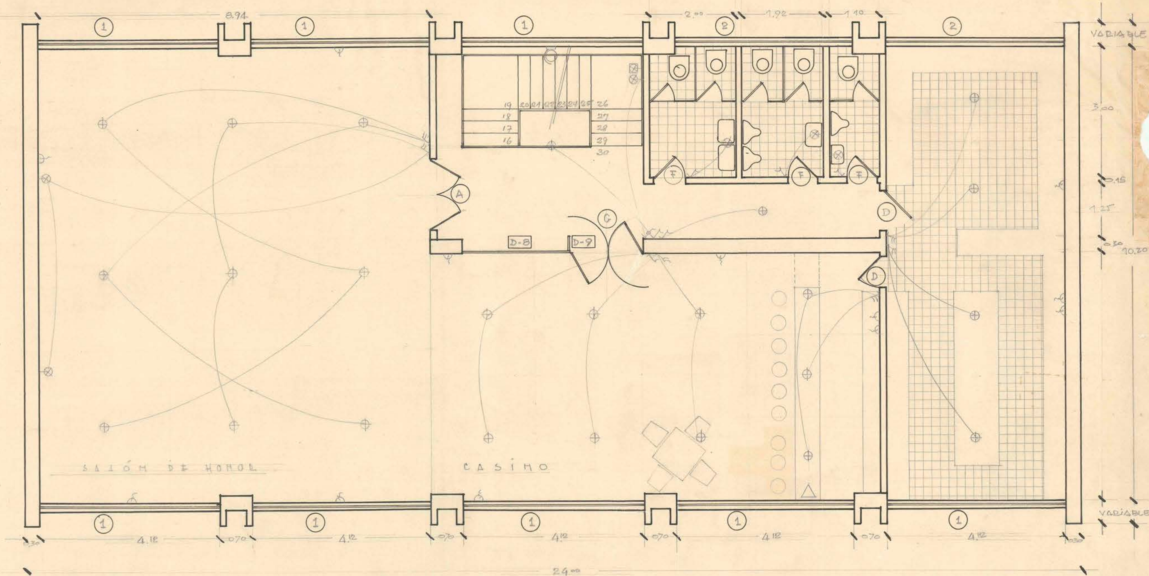
PLANTA 3º PISO
