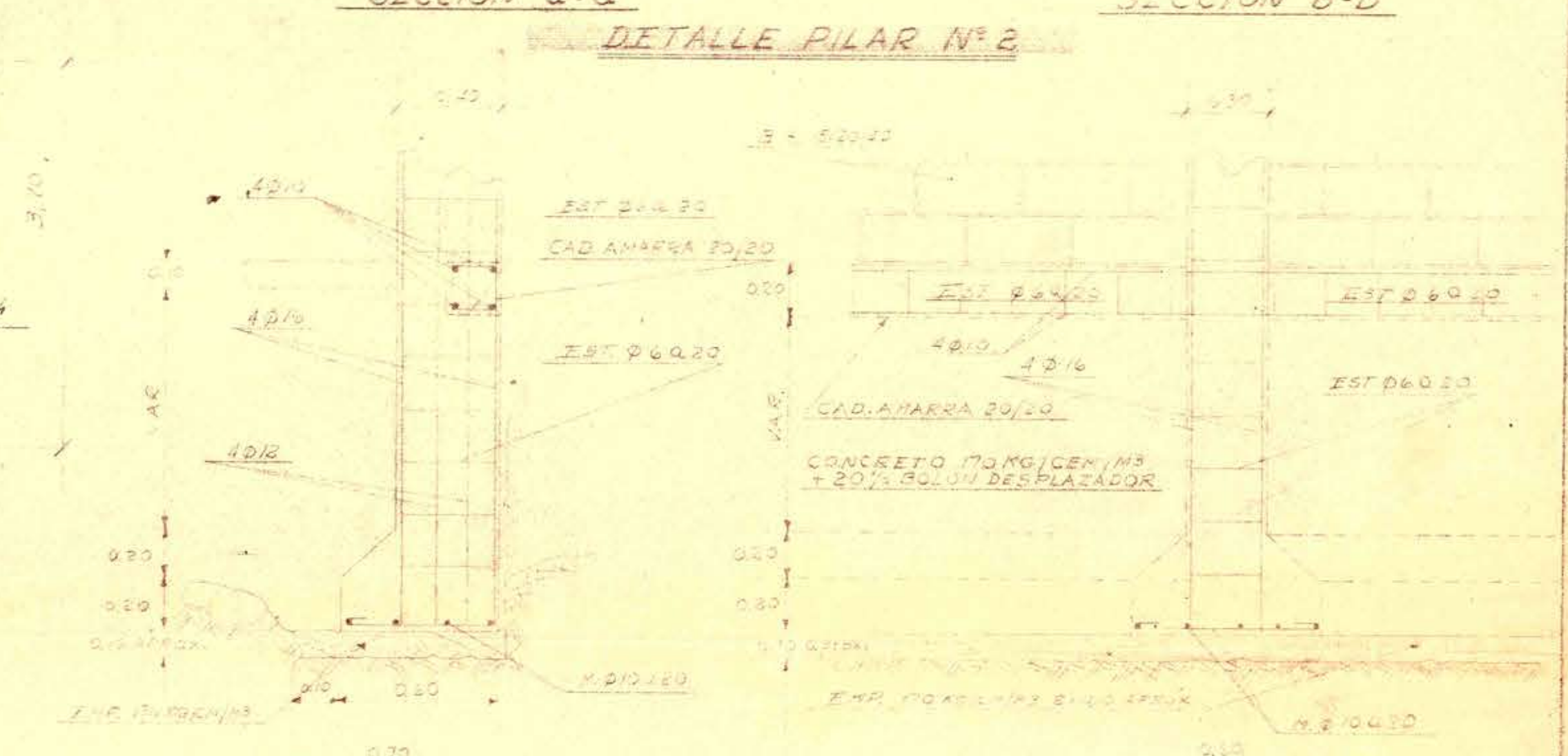
SECCION C-C
