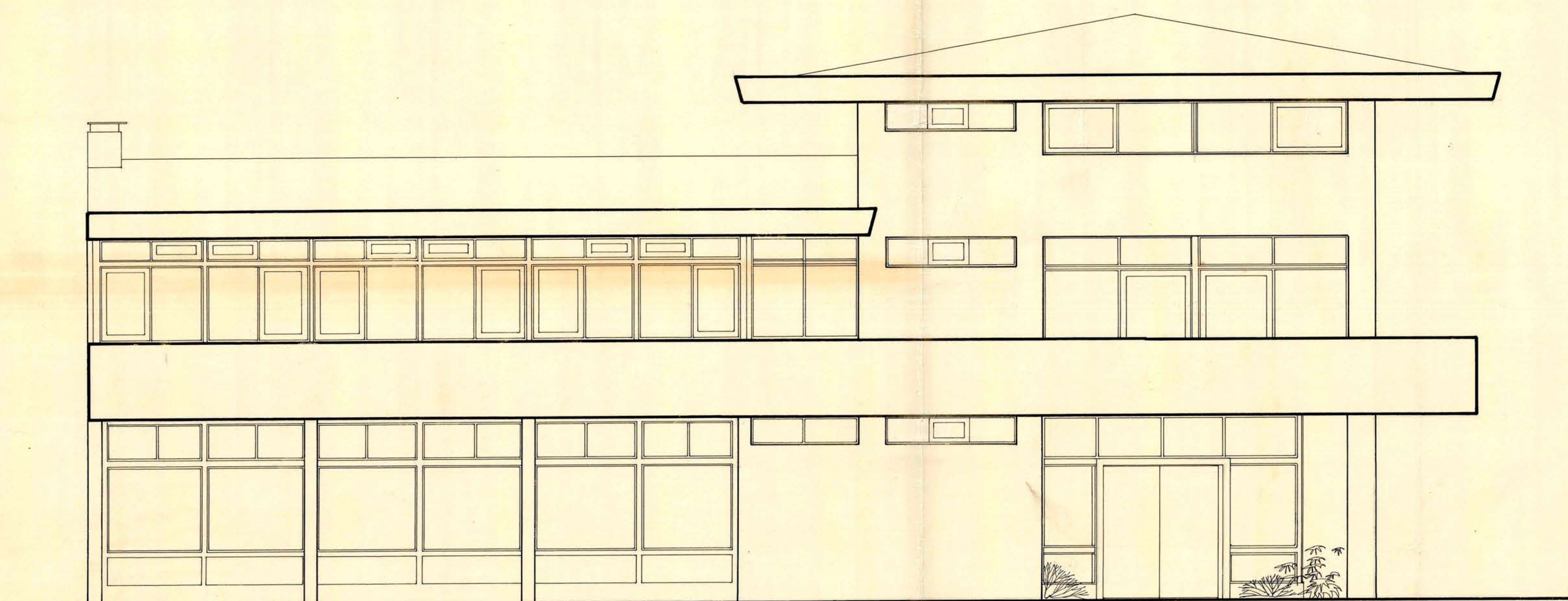
ELEVACION PONIENTE
