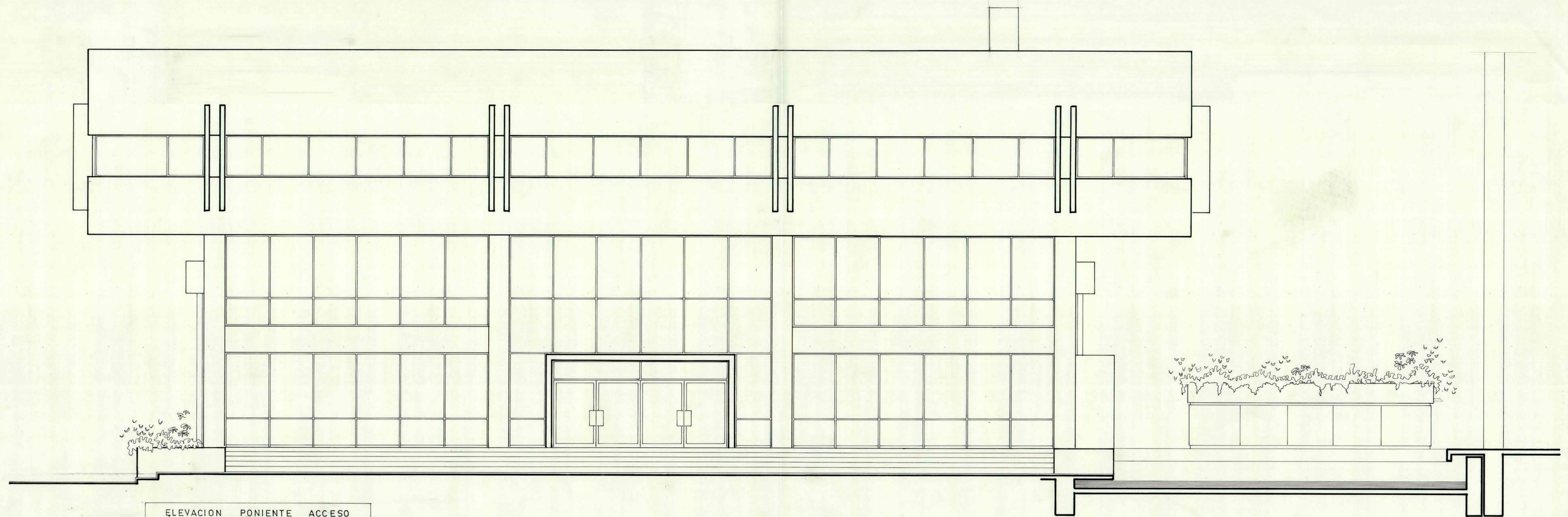
ELEVACION PONIENTE ACCESO
