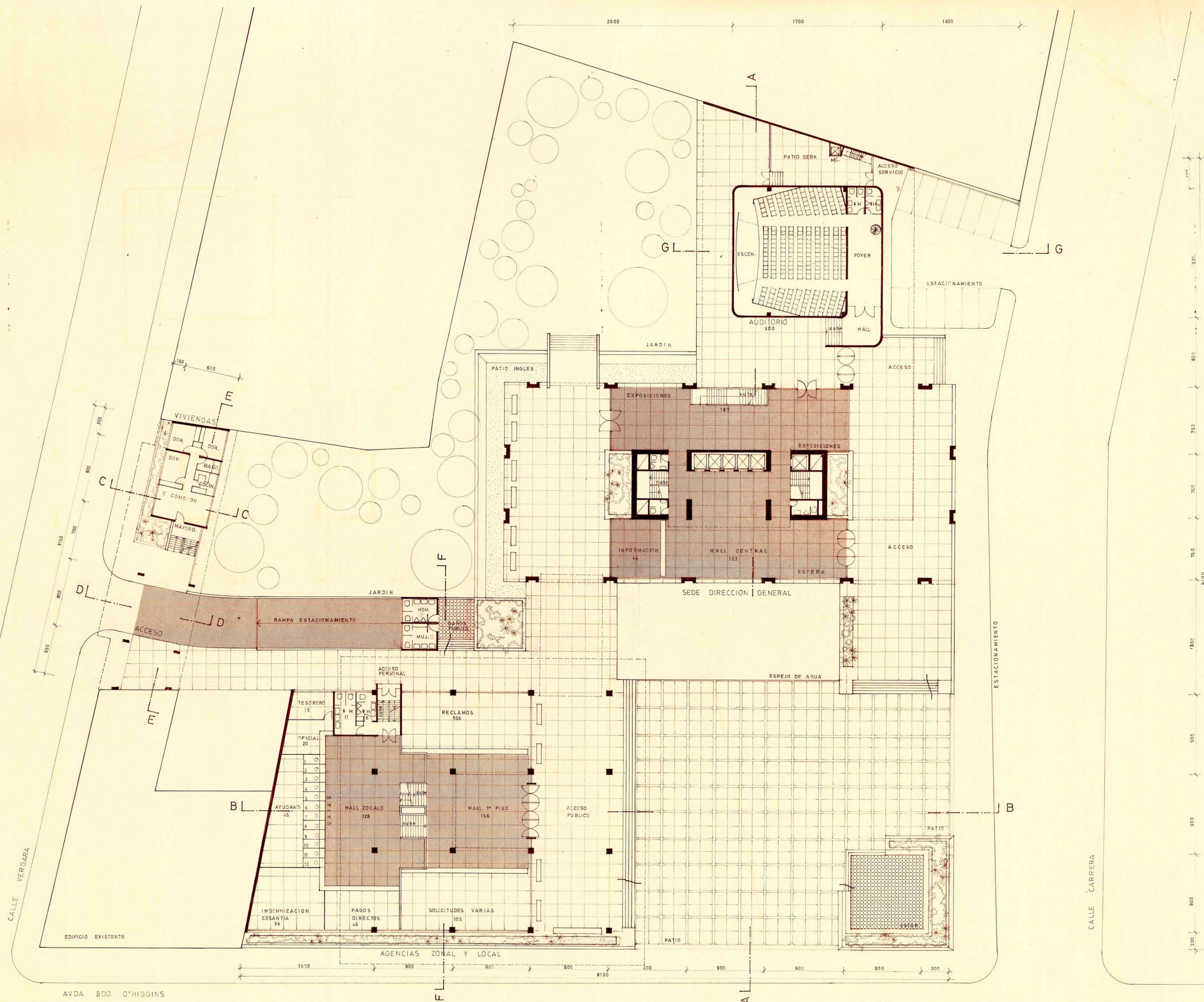
PLANTA GENERAL 1º PISO ESC 1/200
