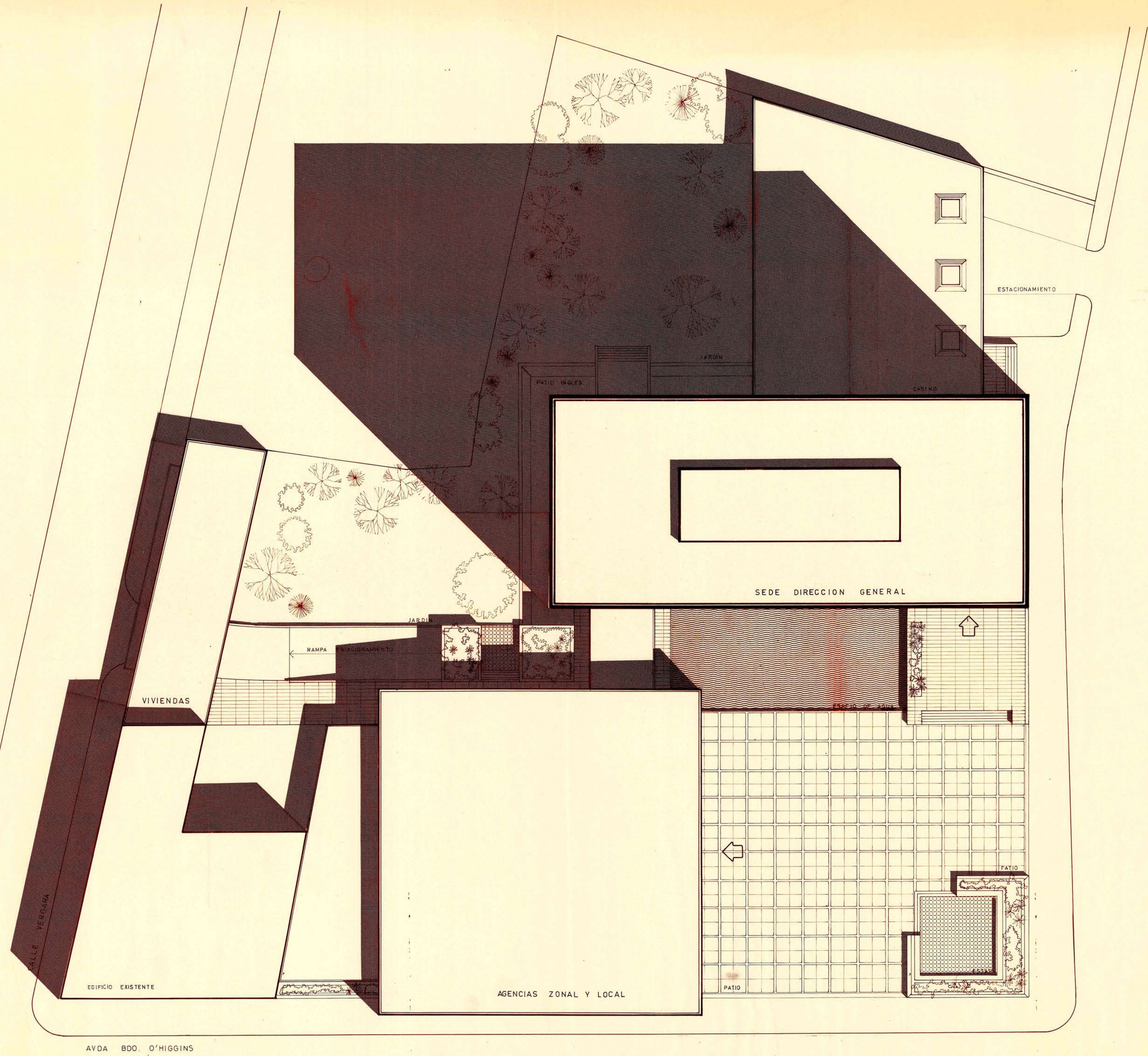
PLANTA DE CONJUNTO ESC 1/200
