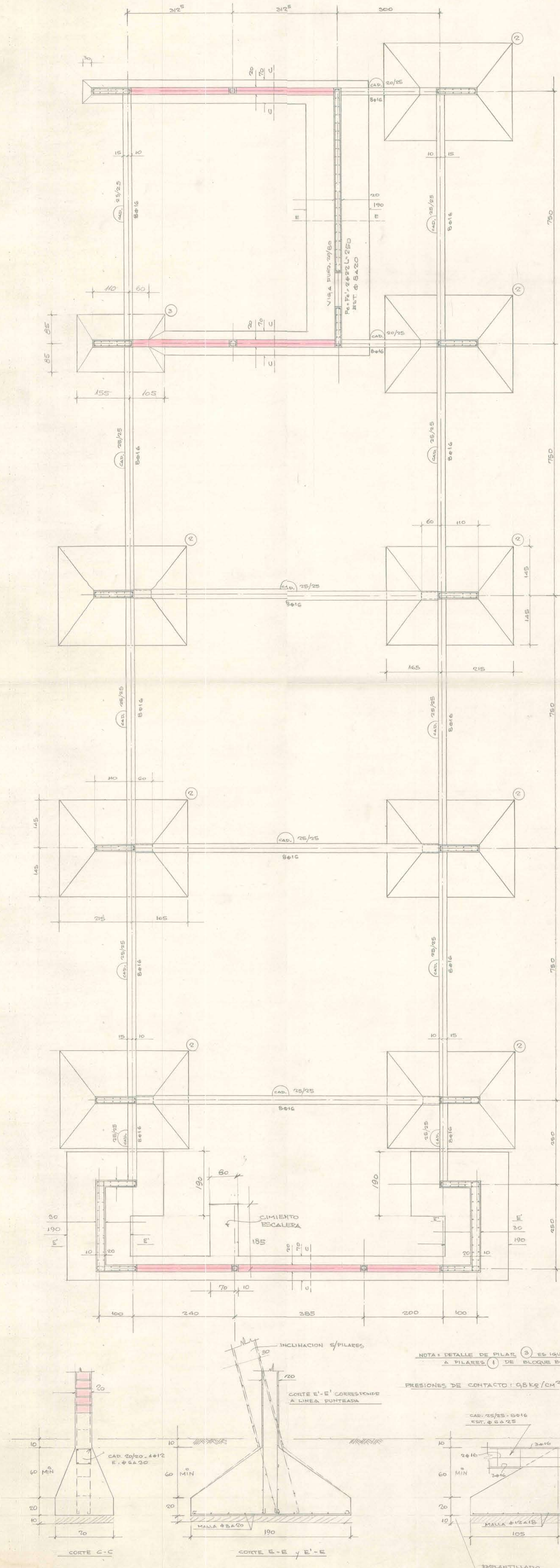
PLANTA DE FUNDACIONES
